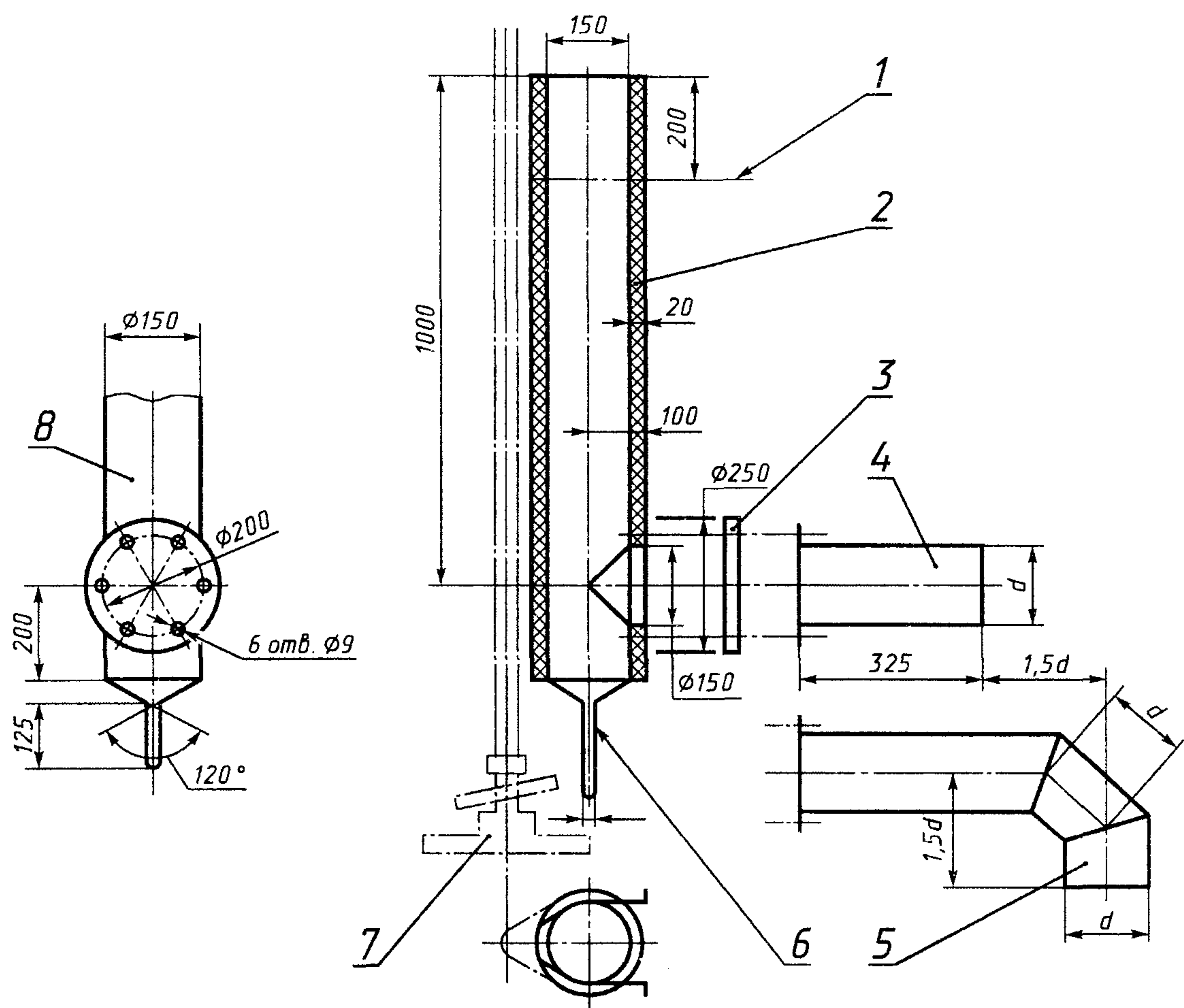
1 — плоскость измерения (пробоотборник и термопара); 2 — теплоизоляция (стекловолотно плотностью 64 кг/м 3 ); 3 — прокладка; 4, 5 — соединительные трубы из нержавеющей стали; 6 — трубка внутренним диаметром 8 мм и толщиной стенки 1 мм; 7 — опорная стойка (высота регулируемая); 8 — труба дымохода из нержавеющей стали
