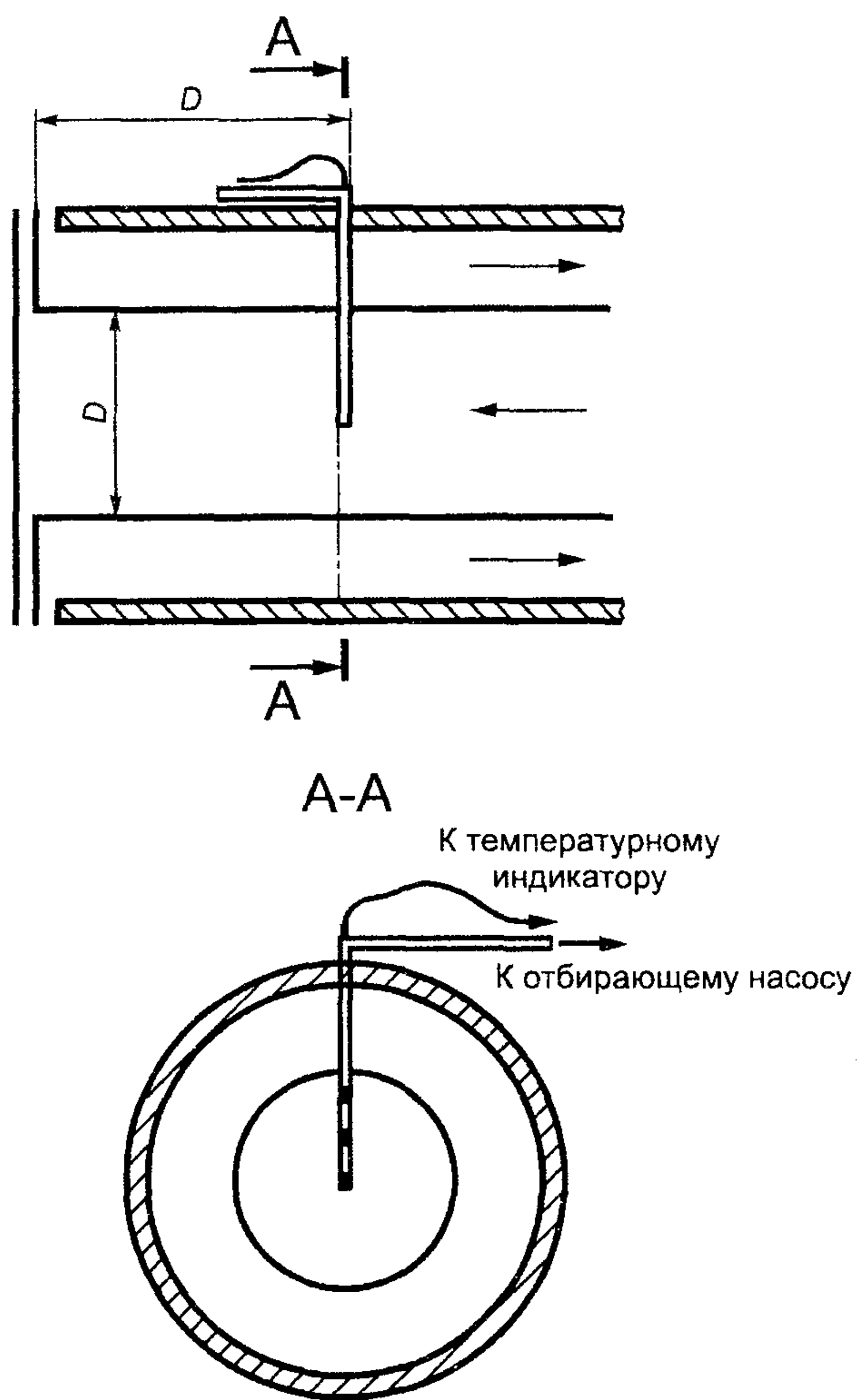
Рисунок 8 — Точка отбора проб для аппаратов типа С
