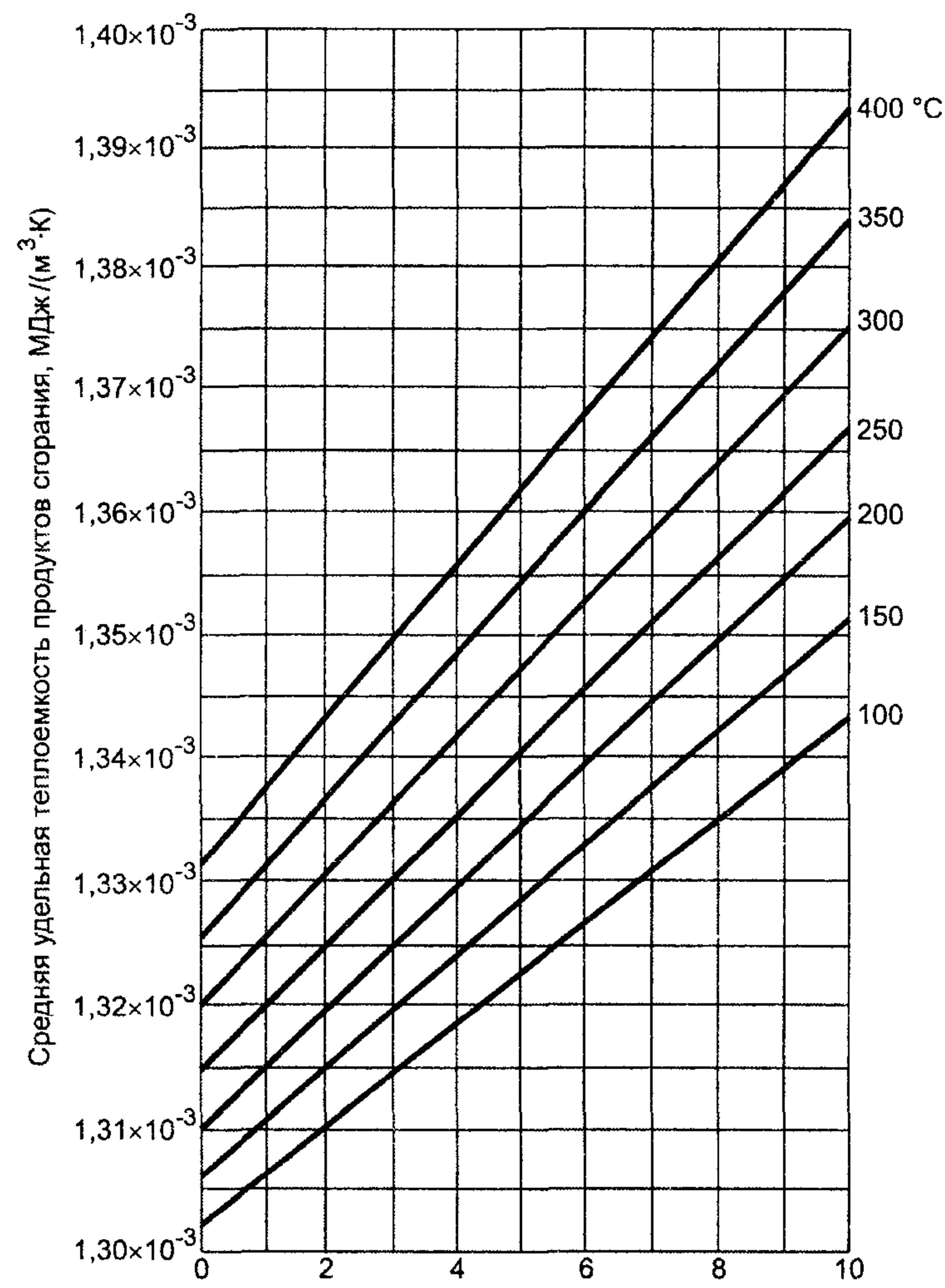
Рисунок 11 — Средняя удельная теплоемкость продуктов сгорания
