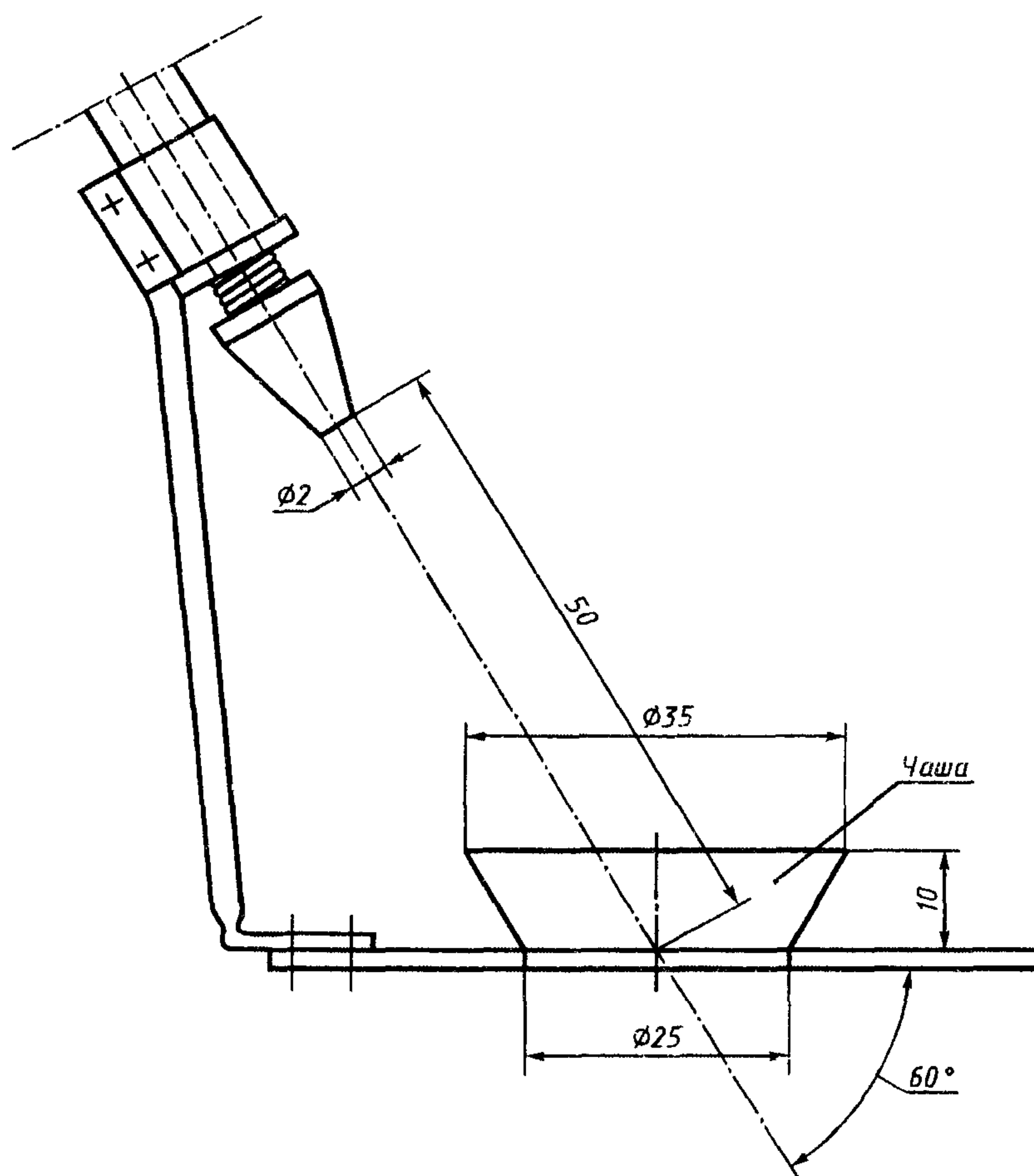
Рисунок 101 — Аппарат для разбрызгивания
