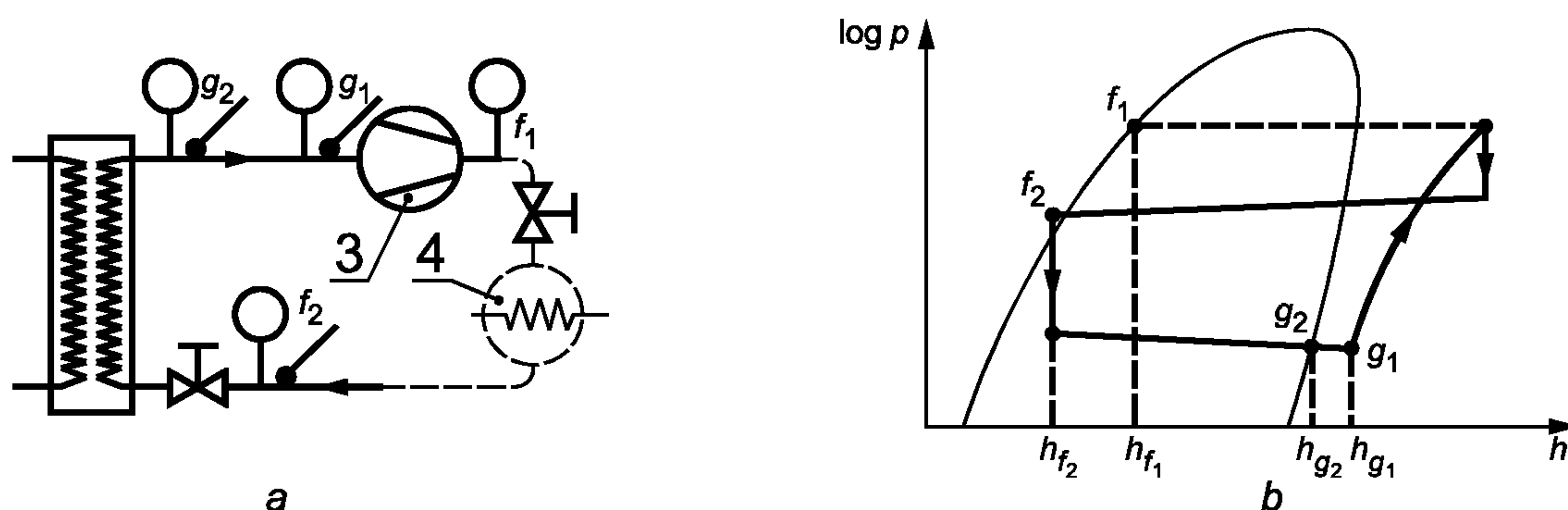
a — схема цикла; b — диаграмма log p—h
