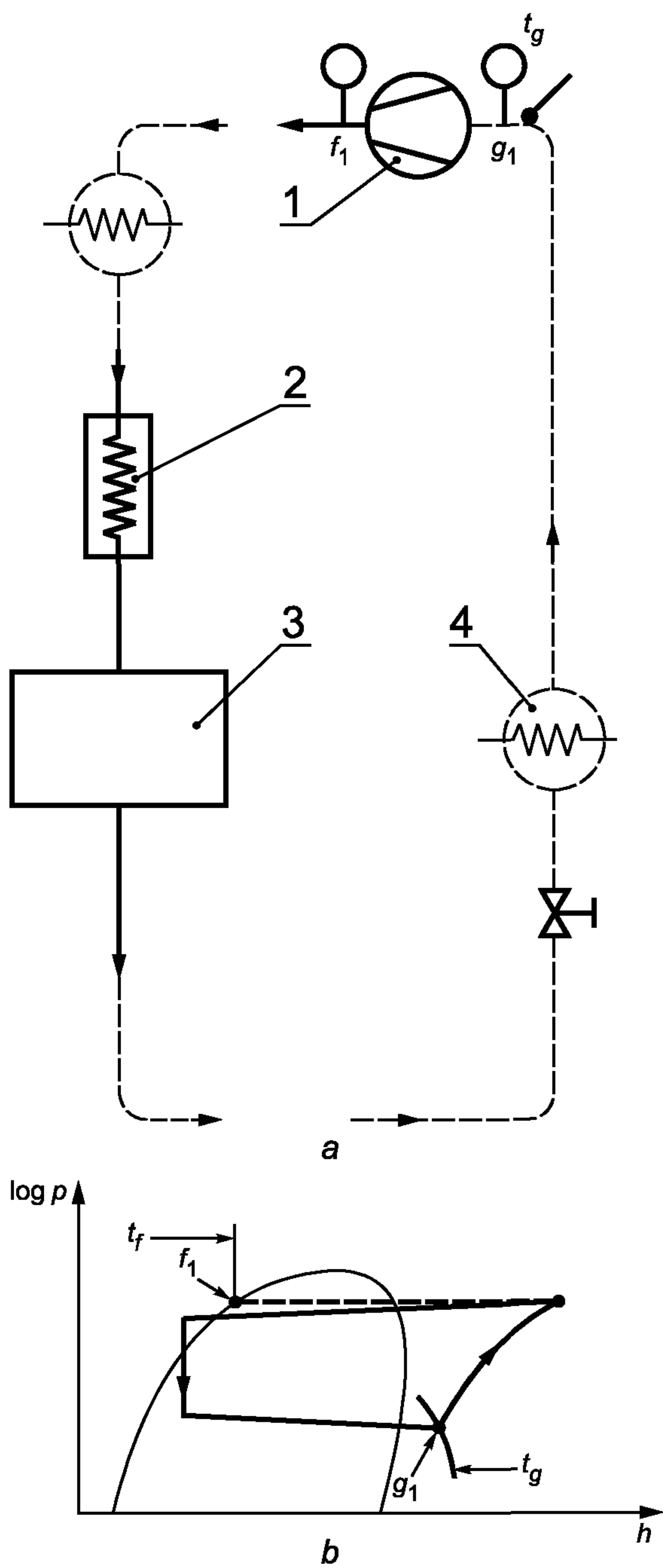
a — схема цикла; b — диаграмма \log p — h 1 — компрессор; 2 — переохладитель; 3 — расходомер; 4 — испаритель
