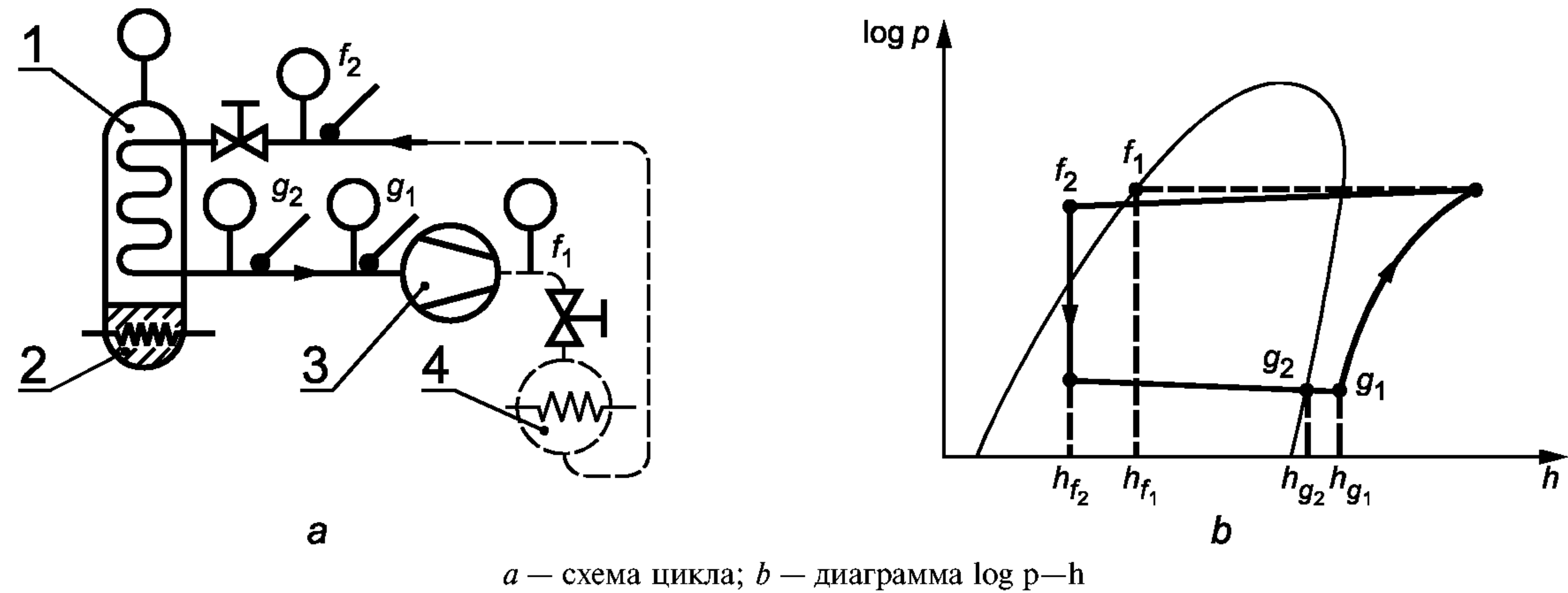
1 — калориметр; 2 — нагреватель; 3 — компрессор; 4 — конденсатор
