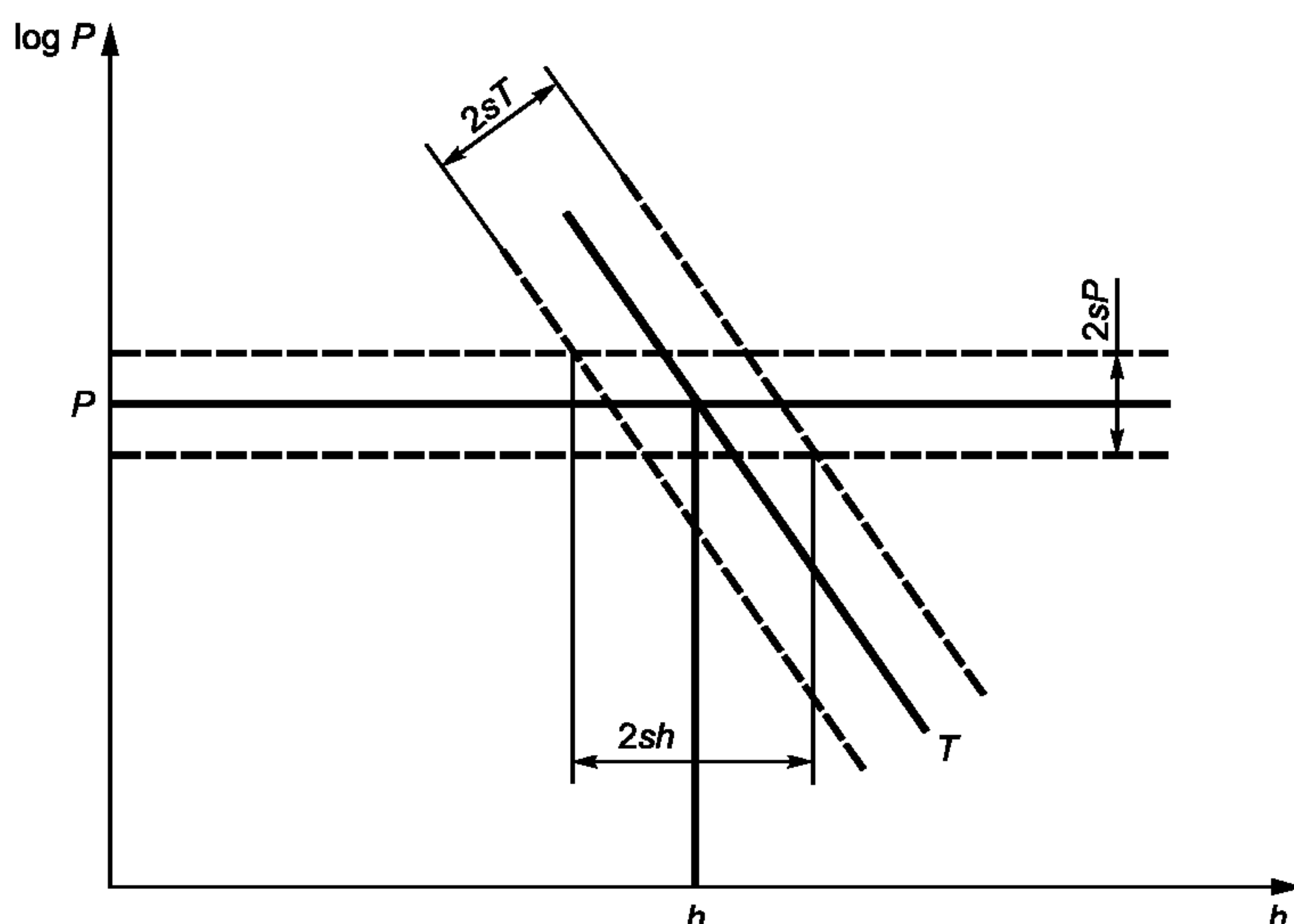
Рисунок В1 — Диаграмма \log p-h
