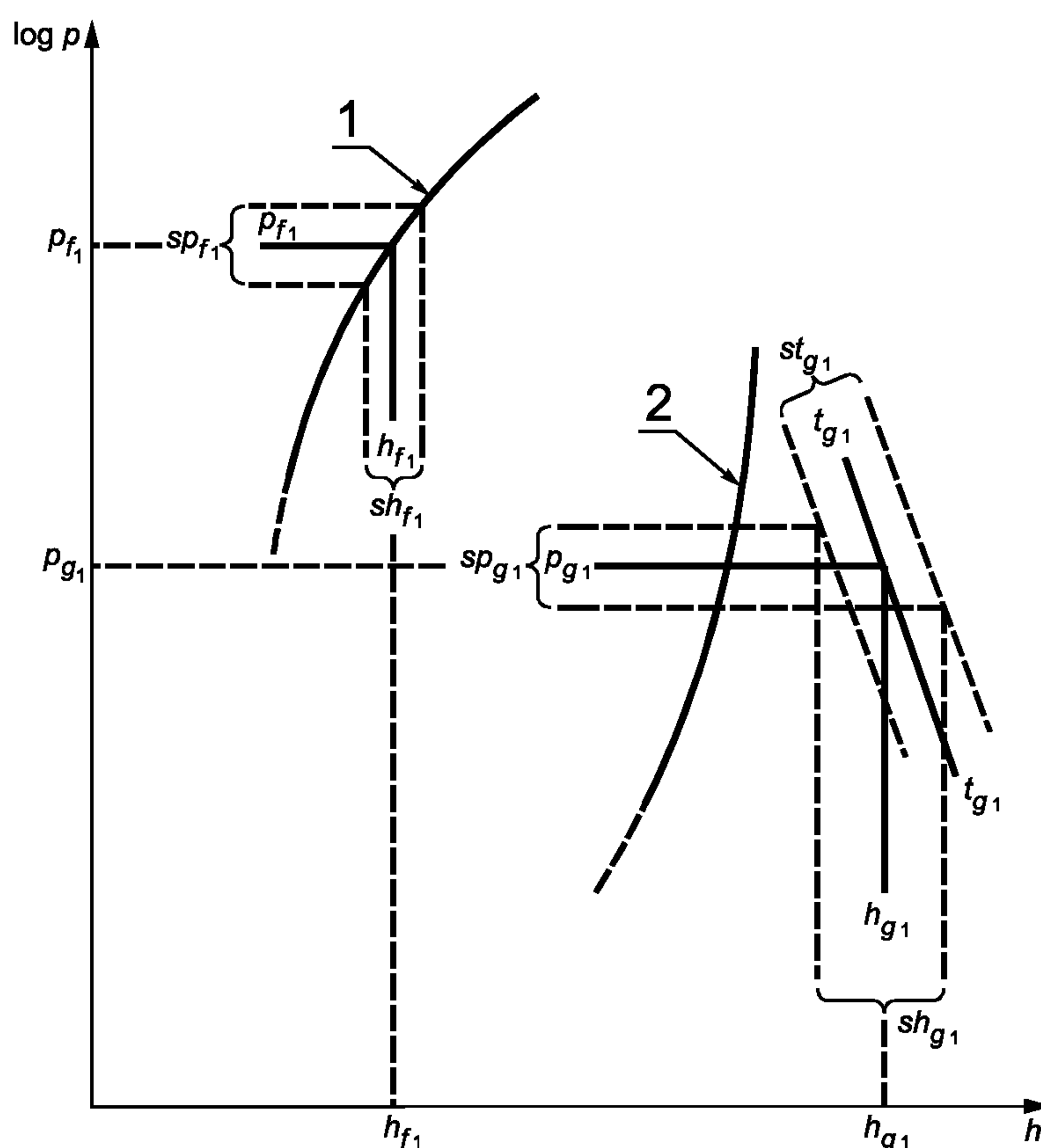
1 — кривая насыщения жидкости; 2 — кривая насыщения пара
