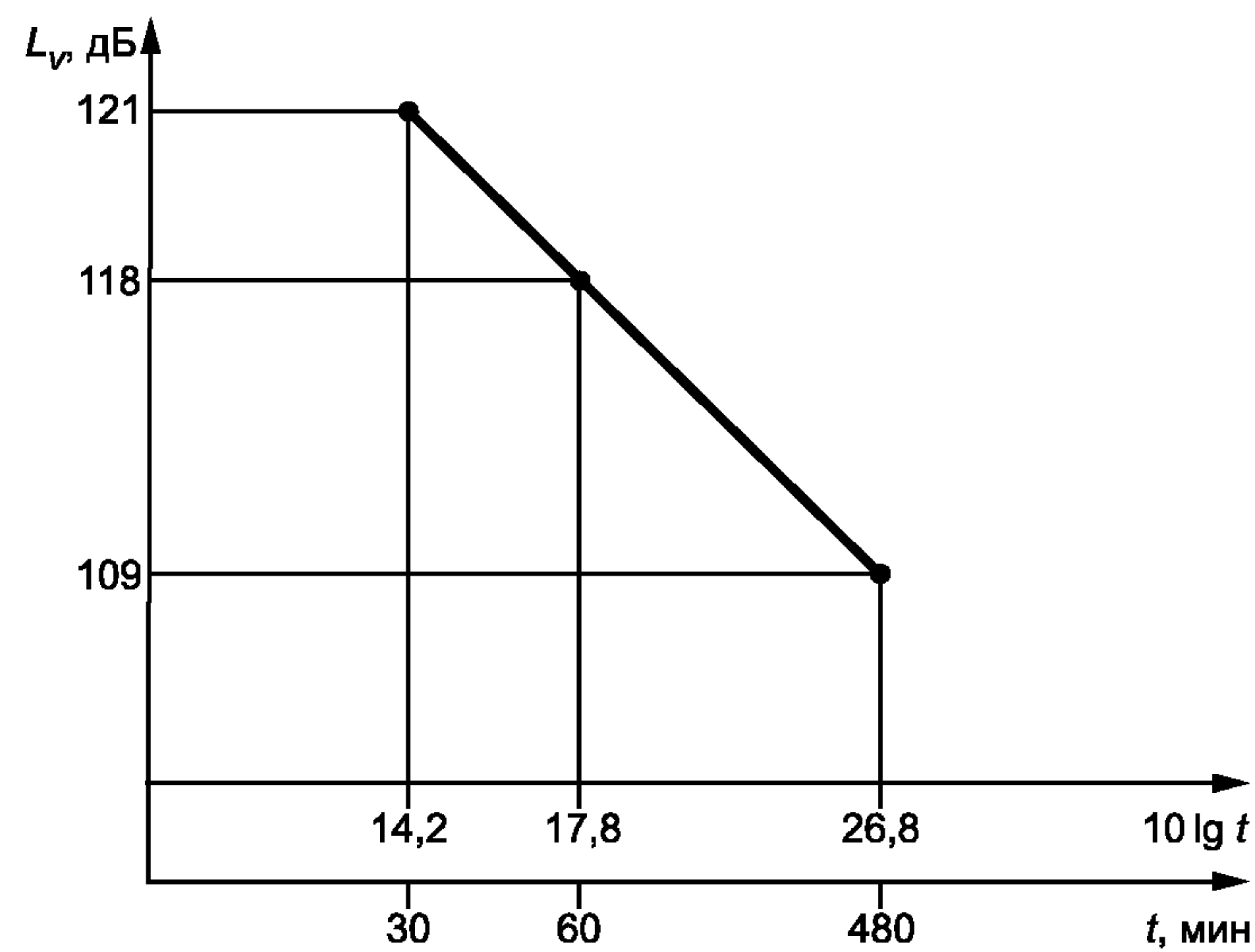
График зависимости предельного уровня вибрации L_v от времени пребывания обслуживающего персонала на рабочем месте, t
