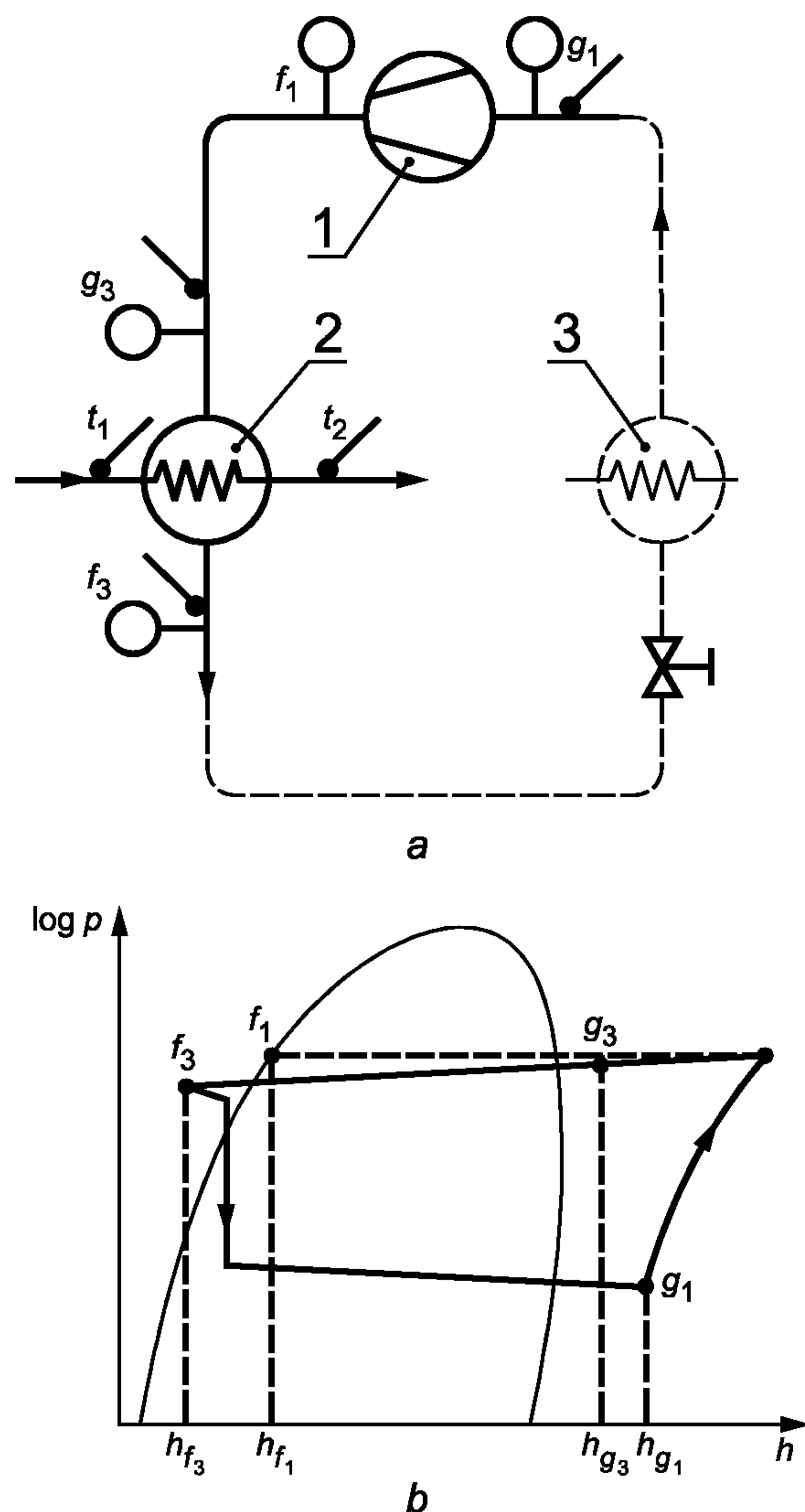
a — схема цикла; b — диаграмма \log p — h 1 — компрессор; 2 — конденсатор; 3 — испаритель
