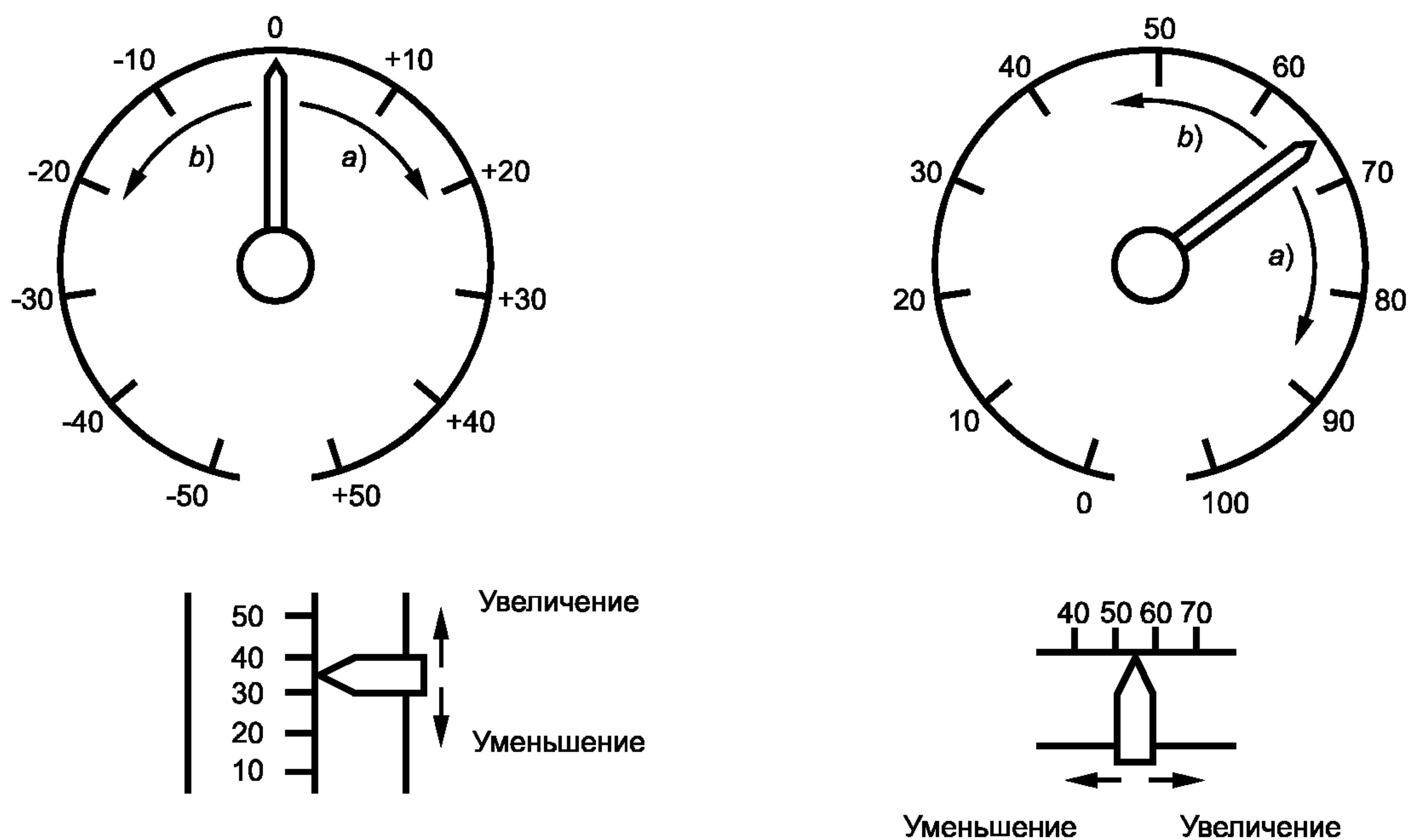
Рисунок 4 — Направления движения стрелок
