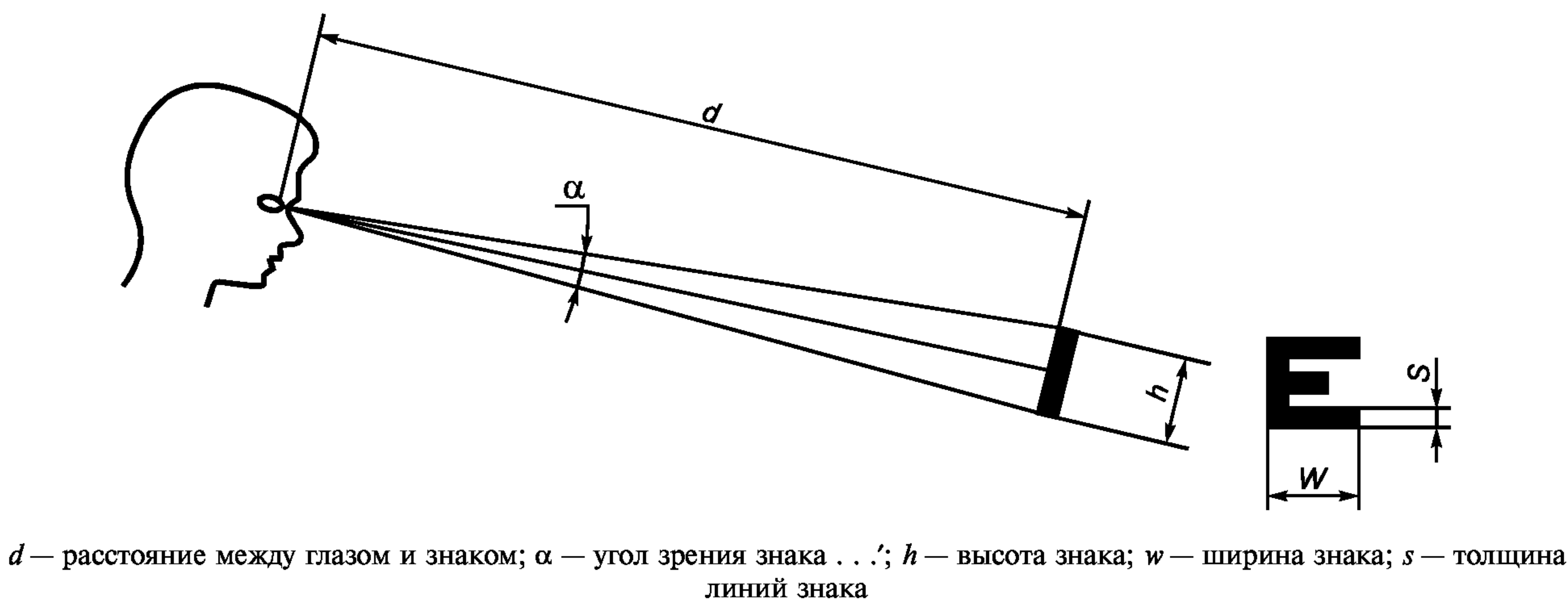
Рисунок 3 — Определение размеров знаков
