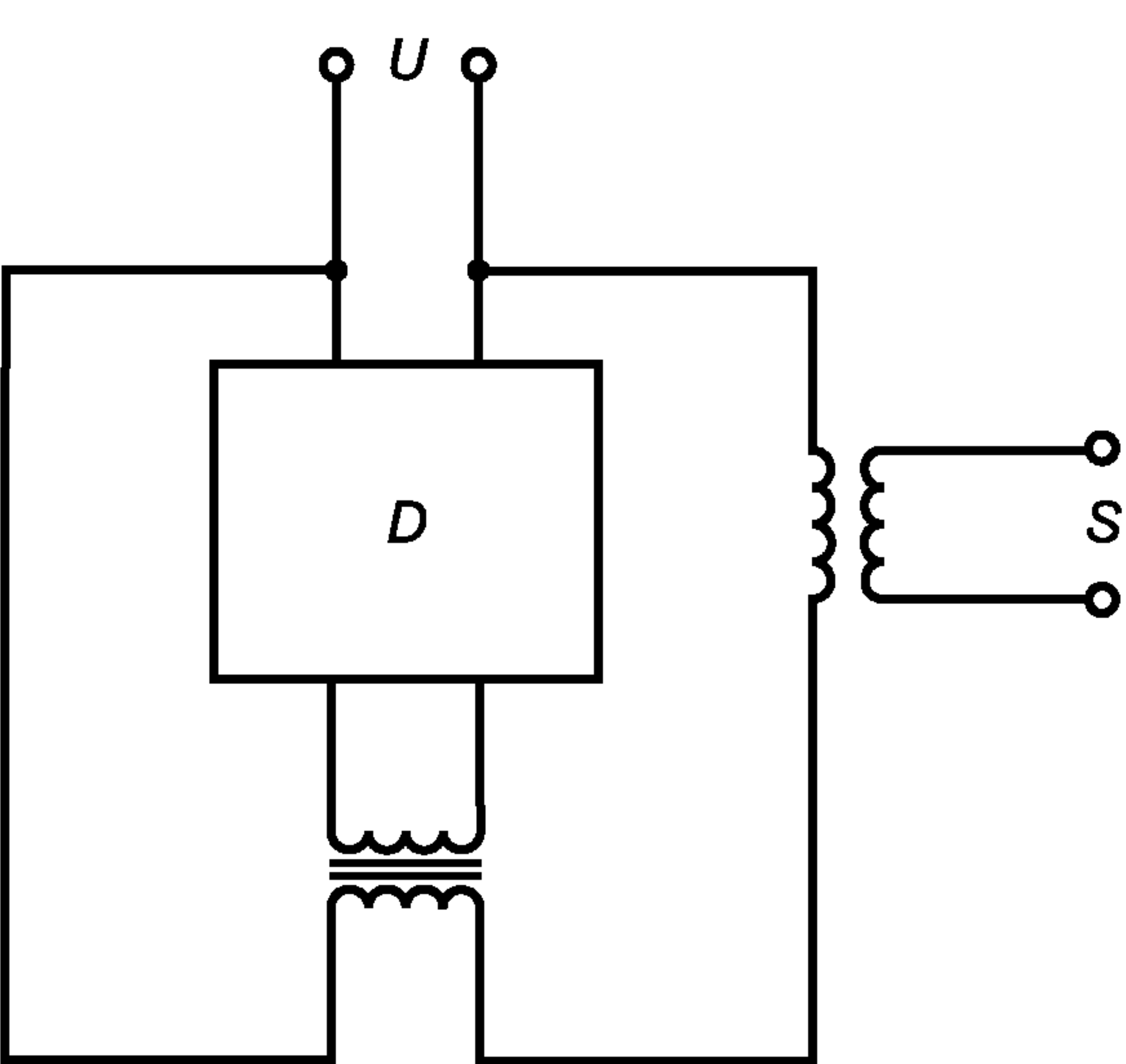
U — источник напряжения 1,1 U_n ; S — источник тока; D — испытуемый АВДТ
