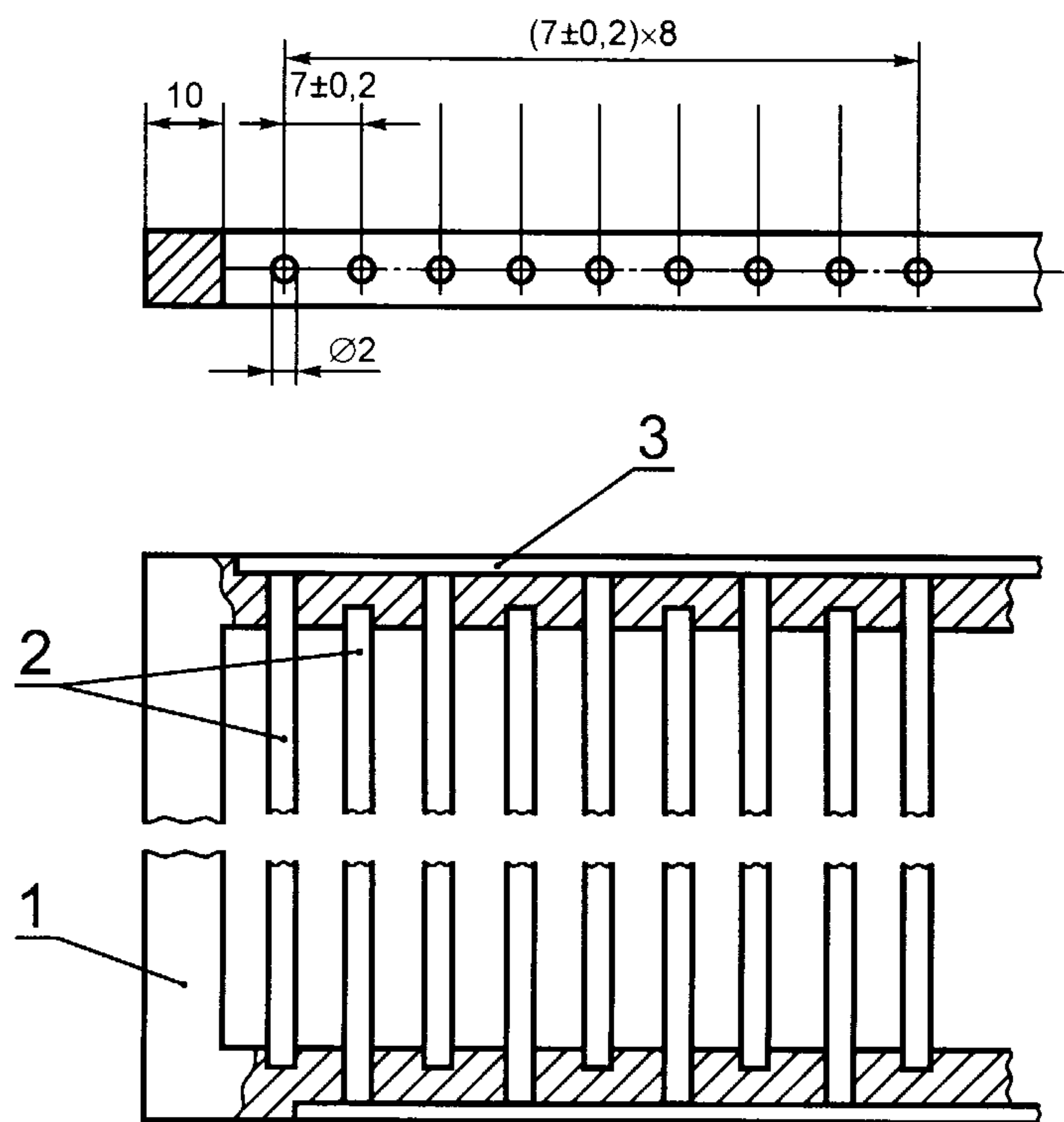
I — рамка из изоляционного материала; 2 — медные проволоки; 3 — металлическое соединение медных проволок
