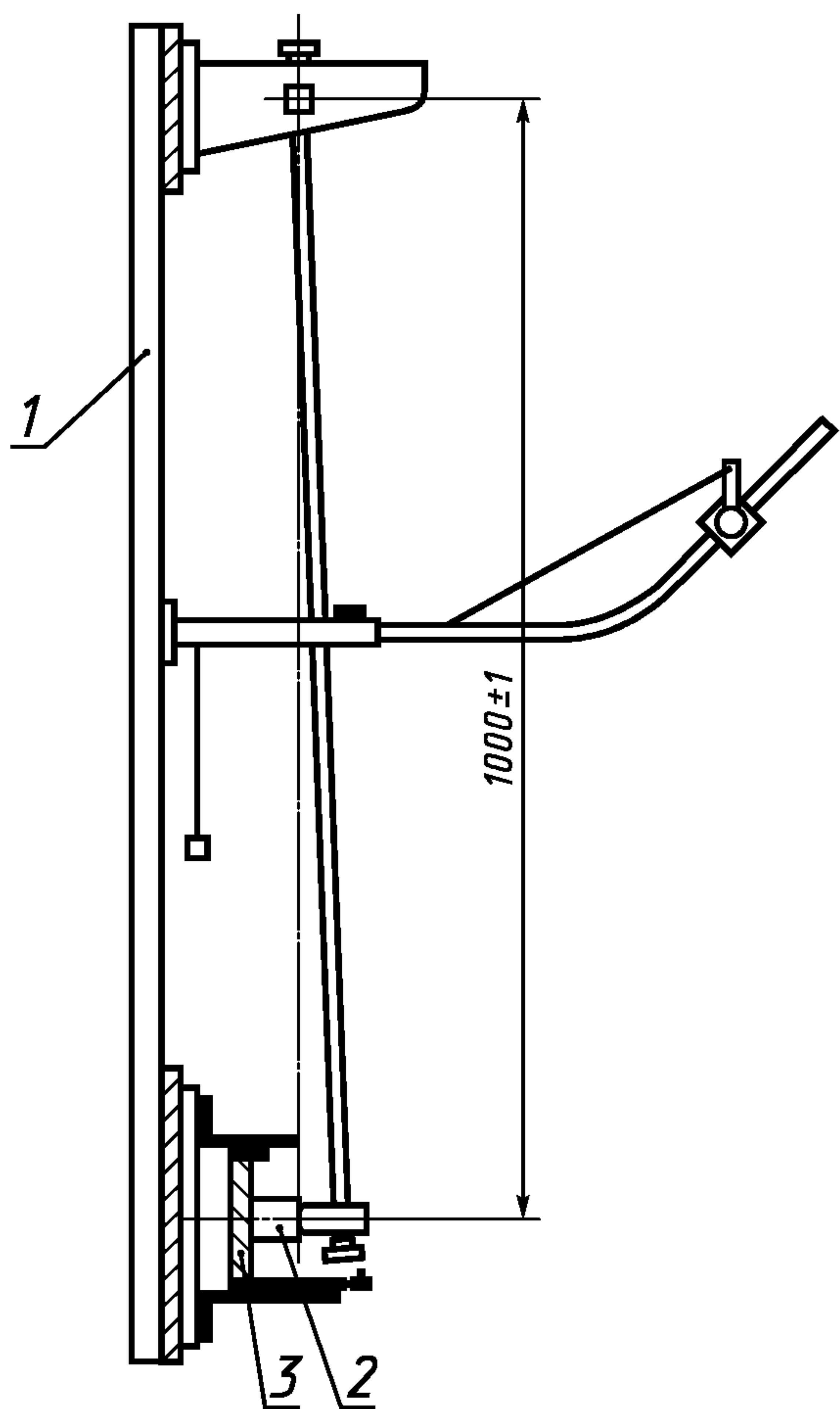
1 — рама; 2 — образец; 3 — монтажная опора
