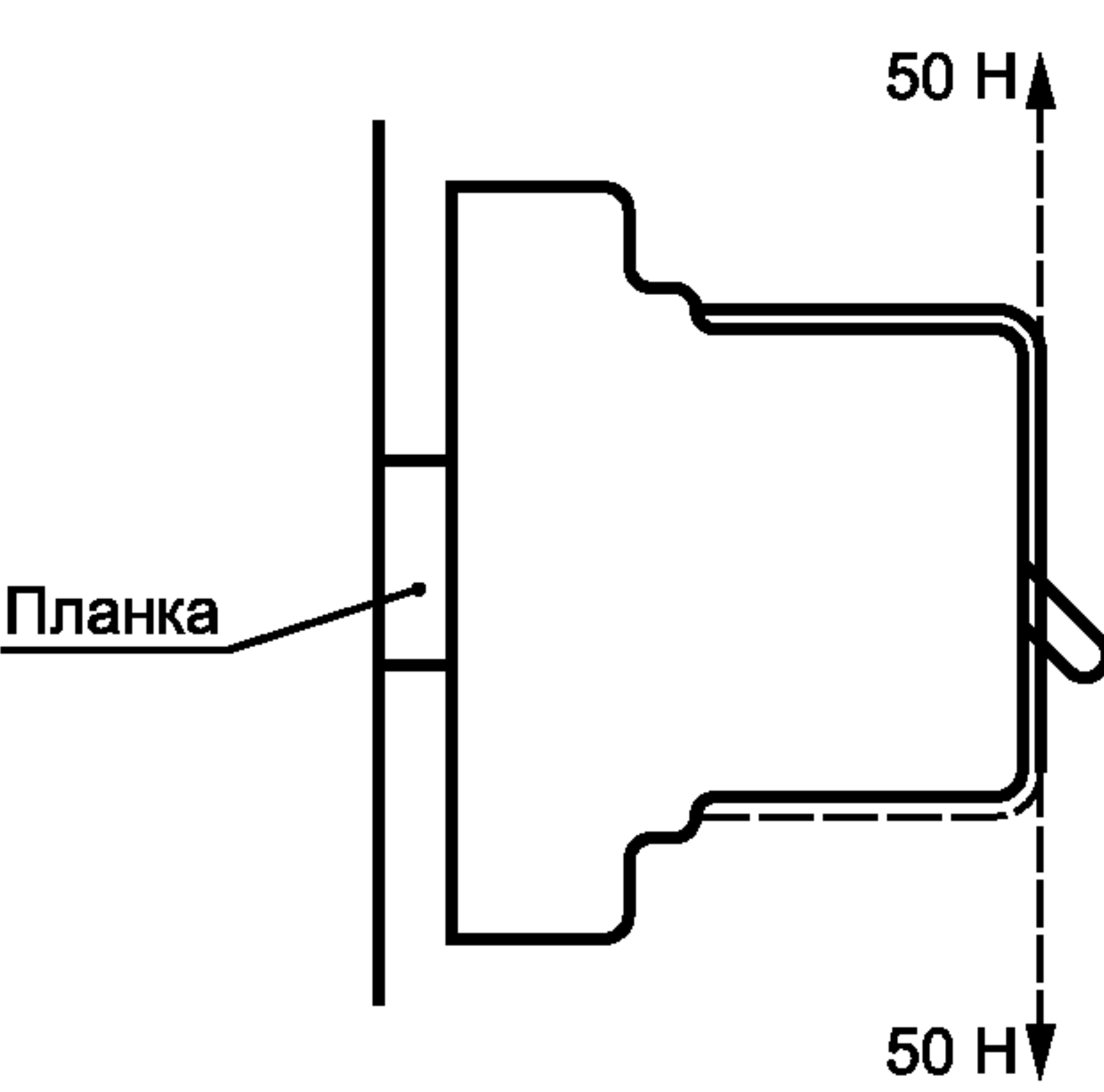
Рисунок 17 — Приложение силы для испытания на механический удар АВДТ, монтируемых на планке (9.13.2.2)
