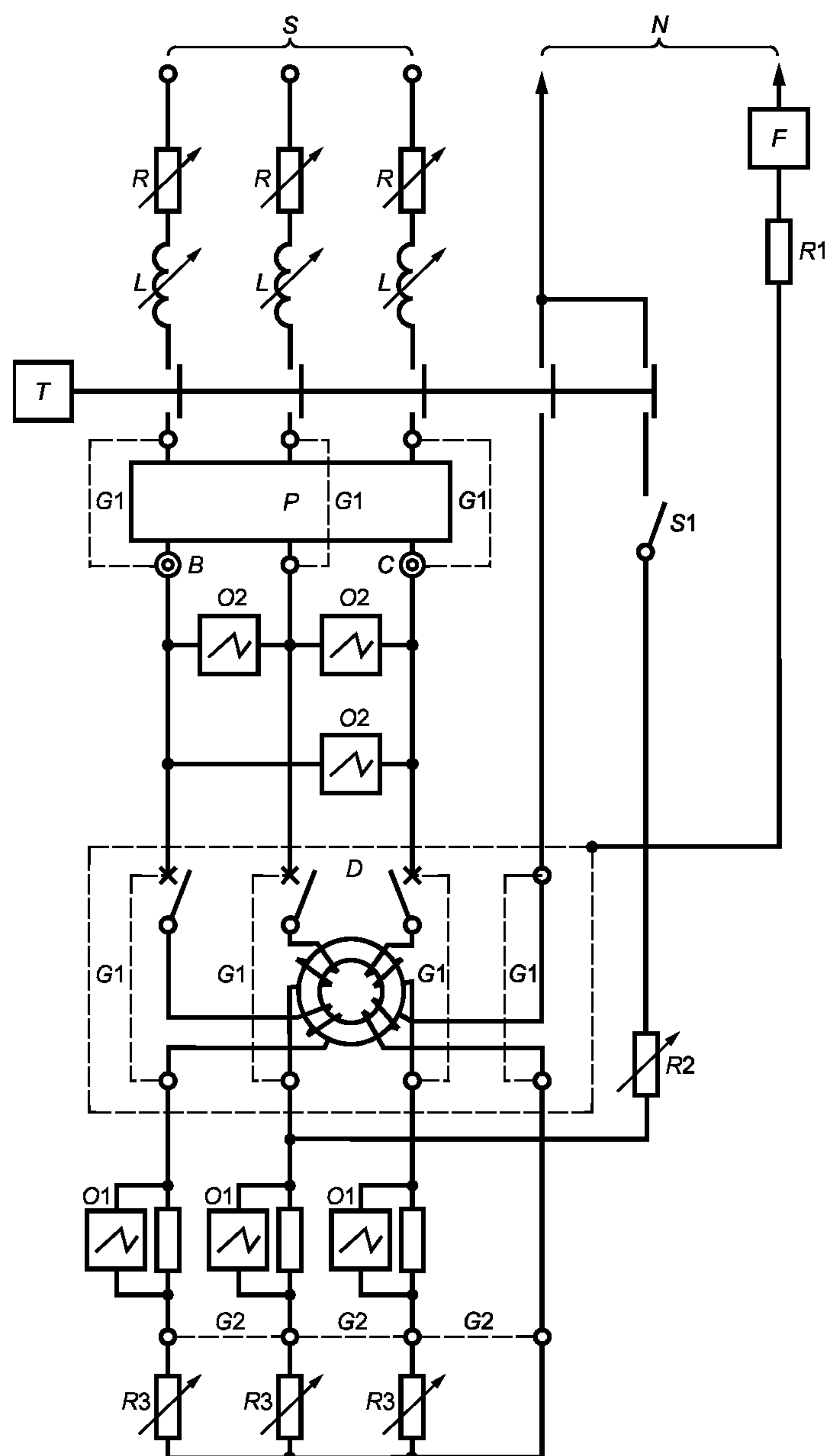
Рисунок 8 — Испытательная цепь для проверки номинальной наибольшей включающей и отключающей способности и координации с ПЗУ трехполусного ВДТ с четырьмя токовыми путями в трехфазной сети с нейтралью (9.11)
