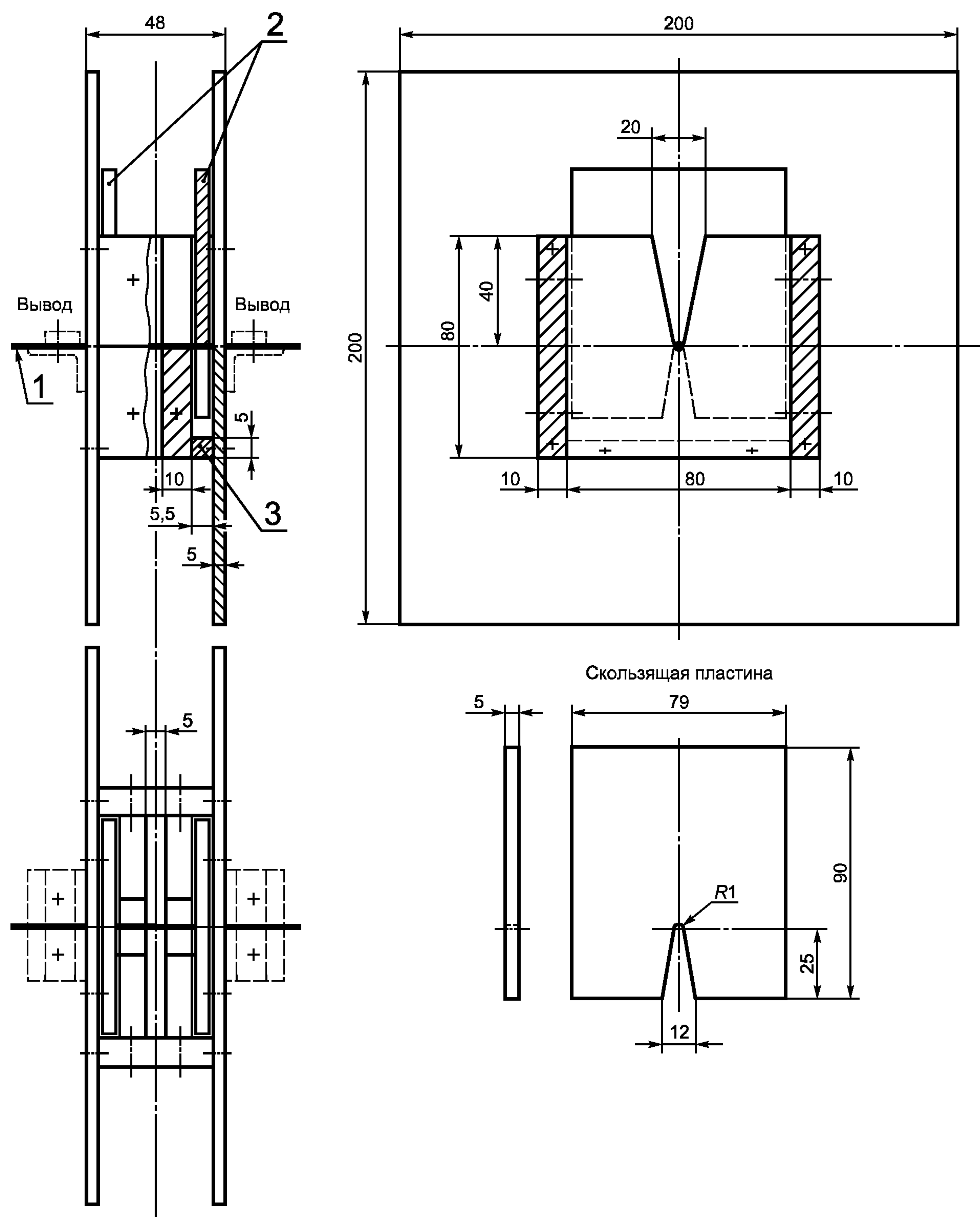
1 — серебряная проволока; 2 — скользящие пластины; 3 — упор для скользящей пластины Рисунок 10 — Испытательное устройство для проверки минимальных значений P_t и I_p , выдерживаемых ВДТ (9.11.2.1a)
