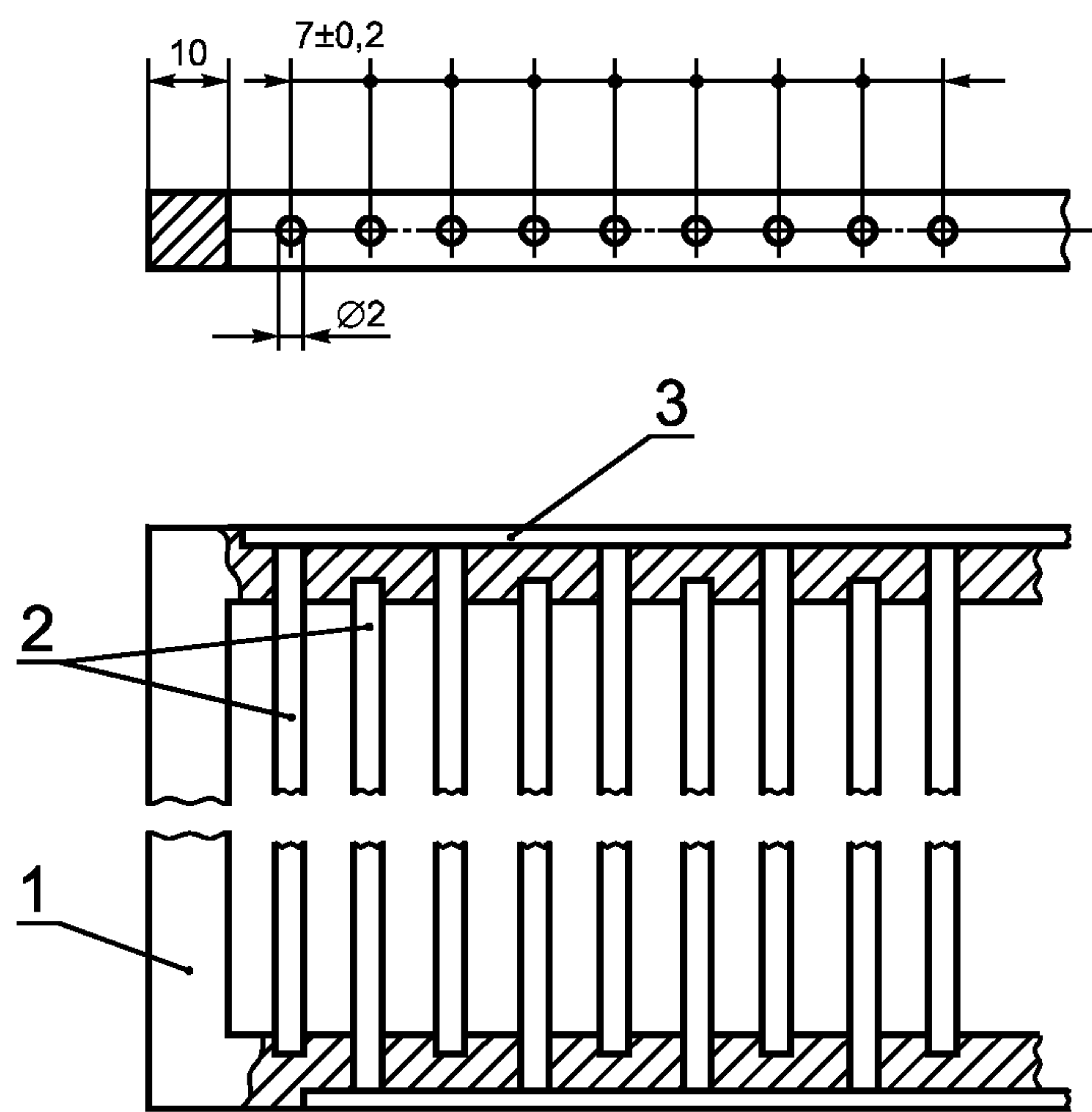
1 — рамка из изоляционного материала; 2 — медные проволочки; 3 — металлическое соединение медных проволок Рисунок С.2 — Сетка
