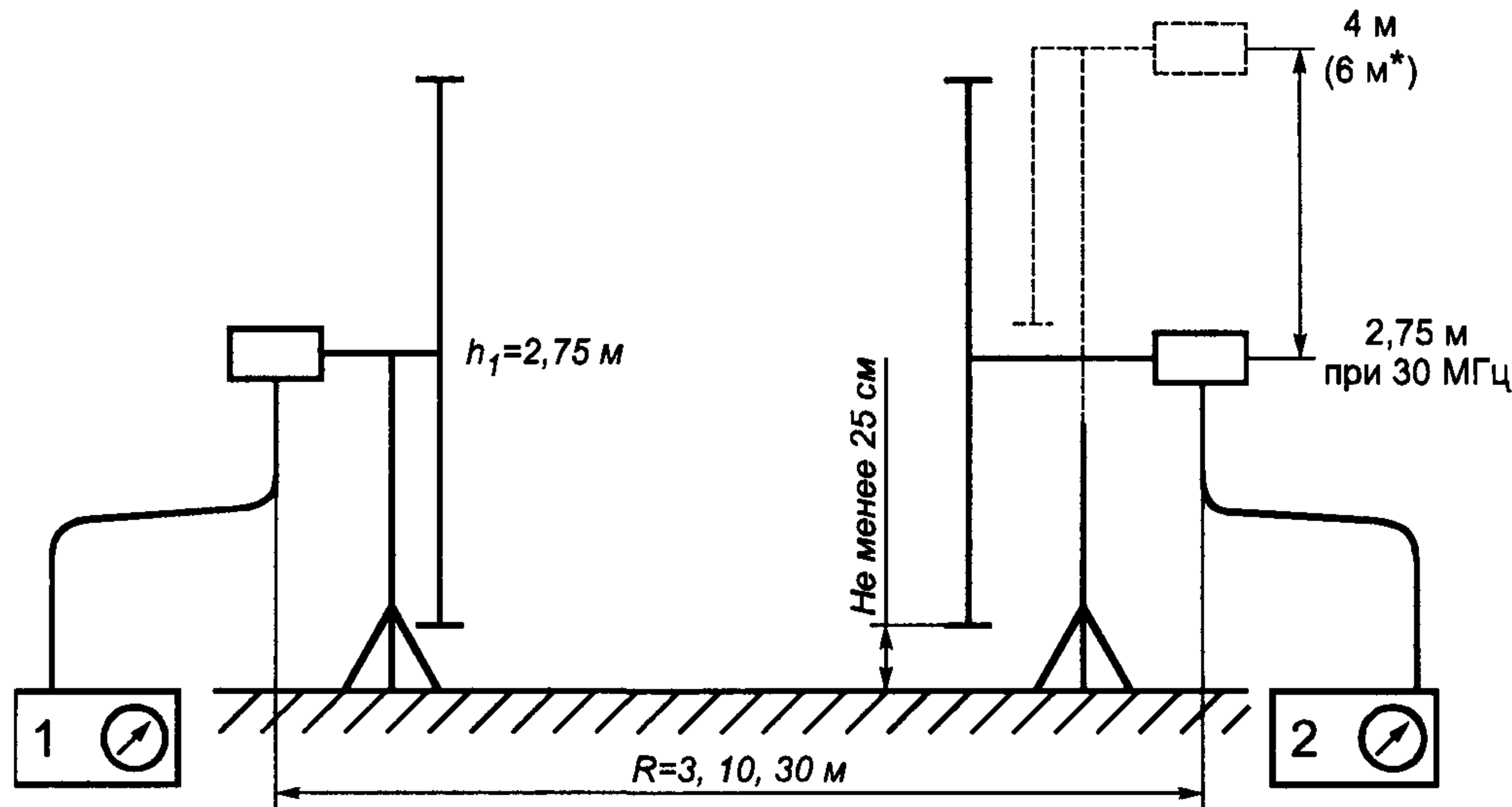
Рисунок Г.1 — Схема измерения затухания площадки при горизонтальной поляризации
