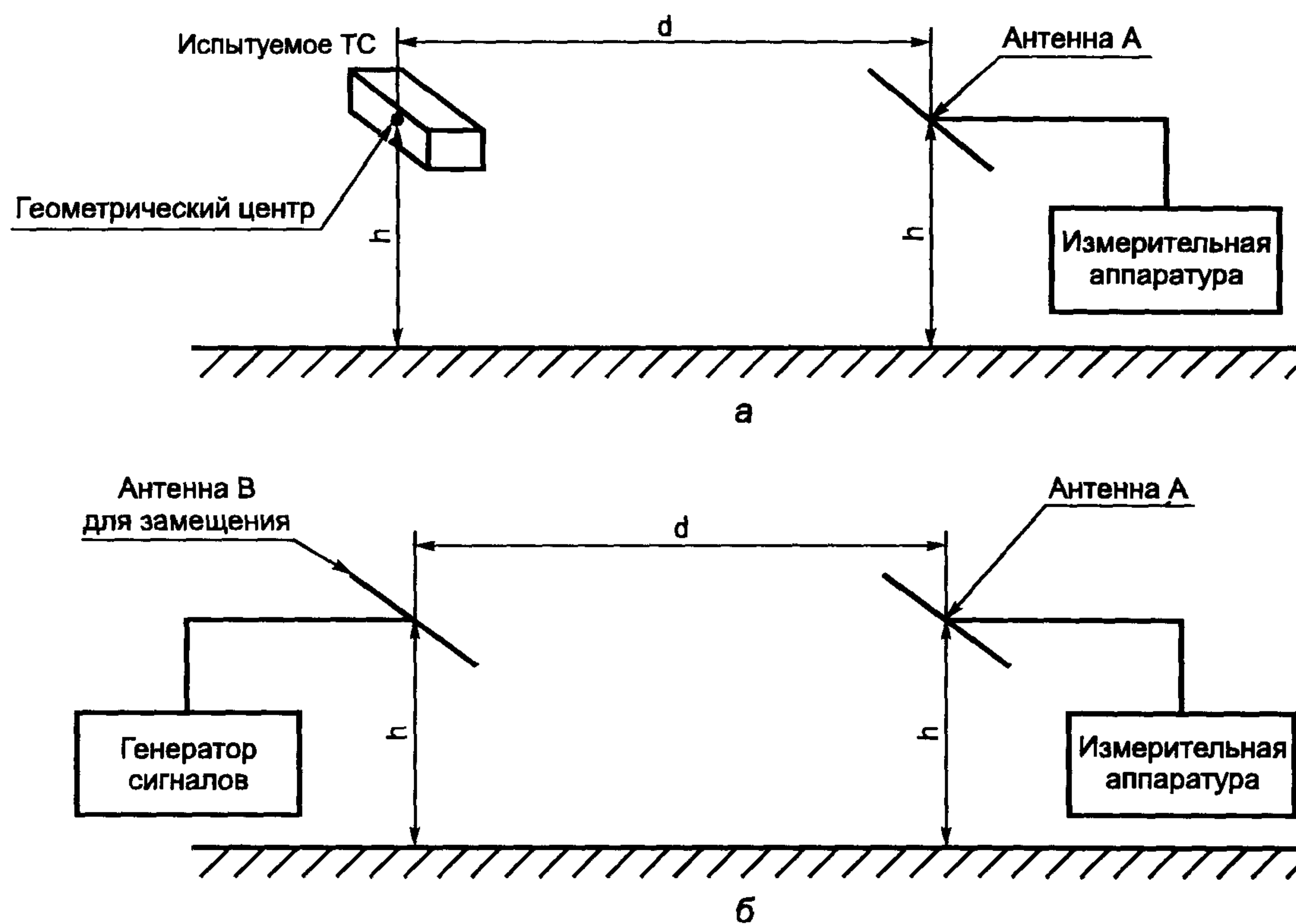
а — измерение; б — калибровка
