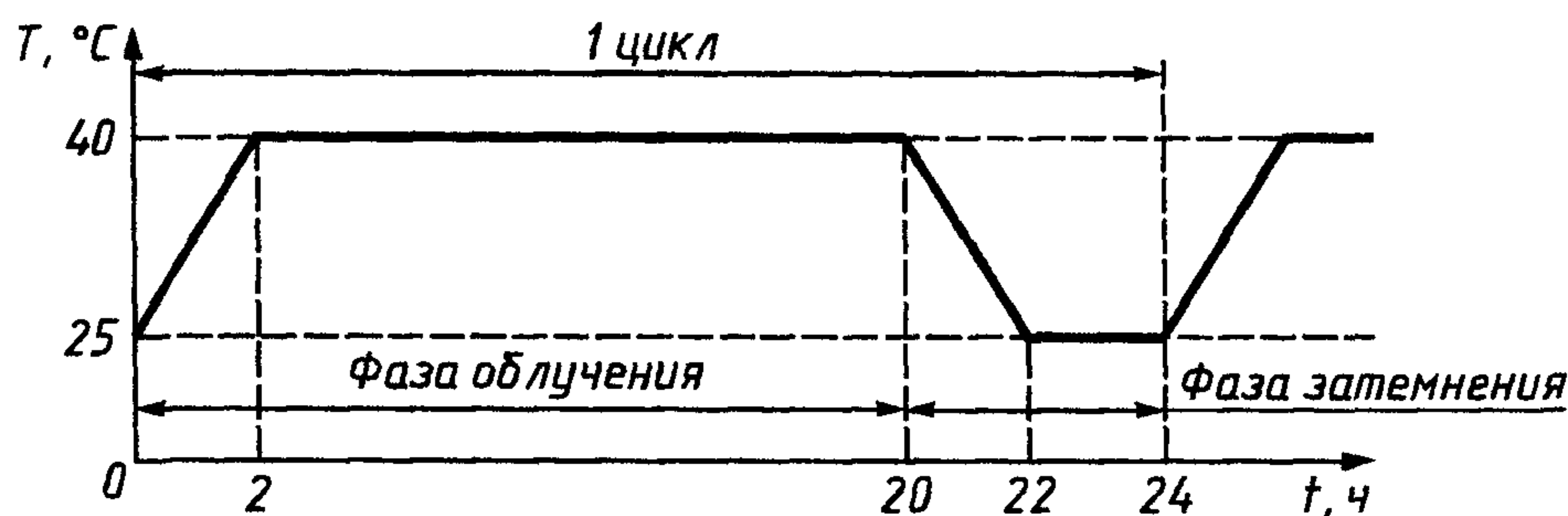
Рисунок 1 — График изменения температуры за один цикл испытаний
