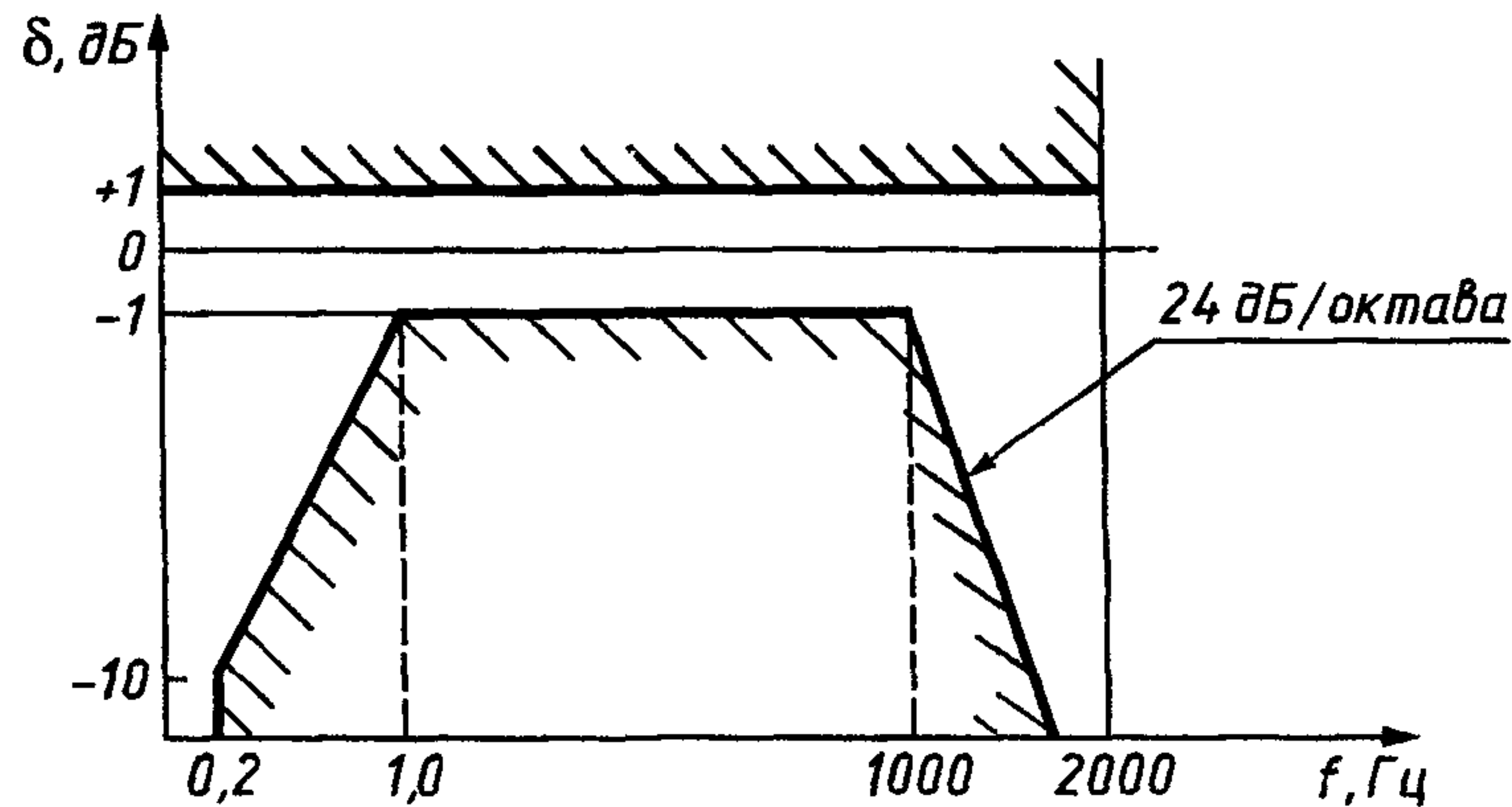
Рисунок А.4 — Амплитудно-частотная характеристика измерительной системы
