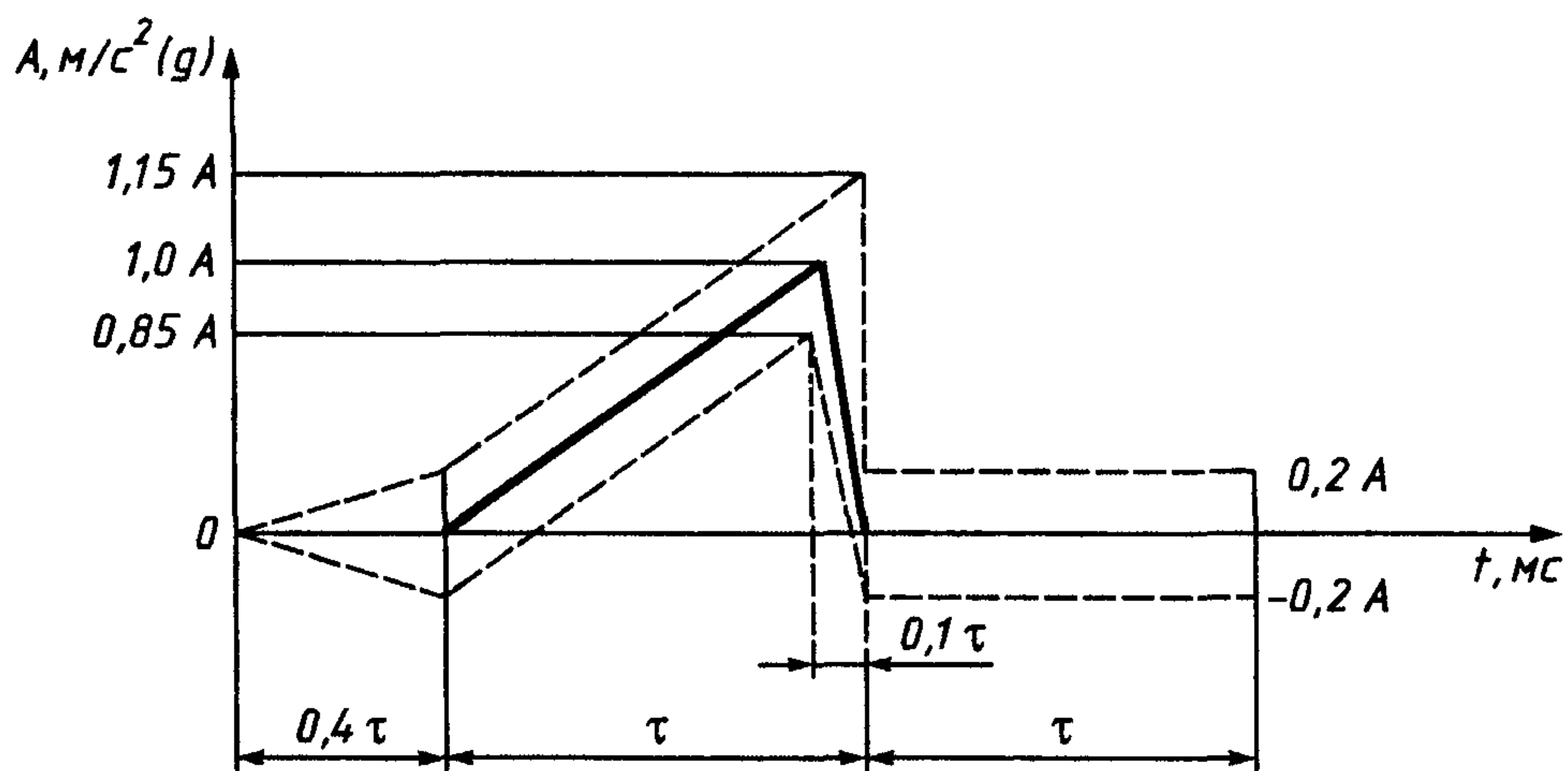
Рисунок А.2 — Треугольный (пилообразный) импульс ударного воздействия
