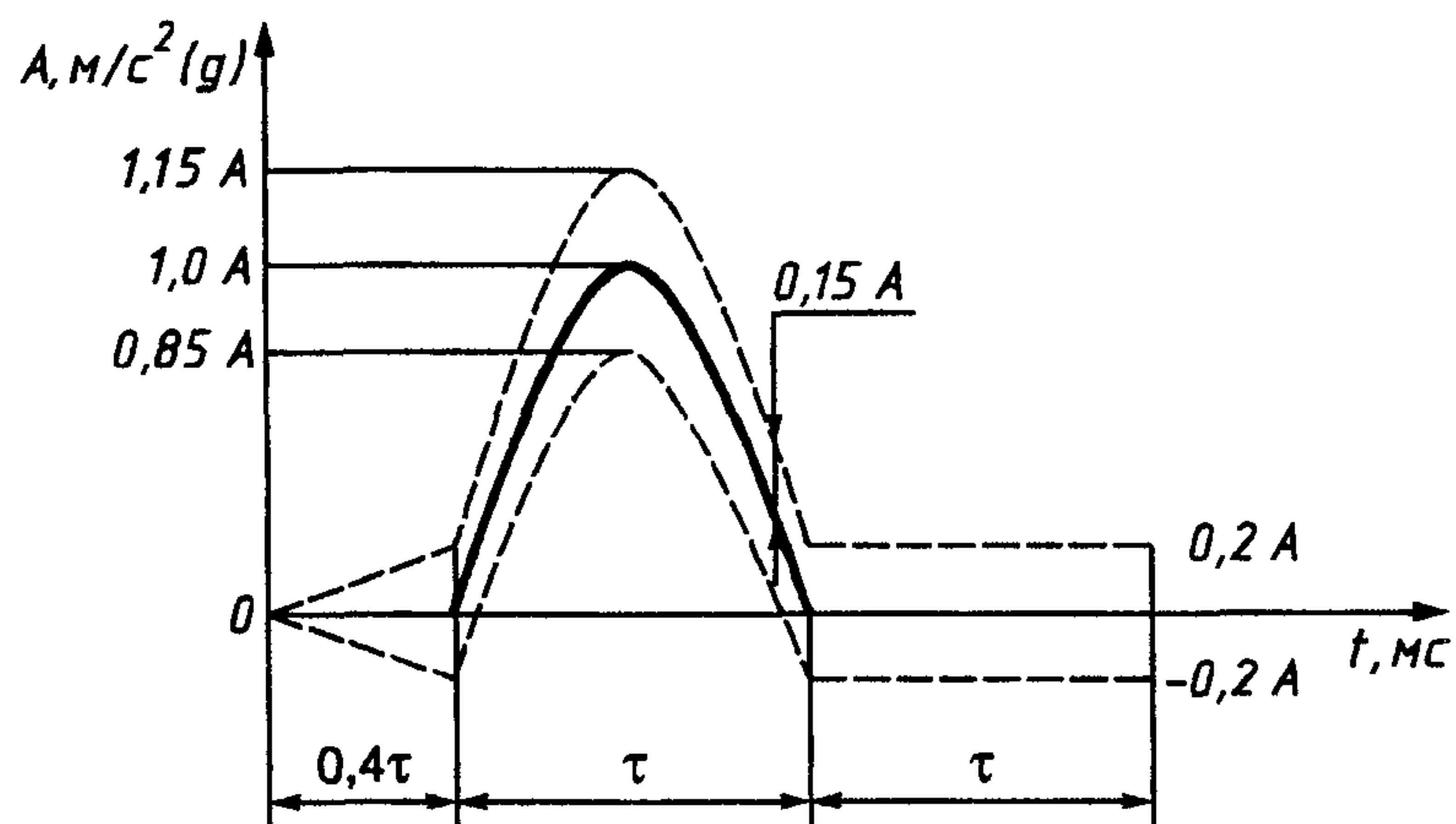
Рисунок А.1 — Полусинусоидальный импульс ударного воздействия
