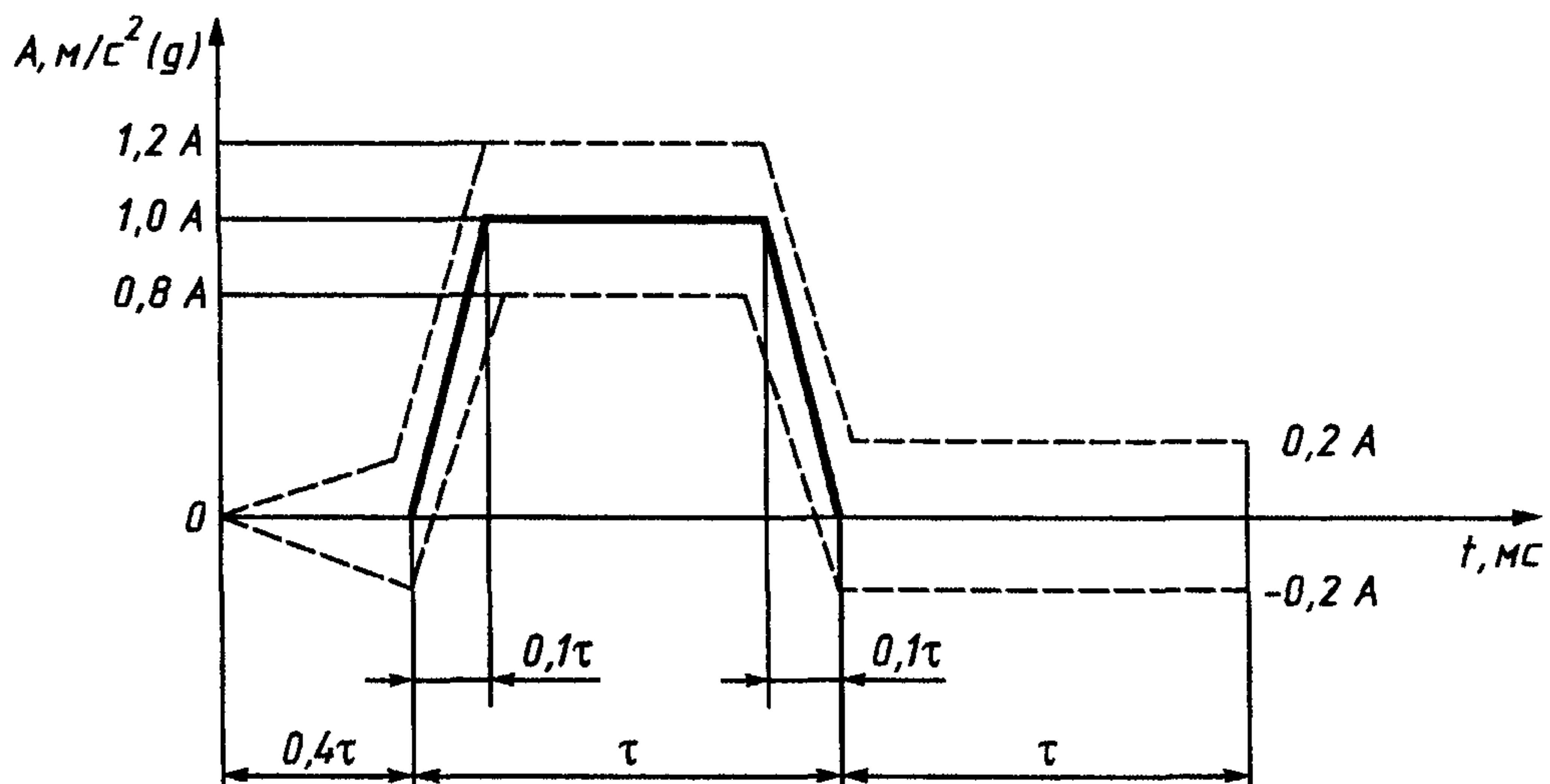
Рисунок А.3 — Трапецеидальный импульс ударного воздействия
