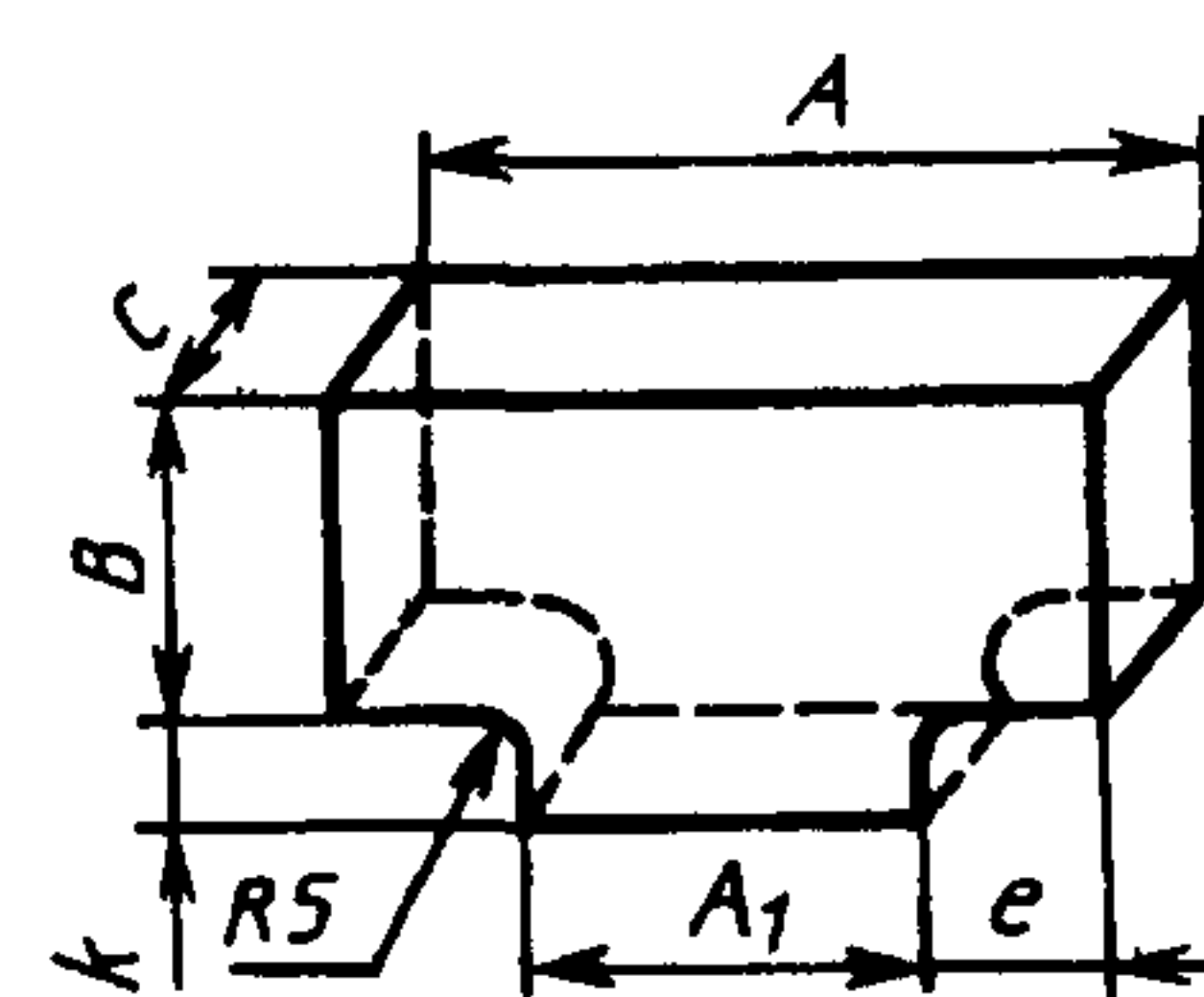
Рисунок 17 — Насадочные изделия номеров 26 — 36
