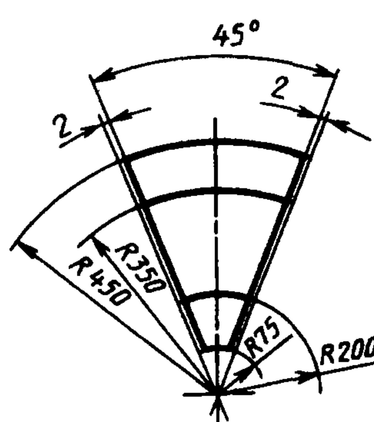
Рисунок 24 — Секторное изделие номер 65
