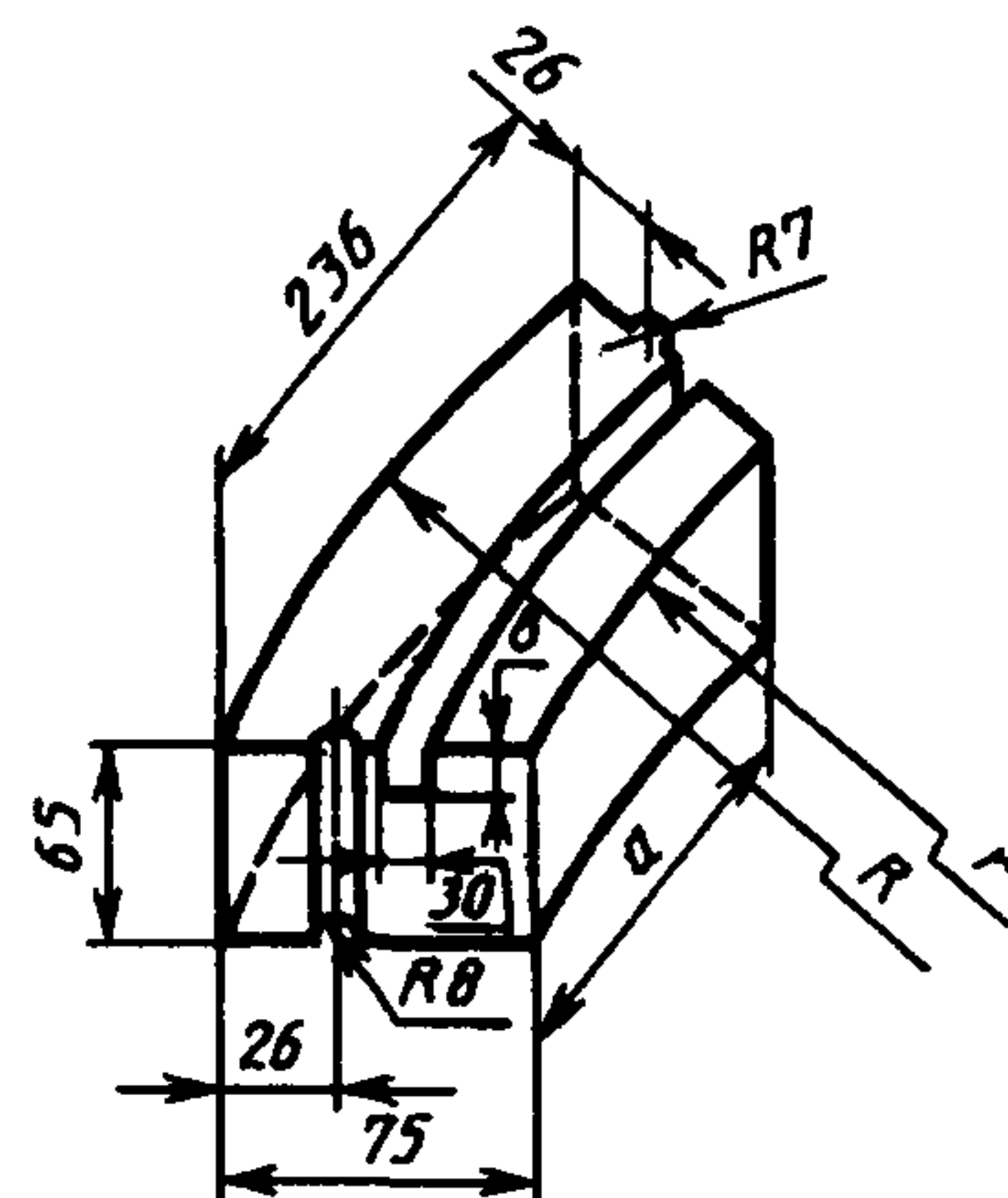
Рисунок 22 — Секторные изделия номеров 57—63
