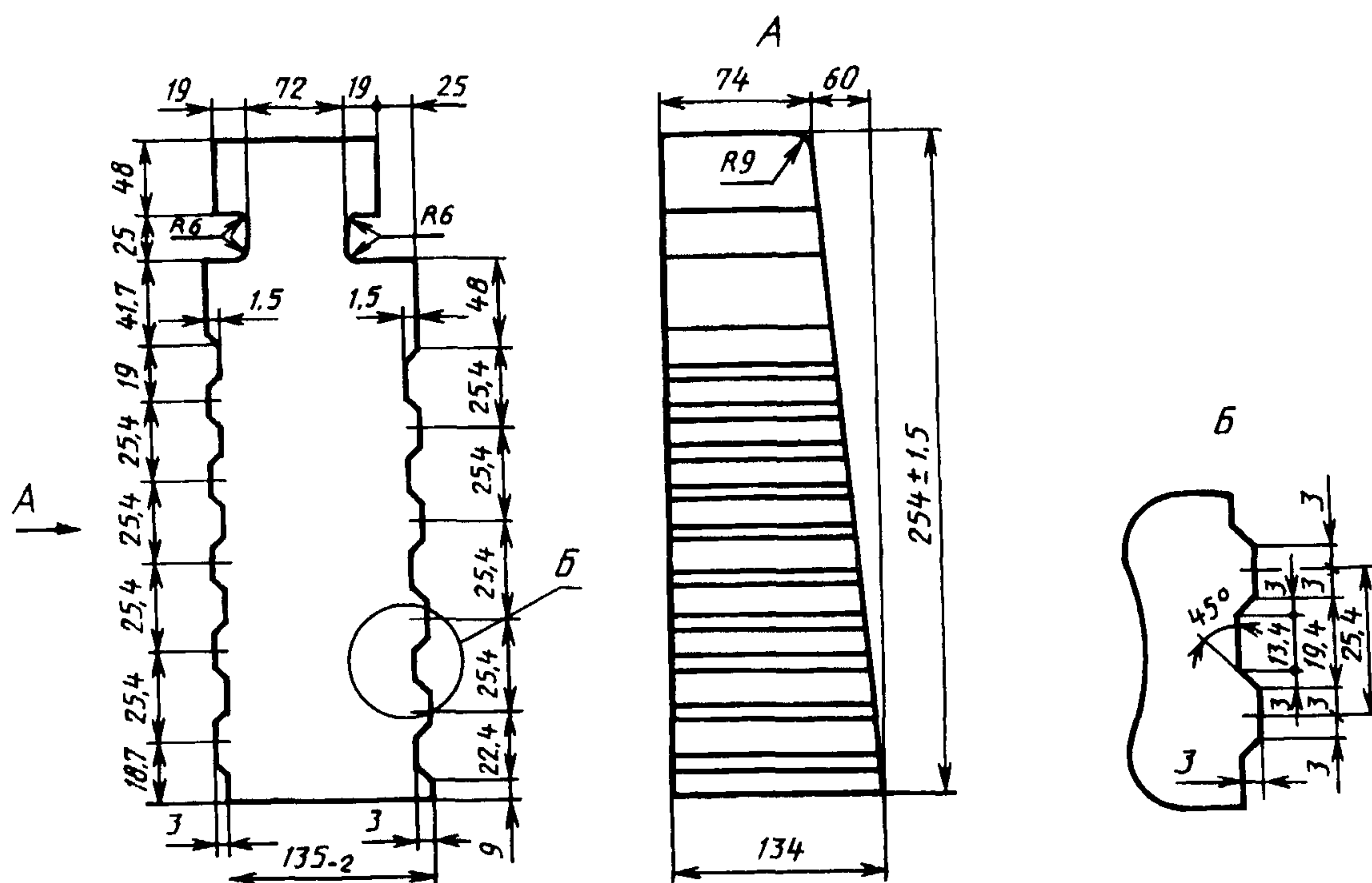
Рисунок 3 — Сводное изделие номер 4
