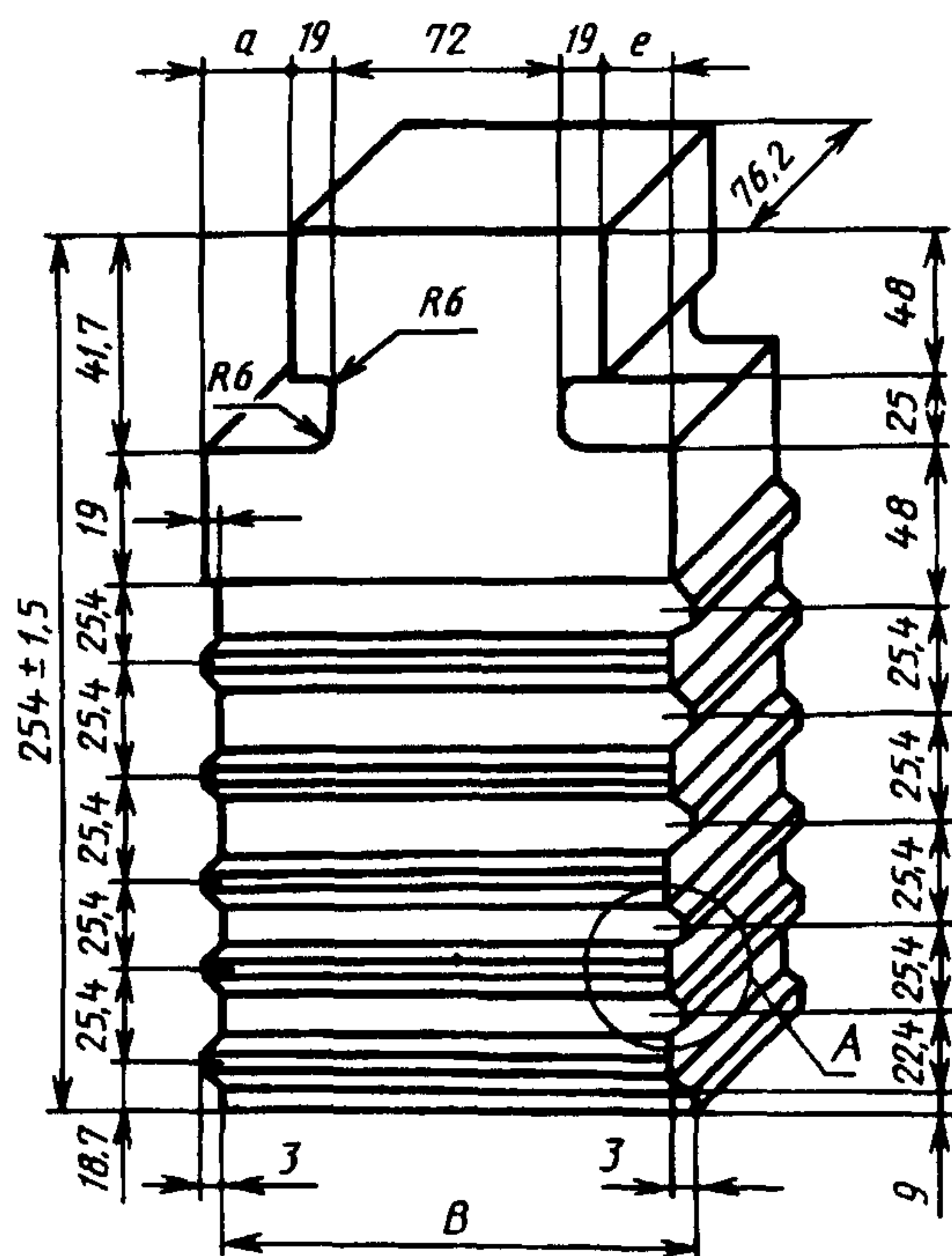
Рисунок 13 — Сводовые изделия номеров 18—20
