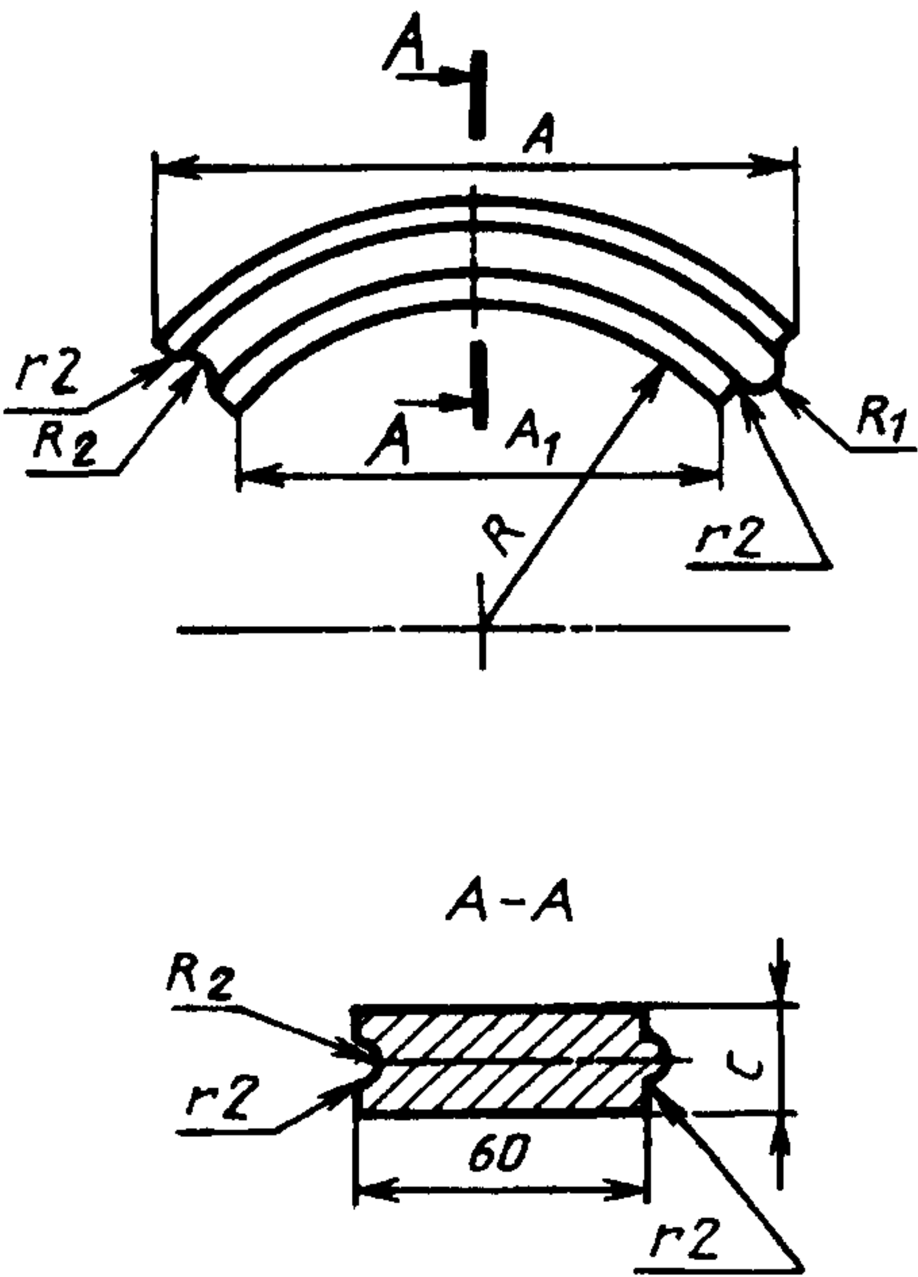
Рисунок 28 — Секторные изделия номеров 73—84
