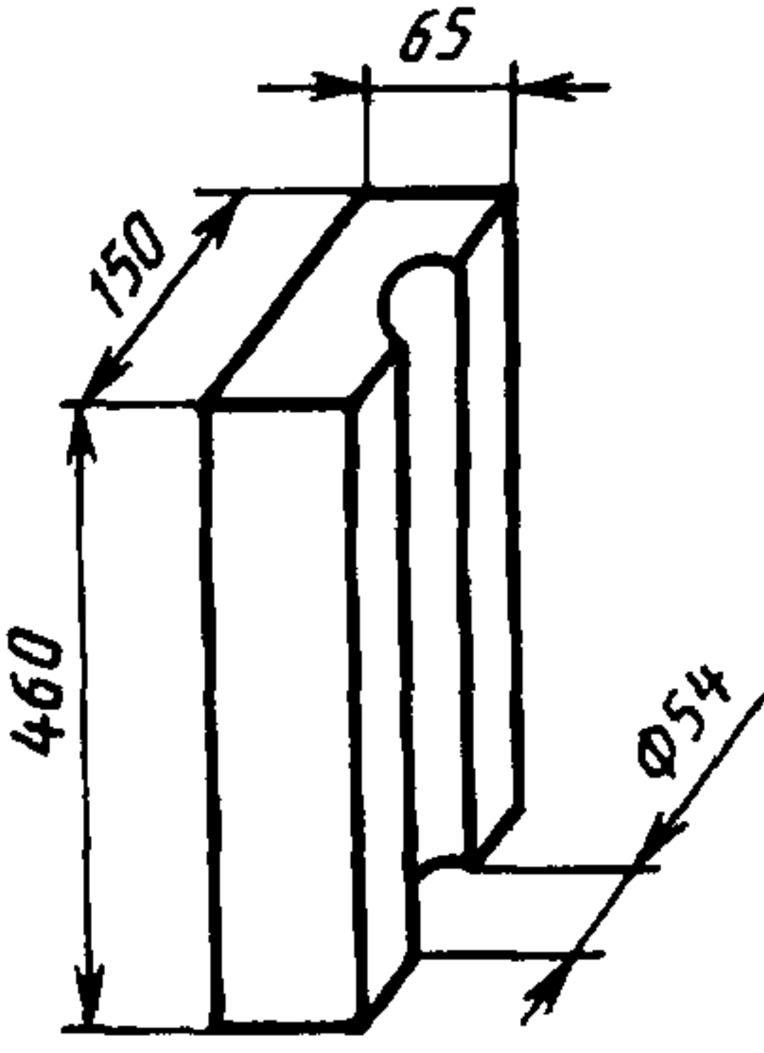
Рисунок 31 — Изделие с контрольным отверстием номер 88
