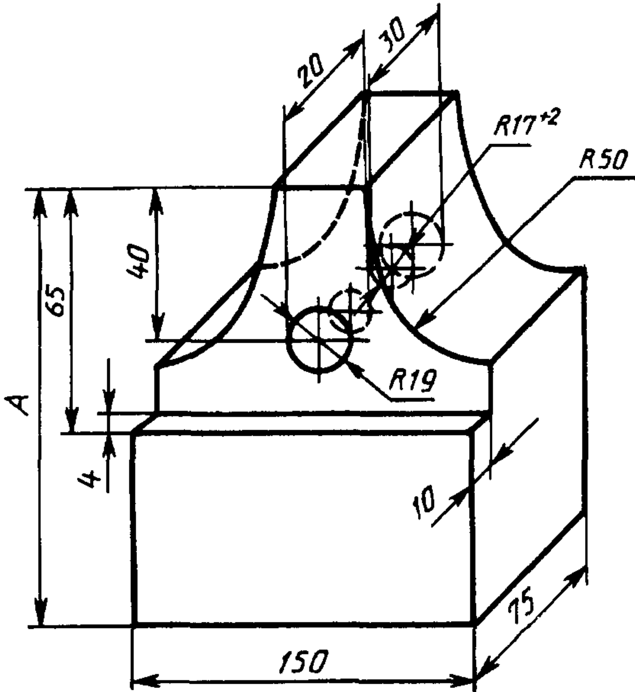
Рисунок 1 — Сводовые изделия номеров 1, 2
