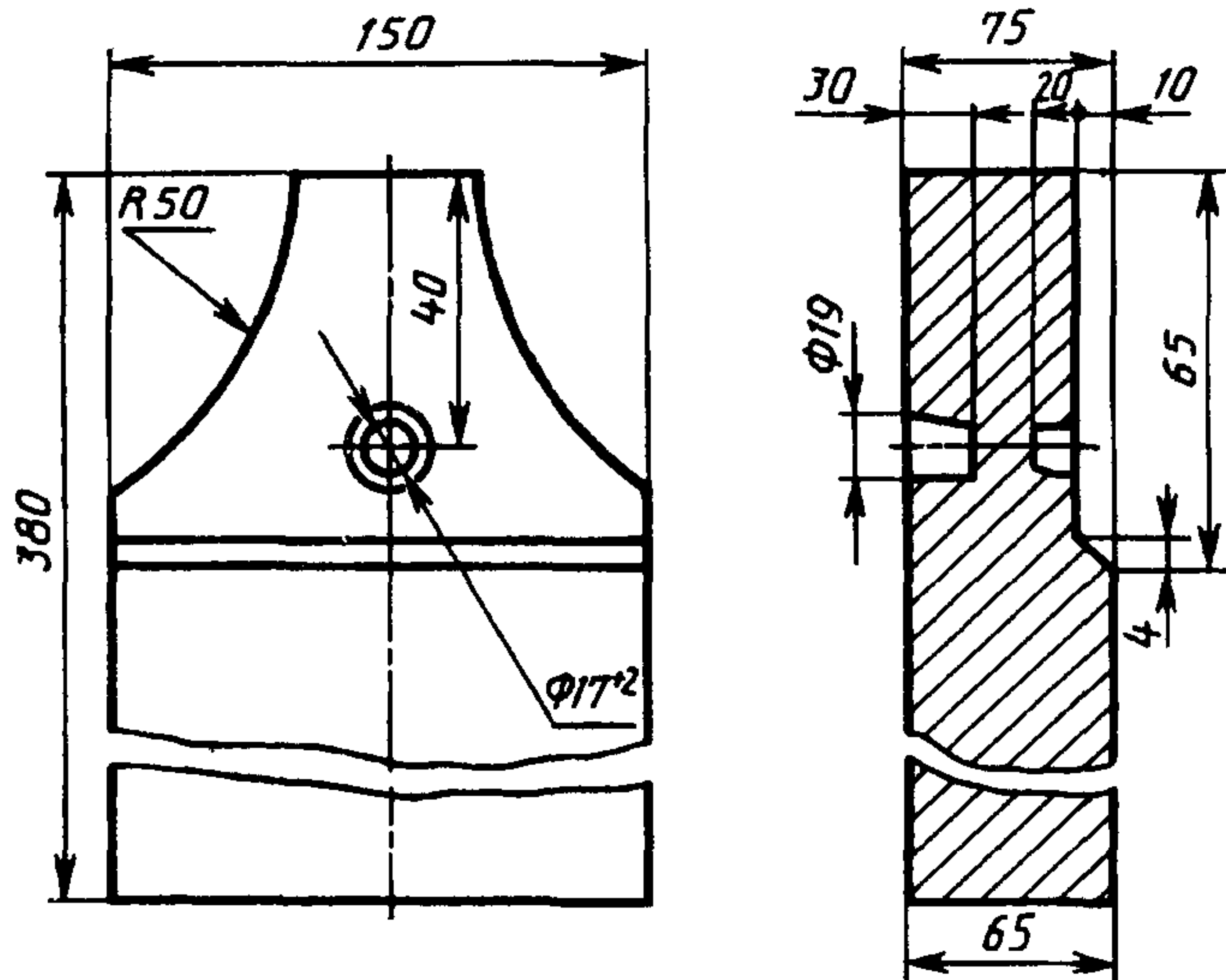
Рисунок 2 — Сводовое изделие номер 3
