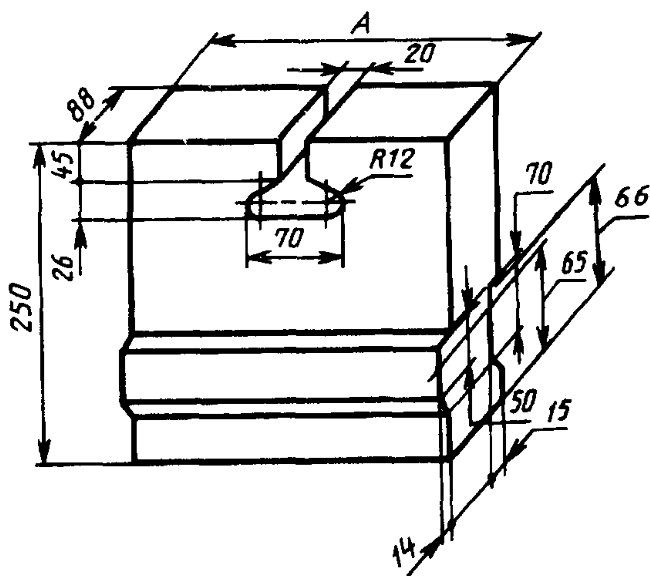
Рисунок 15 — Сводовые изделия номеров 23, 24
