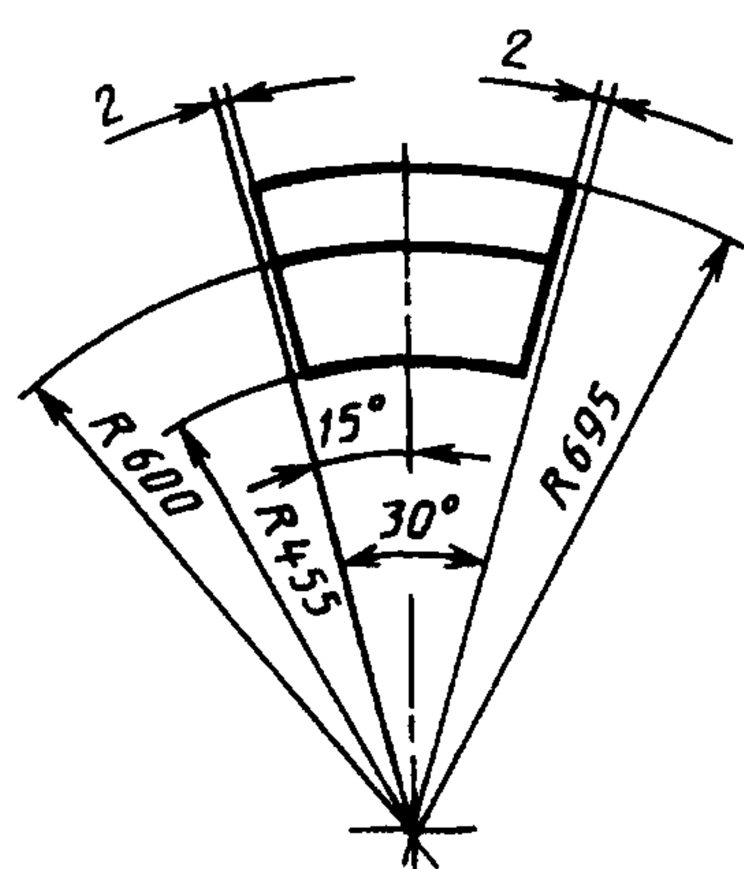
Рисунок 23 — Секторное изделие номер 64
