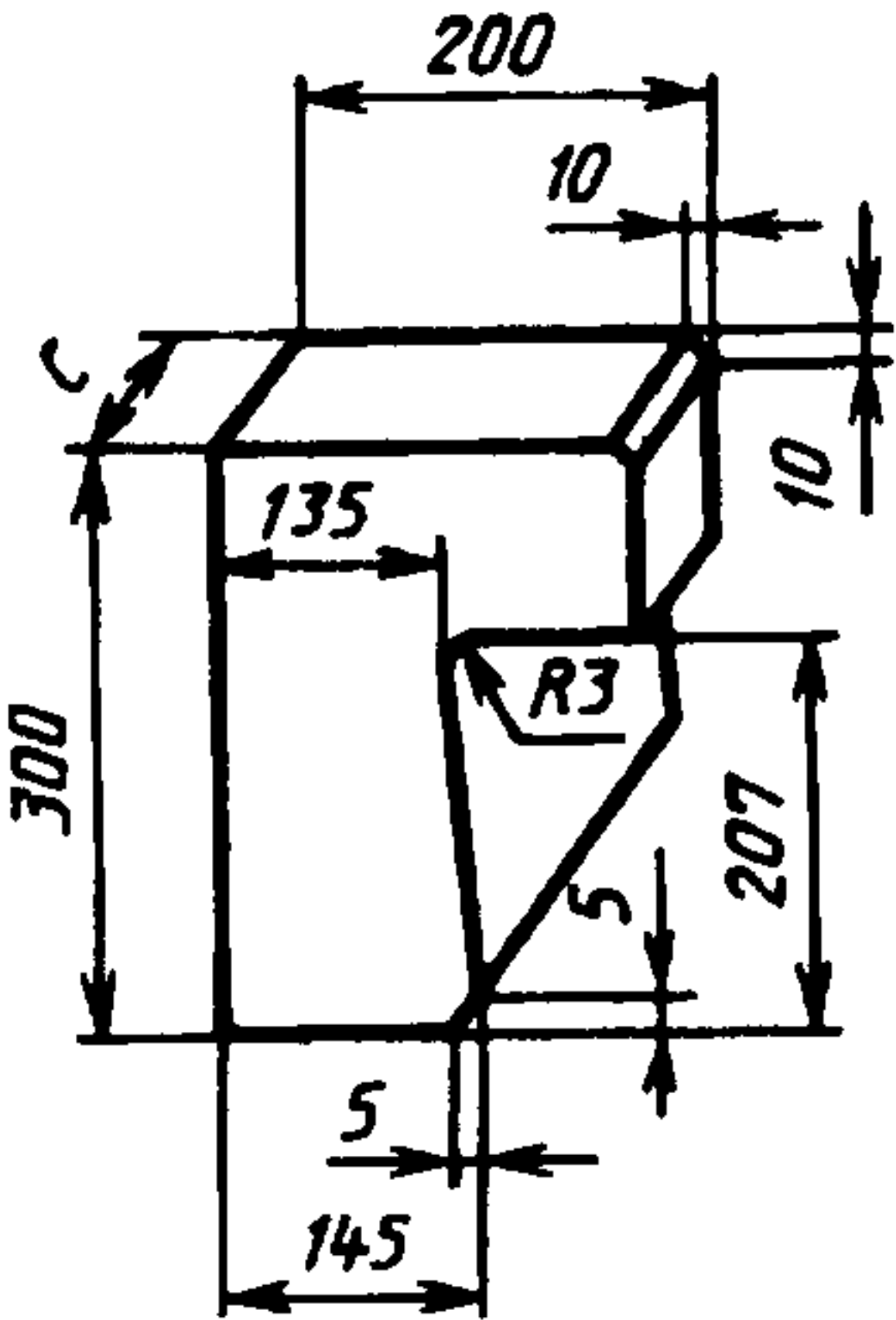
Рисунок 29 — Бортовые изделия номеров 85, 86
