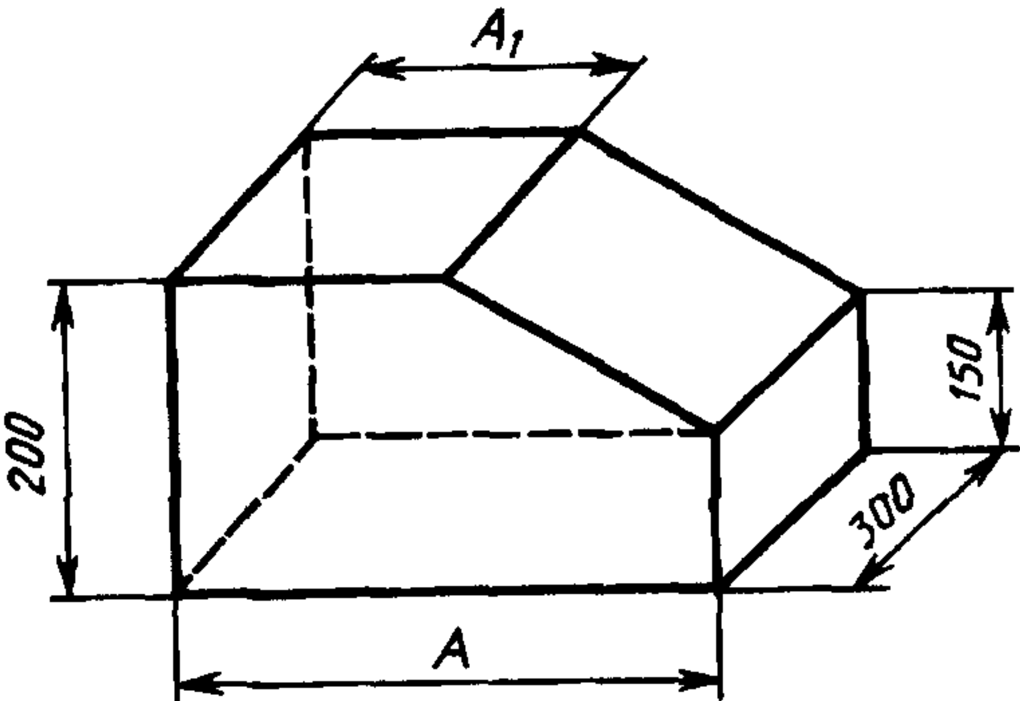
Рисунок 33 — Фасонный брус — изделия номеров 90, 91
