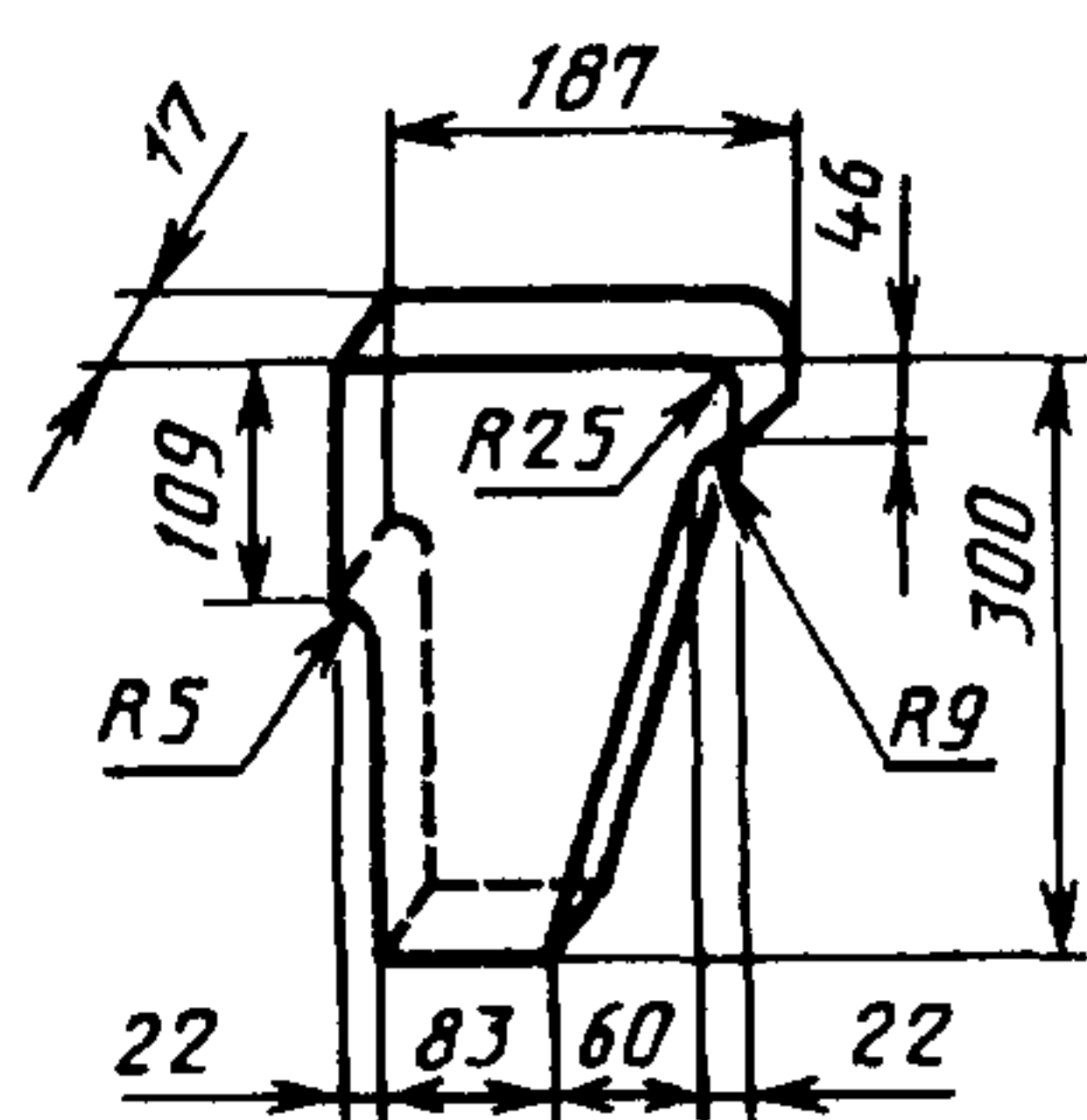
Рисунок 5 — Сводное изделие номер 6
