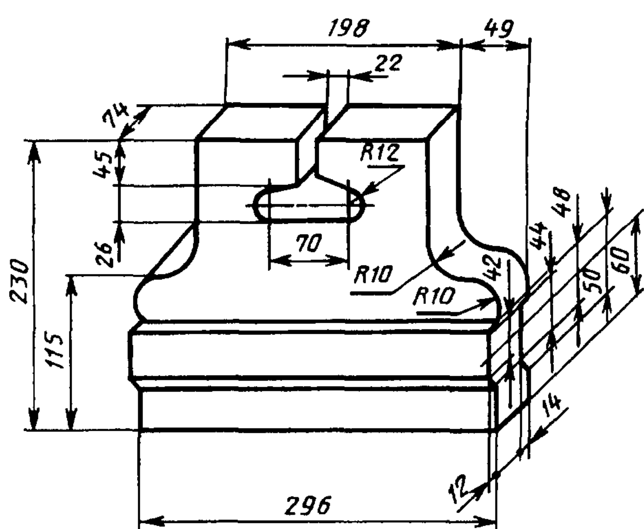
Рисунок 6 — Сводное изделие номер 7
