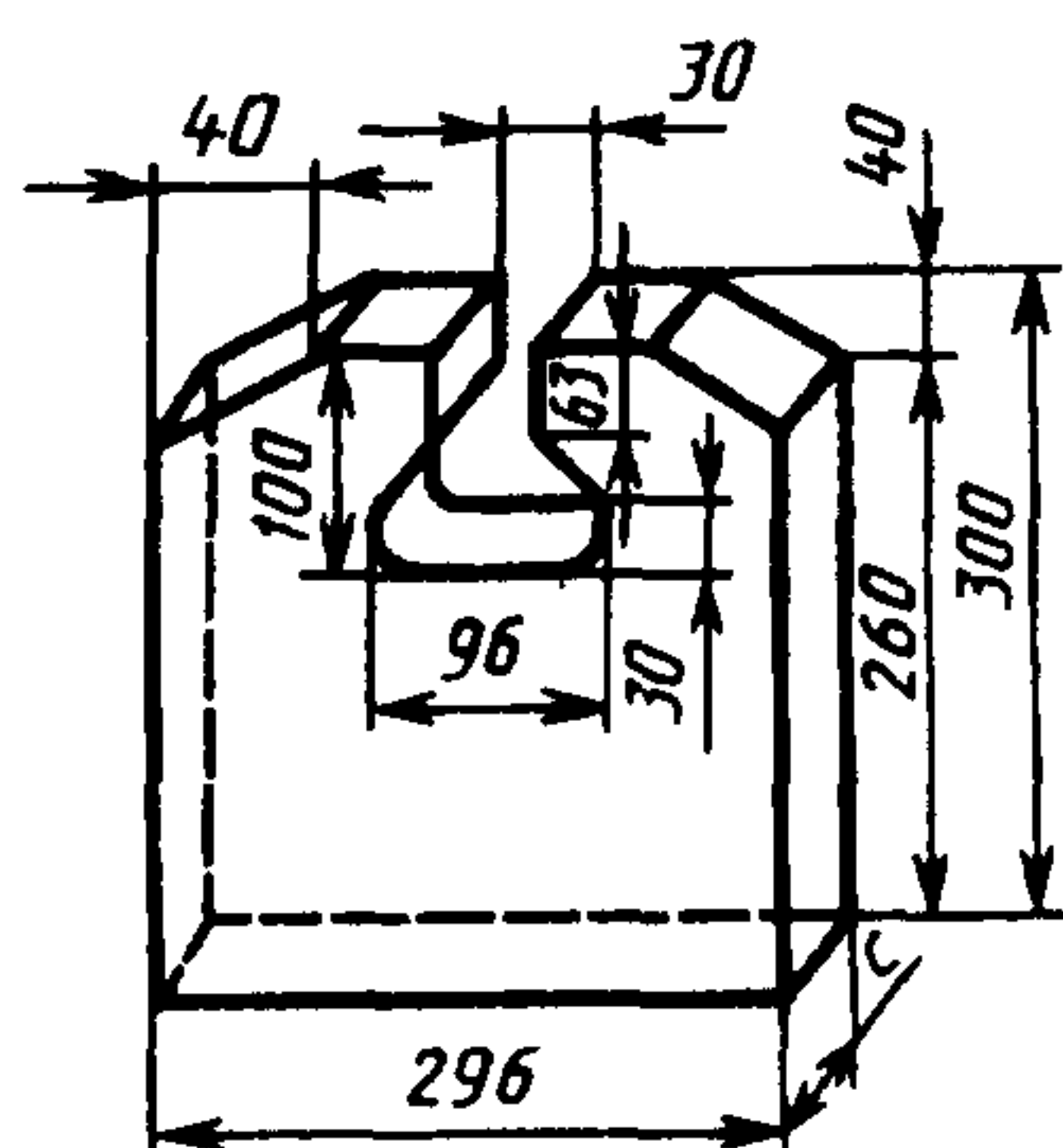
Рисунок 14 — Сводовые изделия номеров 21, 22
