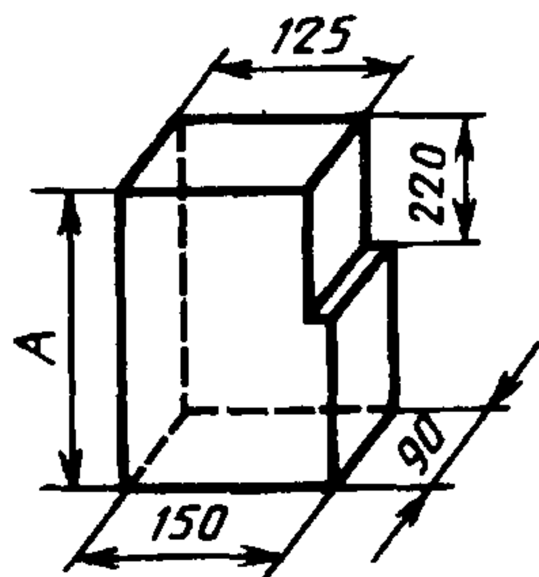
Рисунок 19 — Насадочные изделия номеров 43 — 48
