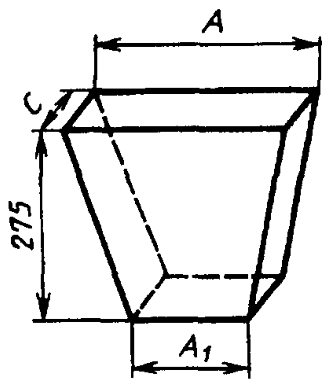
Рисунок 19 — Насадочные изделия номеров 43 — 48
