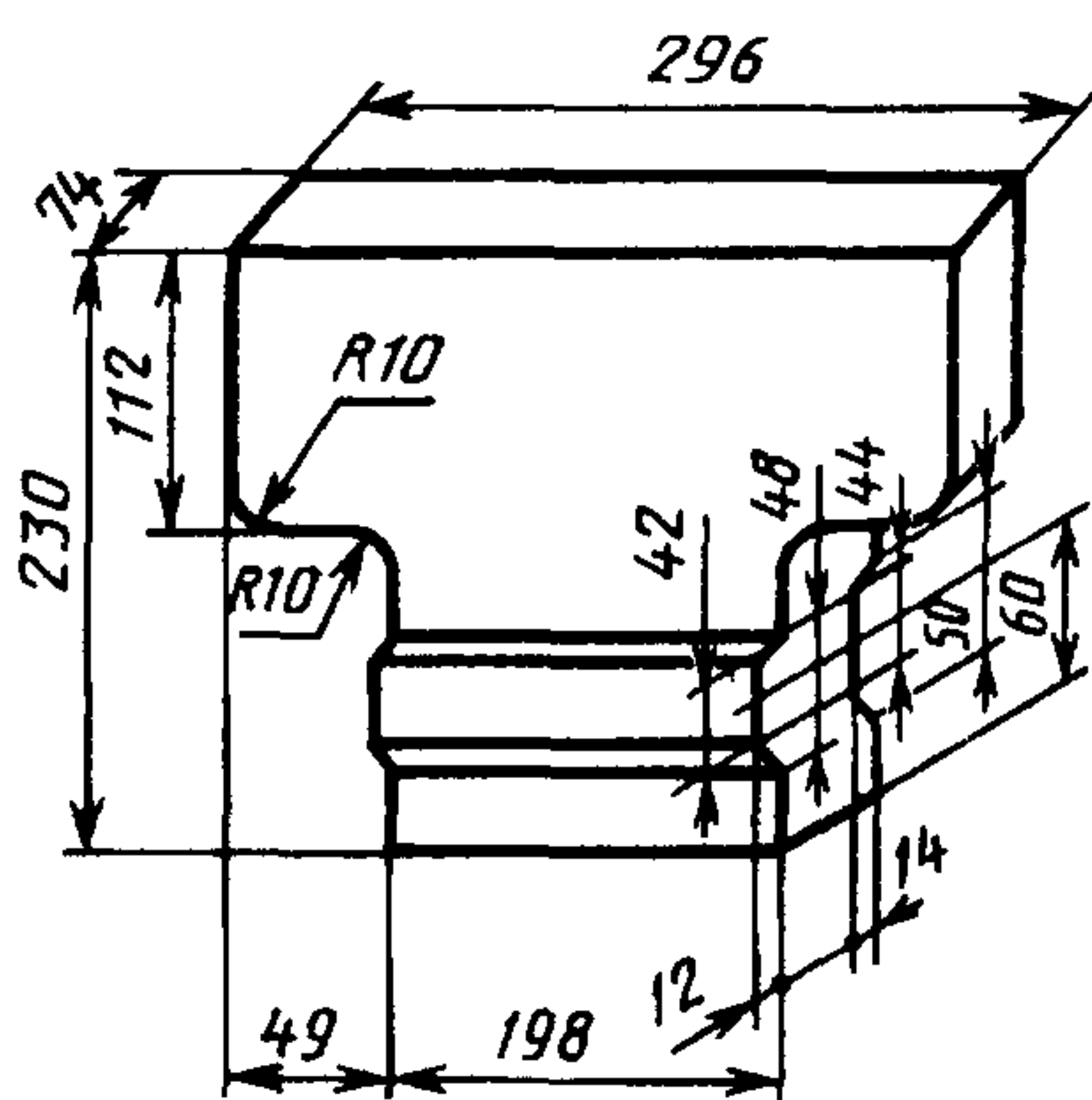
Рисунок 7 — Сводное изделие номер 8
