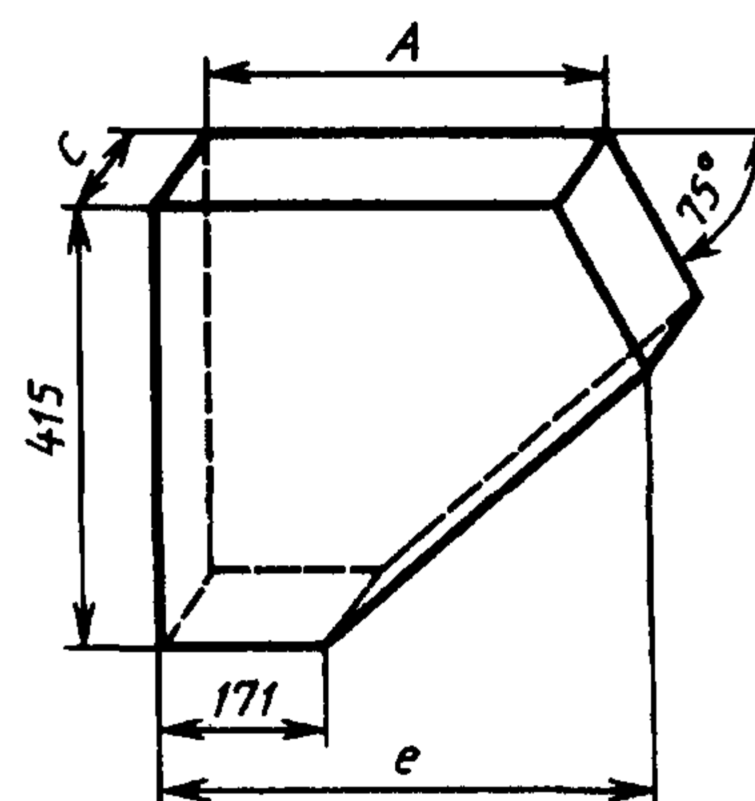
Рисунок 18 — Насадочные изделия номеров 37 — 42
