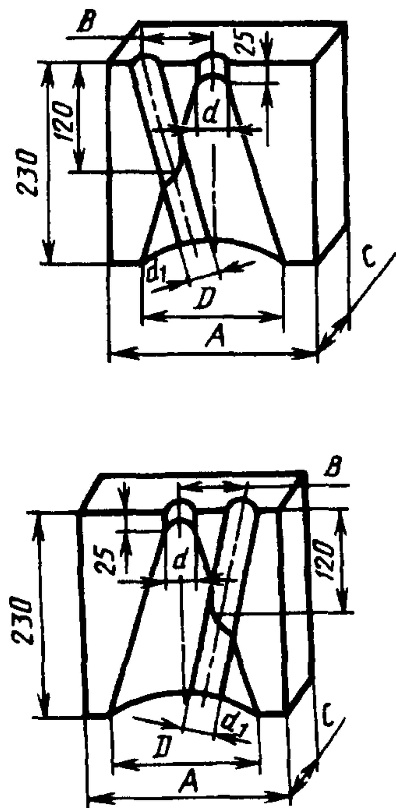
Рисунок 21 — Горелочные изделия номеров 52—56
