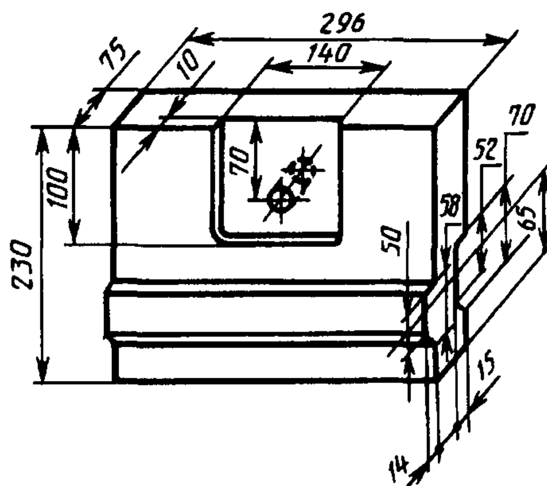
Рисунок 16 — Сводное изделие номер 25
