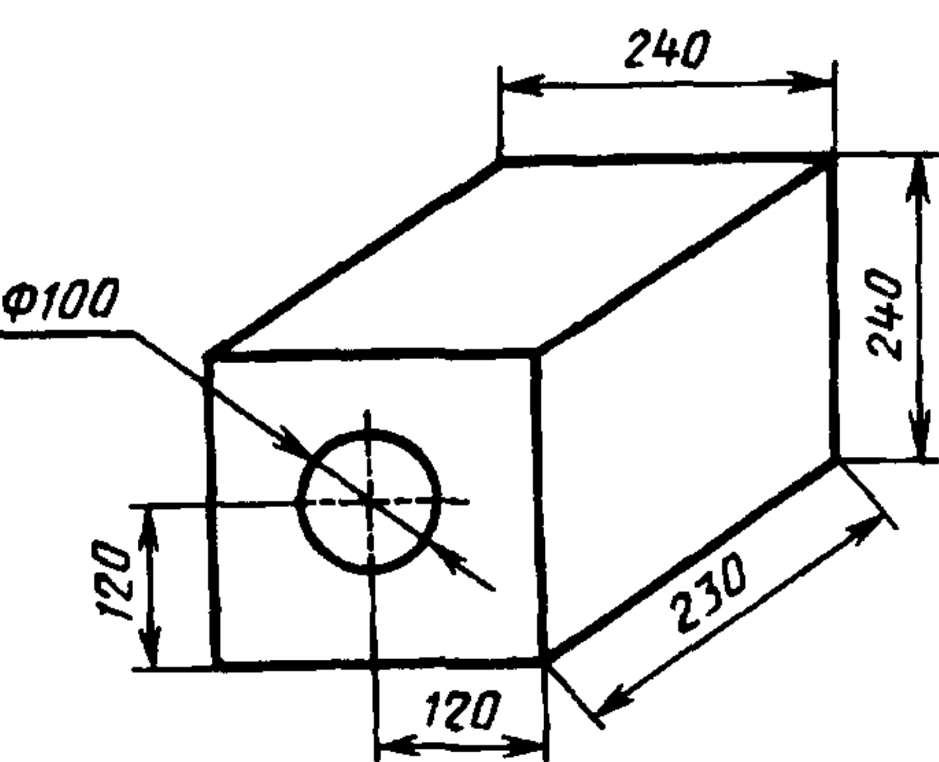
Рисунок 30 — Изделие с контрольным отверстием номер 87
