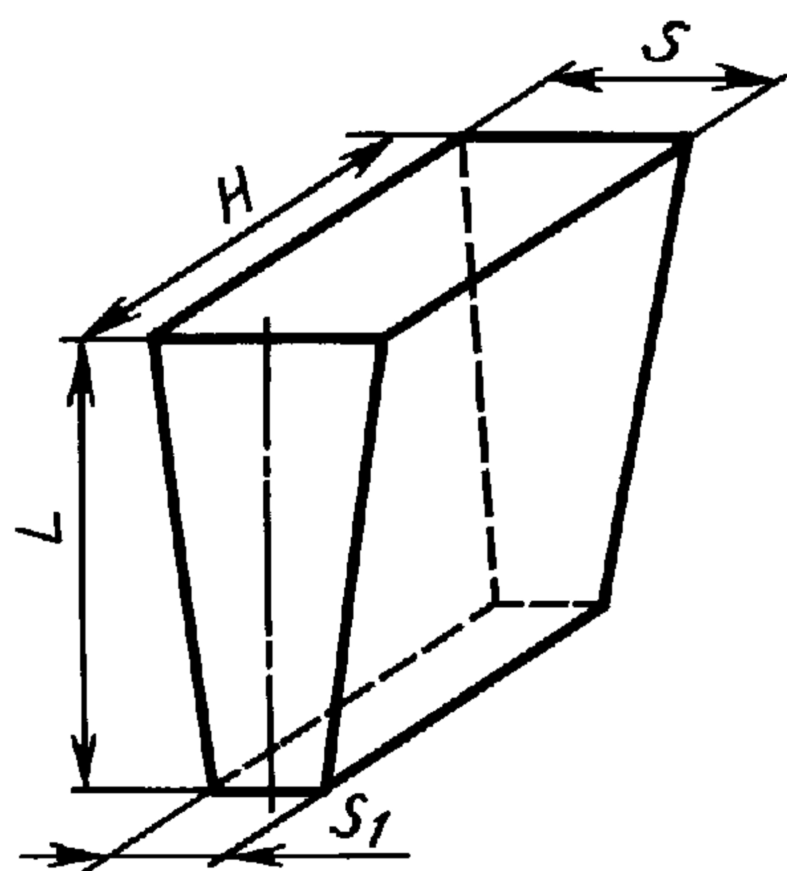
Рисунок 5 — Клин торцовый полуторный двусторонний
