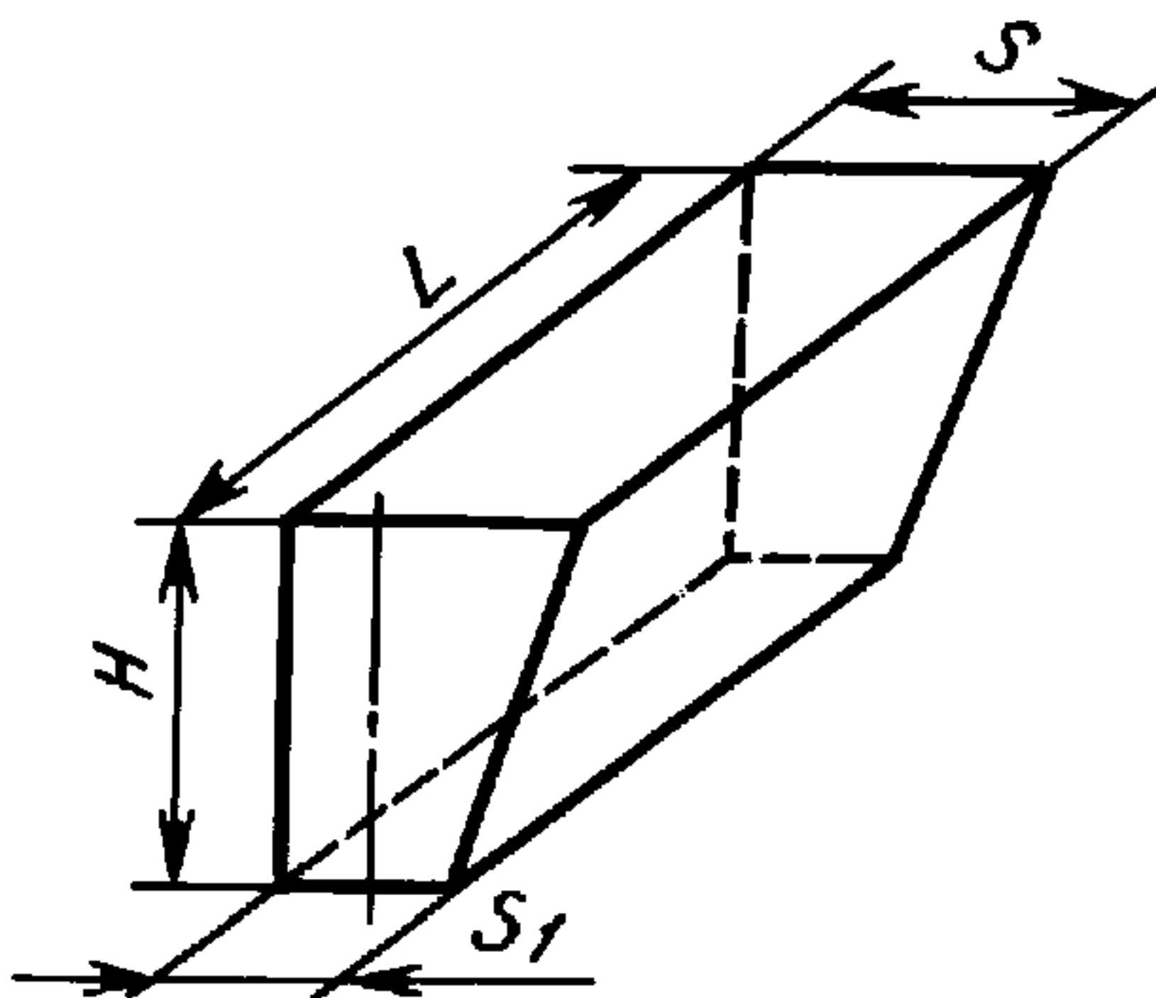
Рисунок 2 — Клин ребровый односторонний
