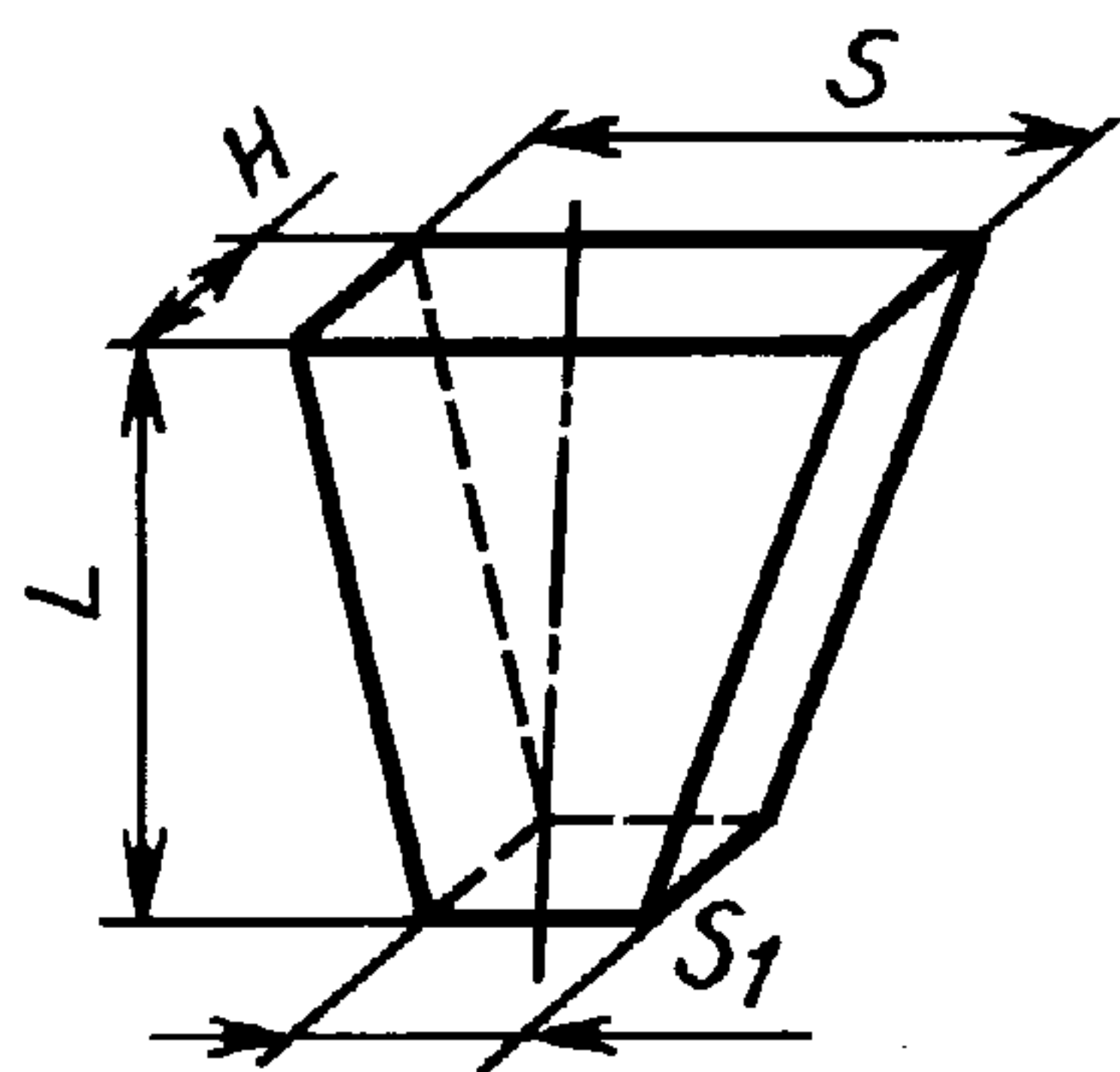
Рисунок 7 — Клин трапецеидальный двусторонний
