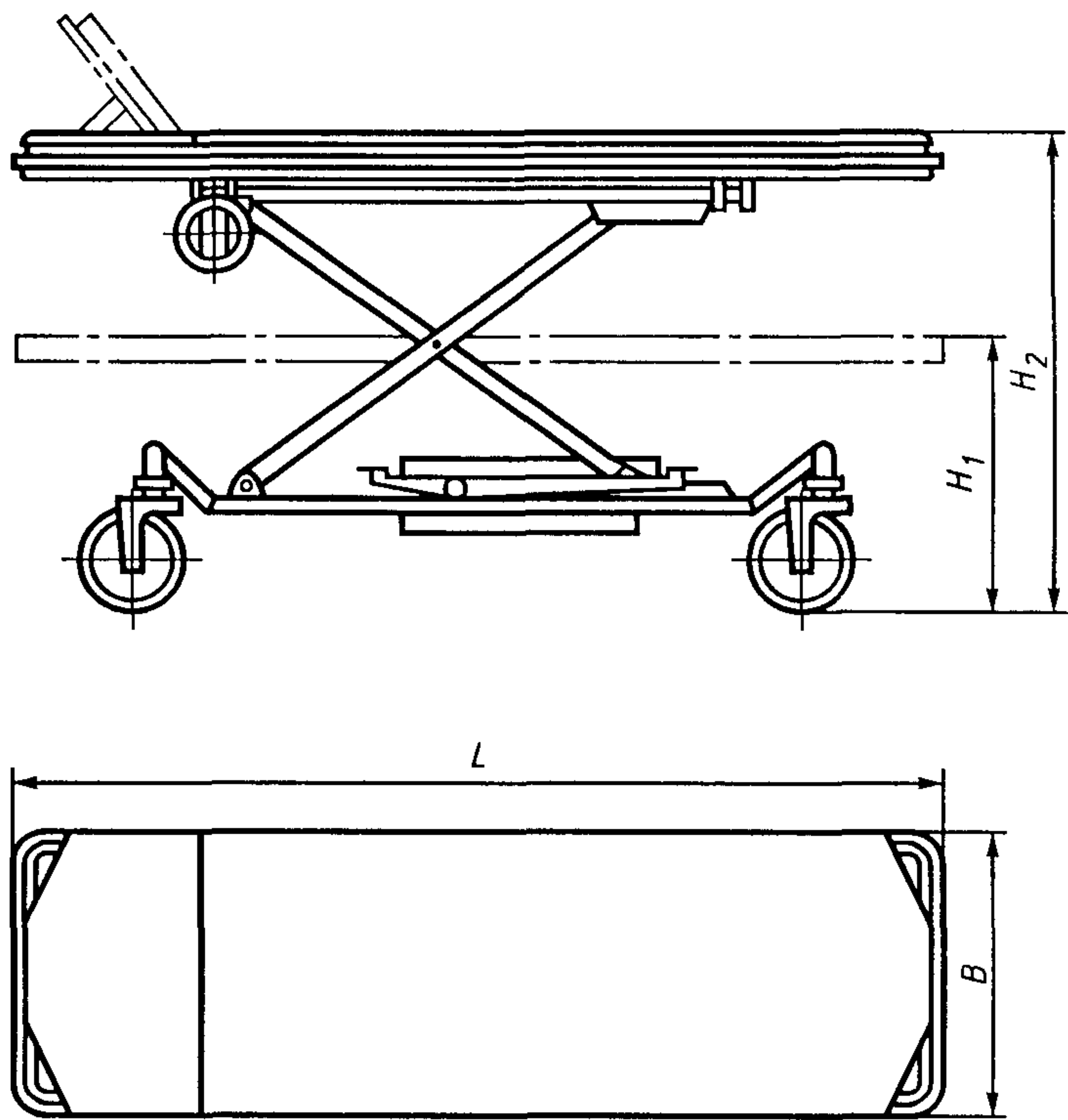
Рисунок А.1 — Тележка с подъемной панелью
