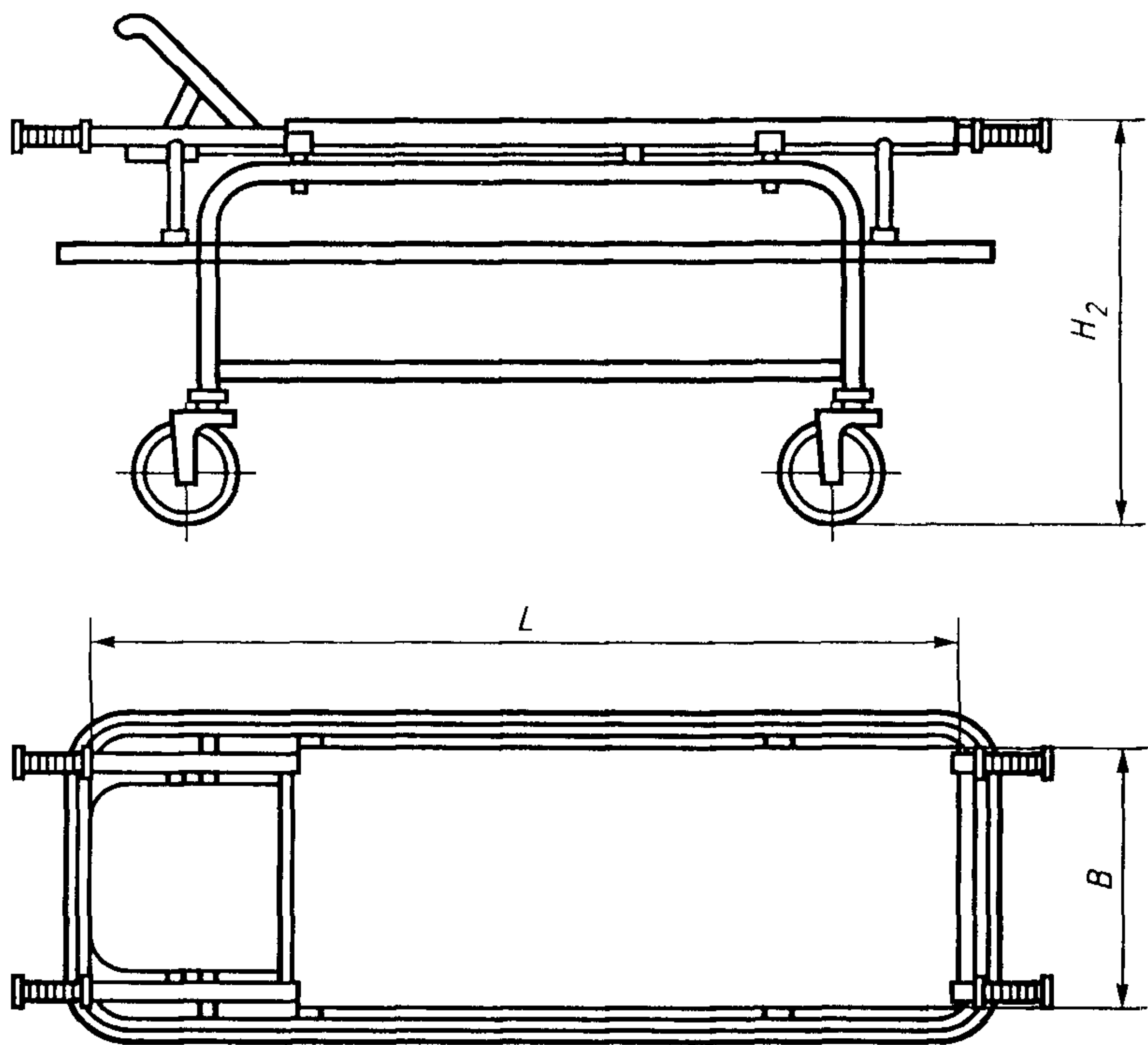
Рисунок А.2 — Тележка со съемной панелью (носилками)
