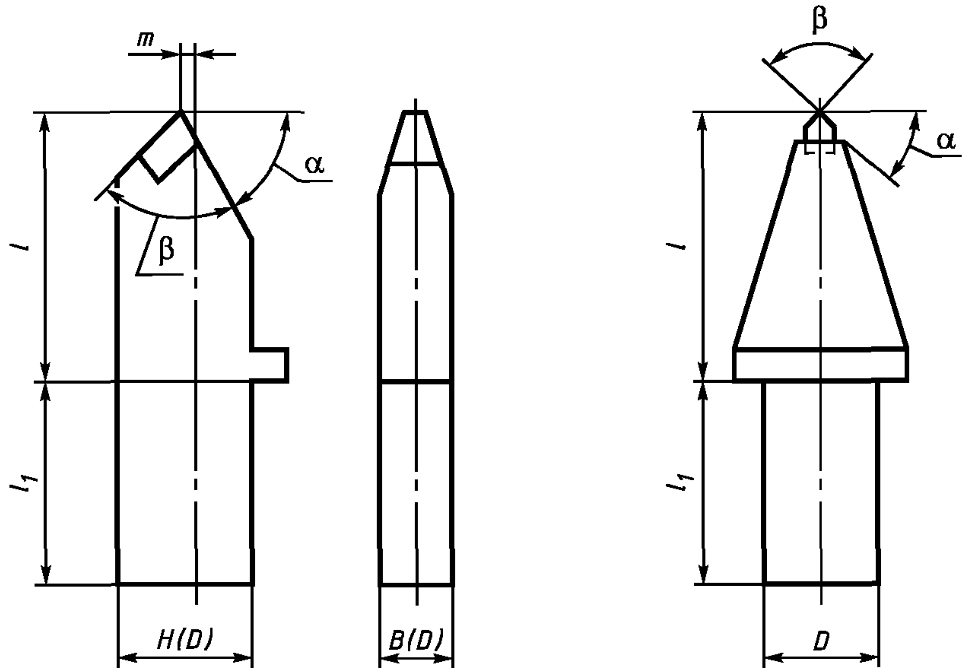
Рисунок 2 — Резец исполнения ТН
