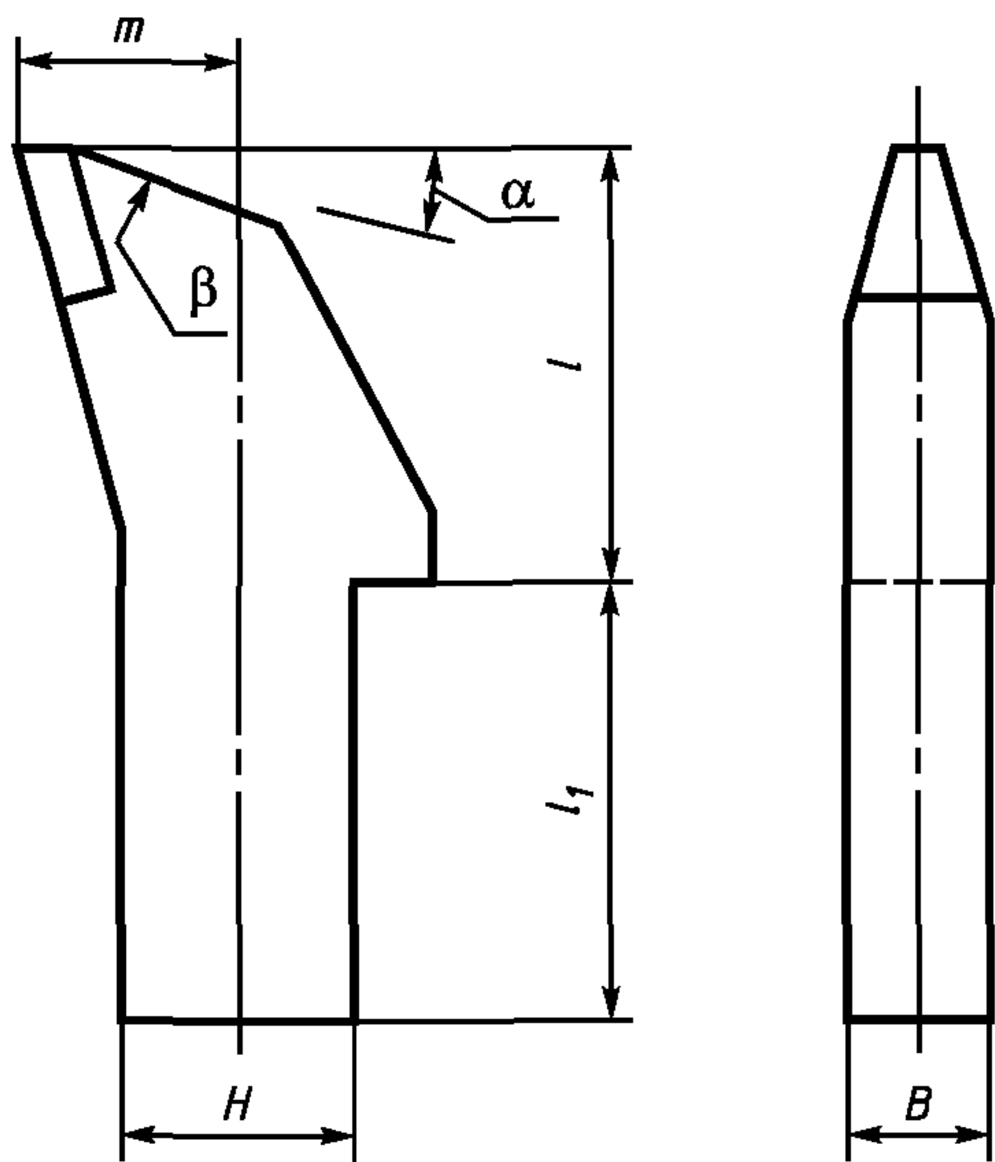
Рисунок 1 — Резец типа Р
