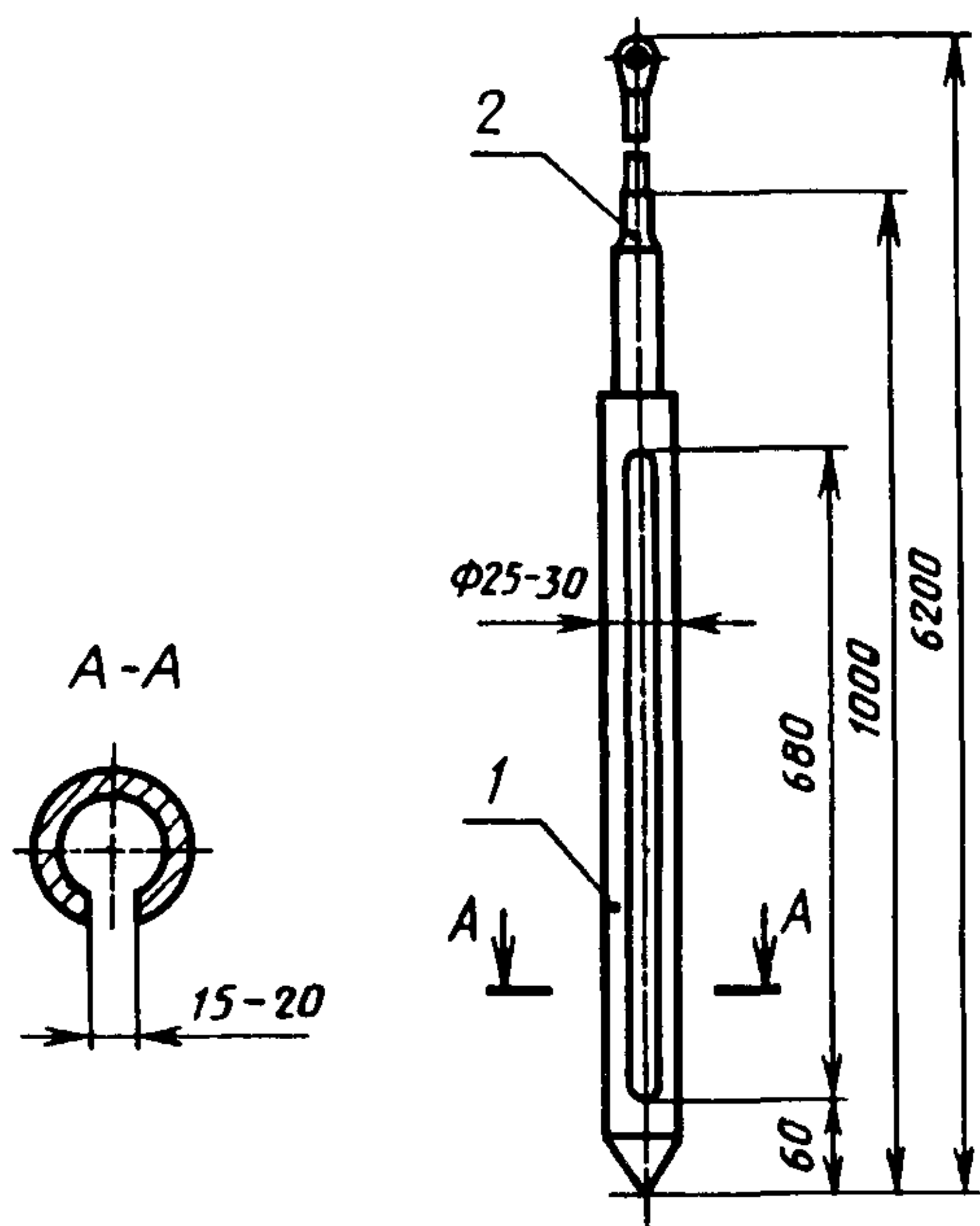
1 — корпус, 2 — держатель с заземлением
