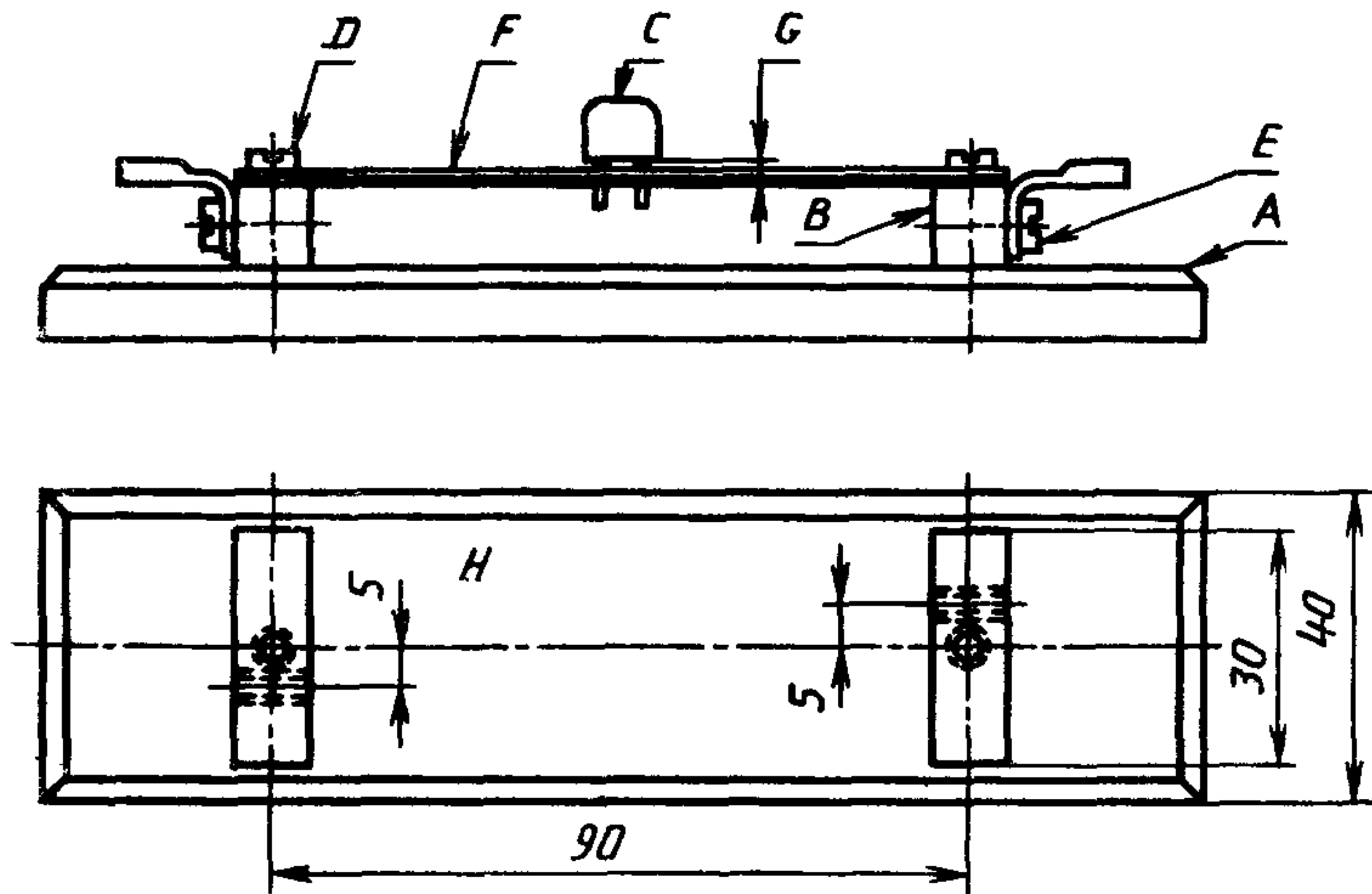
Размеры в миллиметрах
