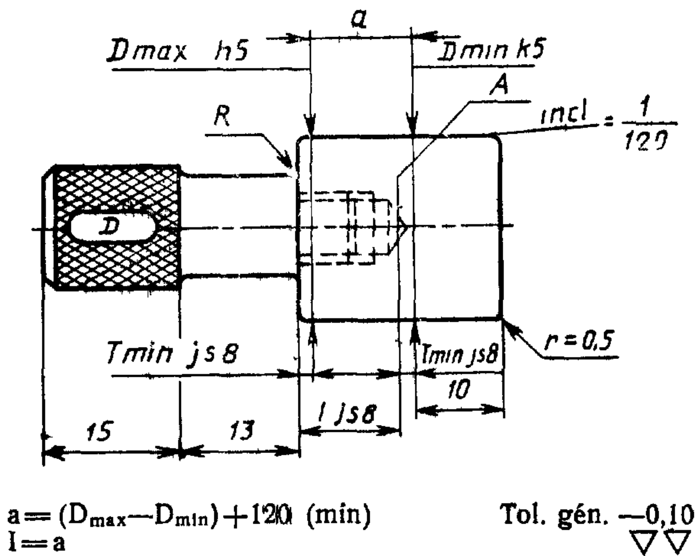
Calibre vérificateur de référence Contrôle du diamètre à l'entrée de la chambre D
