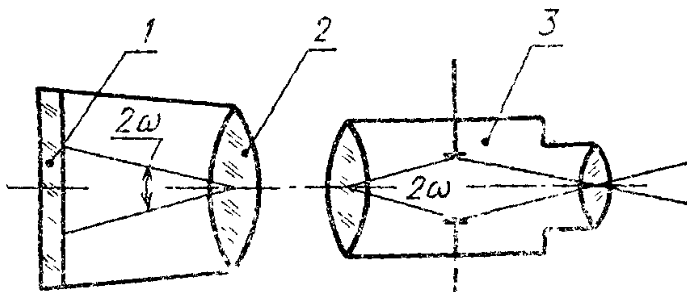
1 — шкала; 2 — широкоугольный объектив коллиматора; 3 — испытуемый прибор
