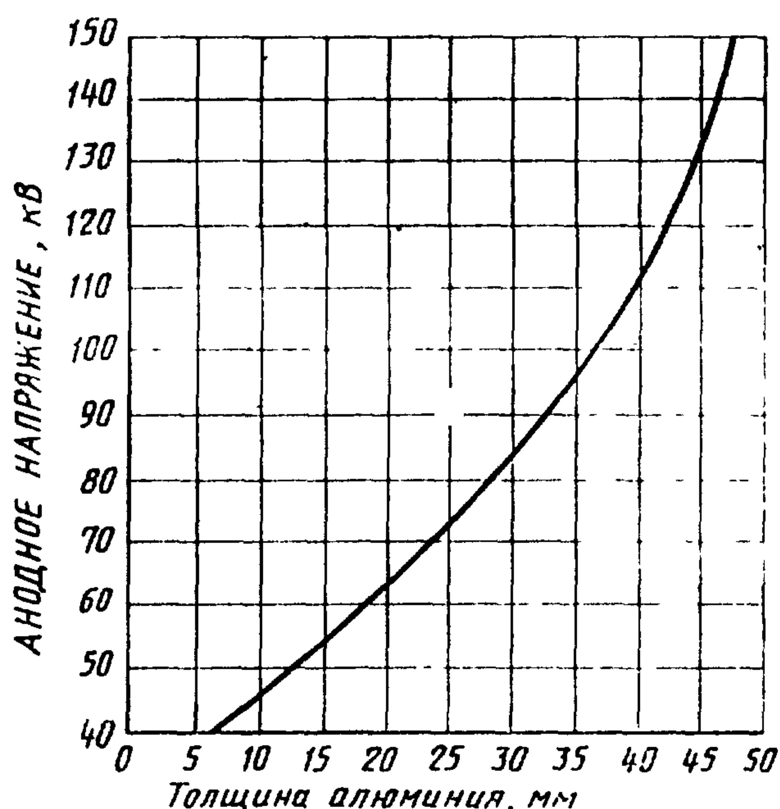
Рисунок 101 — ОБЩАЯ ФИЛЬТРАЦИЯ для измерения ВОЗДУШНОЙ КЕРМЫ
