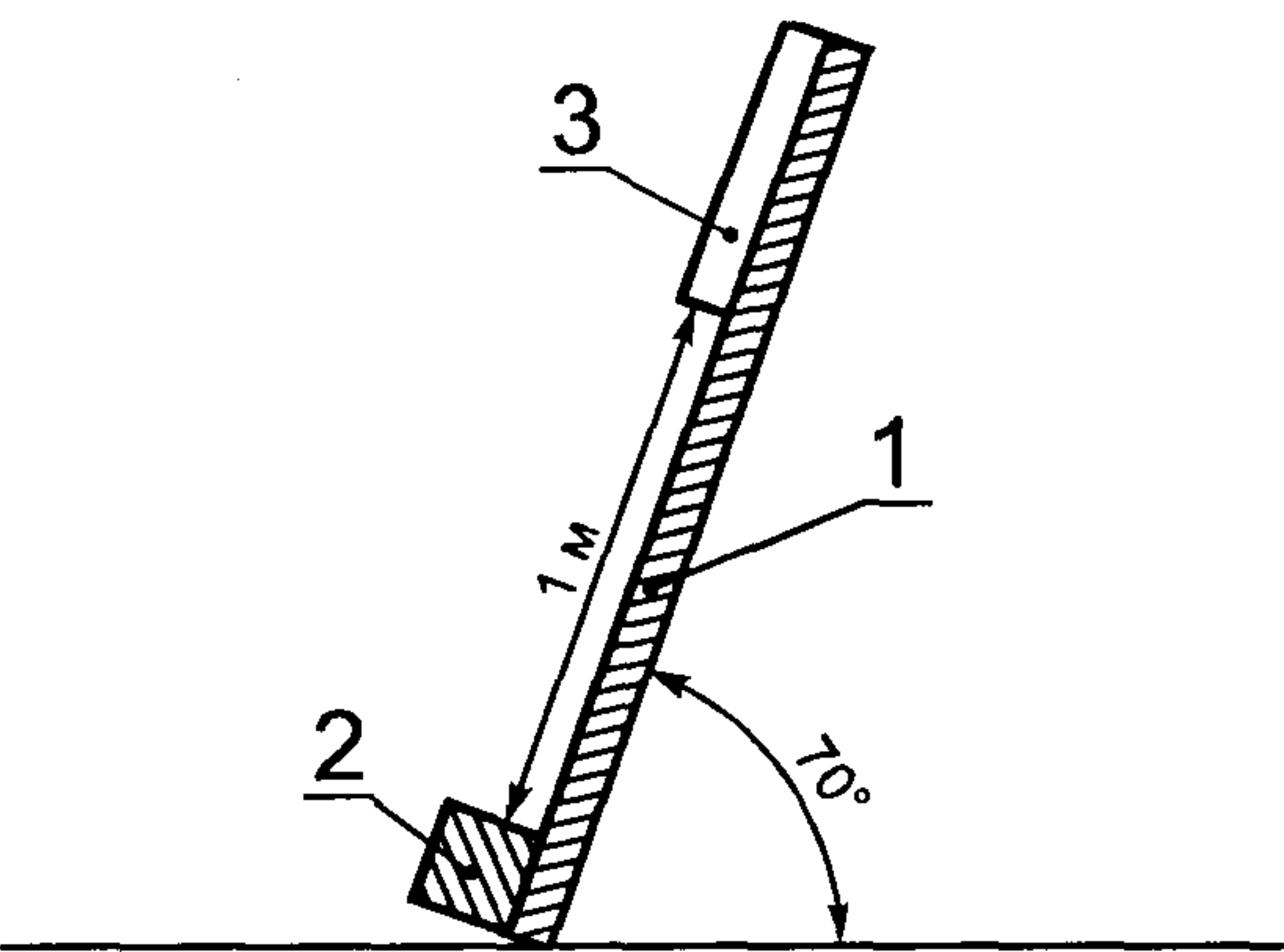
1 — гладкая наклонная плоскость; 2 — упорная колодка; 3 — испытуемая ПОДУШКА
