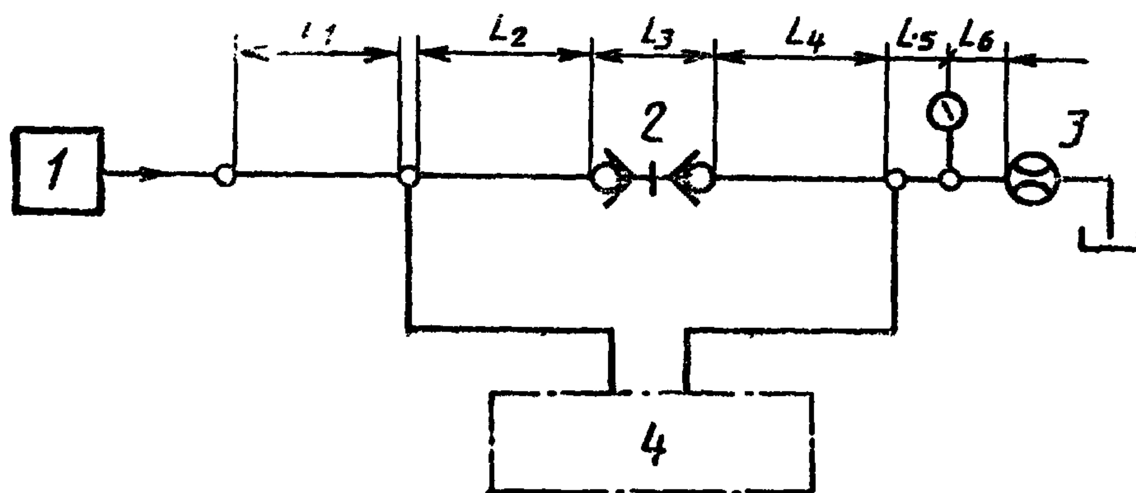
Принципиальная схема испытательной установки
