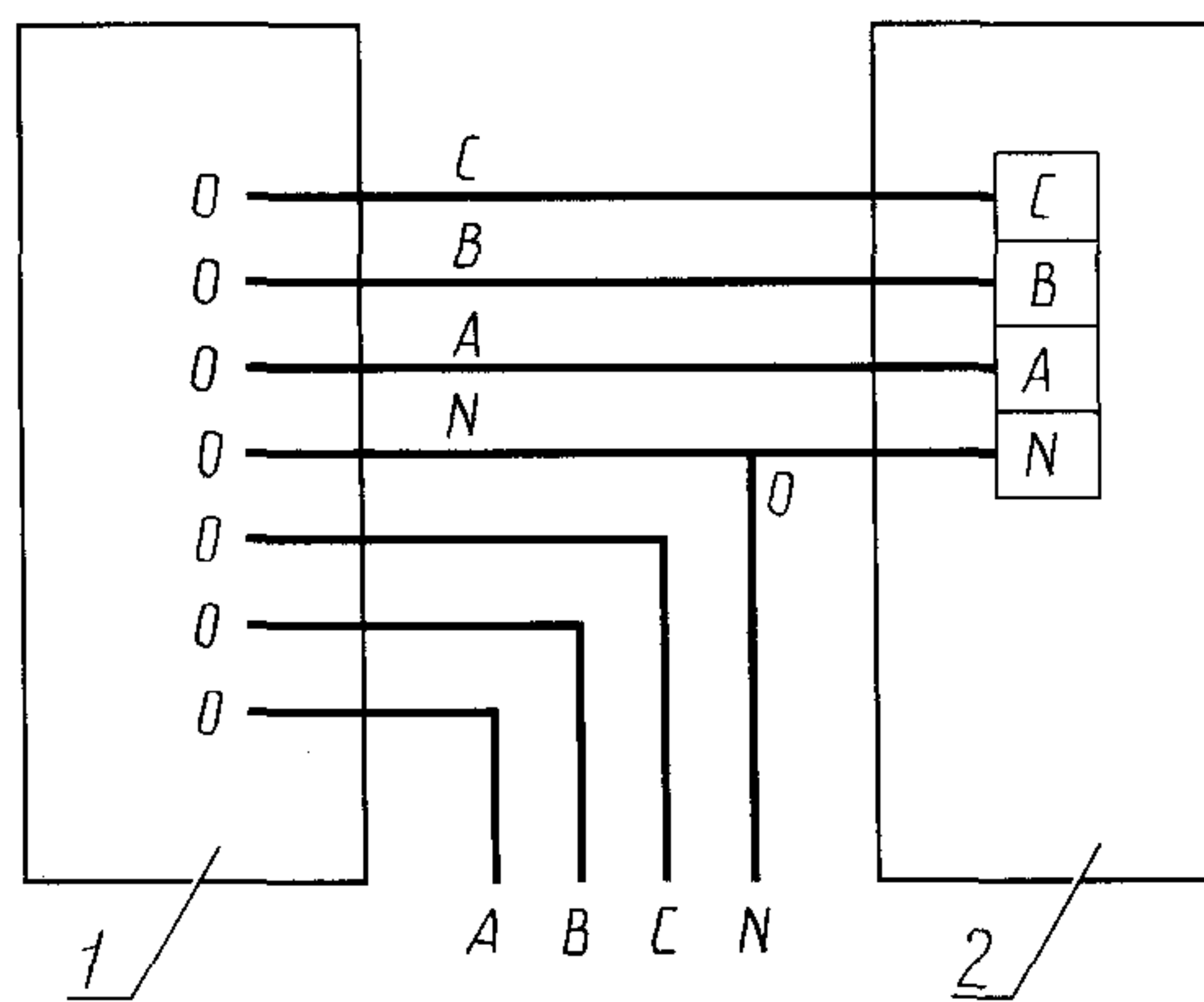
Схема подключения автотрансформатора к оборудованию
