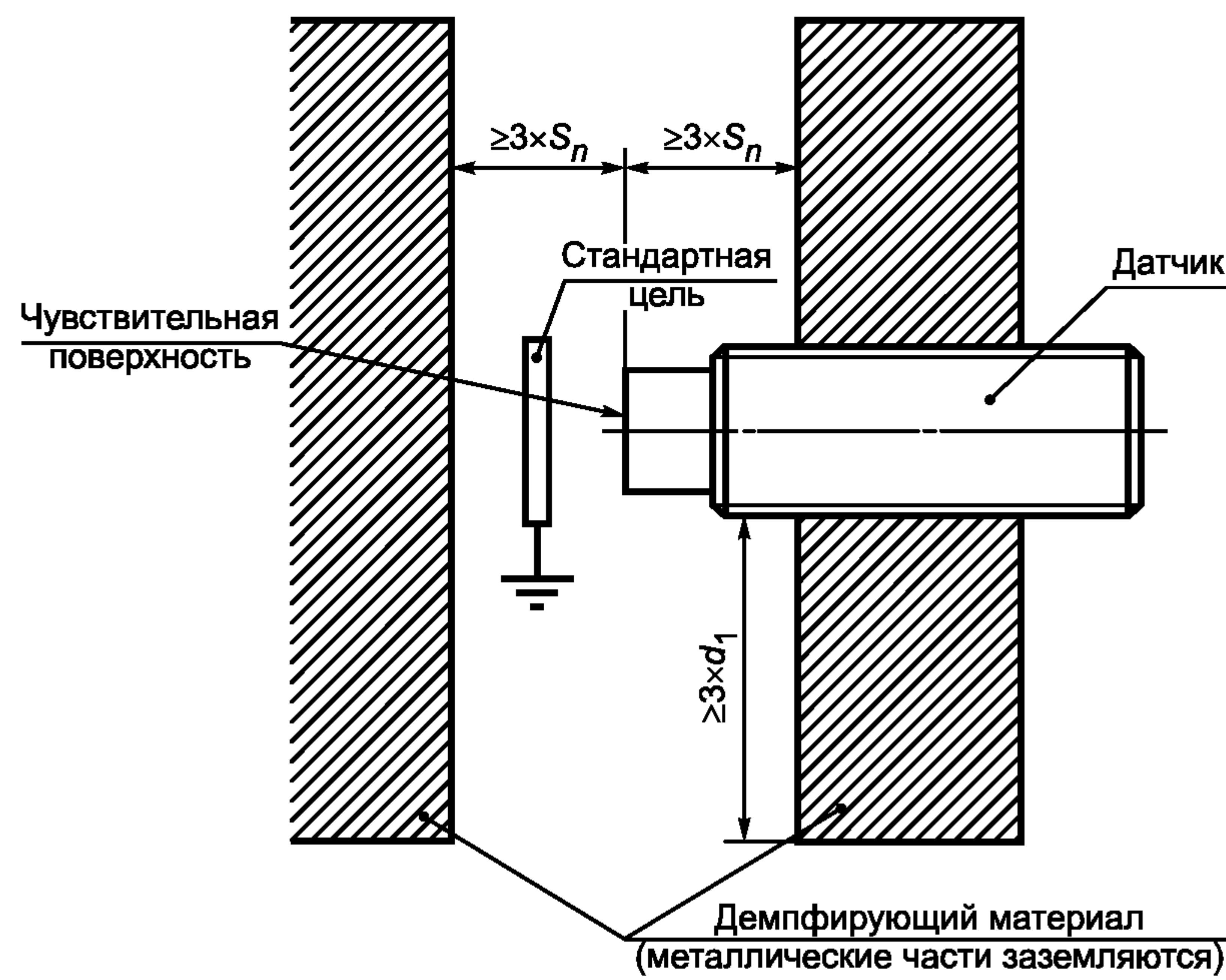
Рисунок А.2 (CA) — Установка (монтаж)
