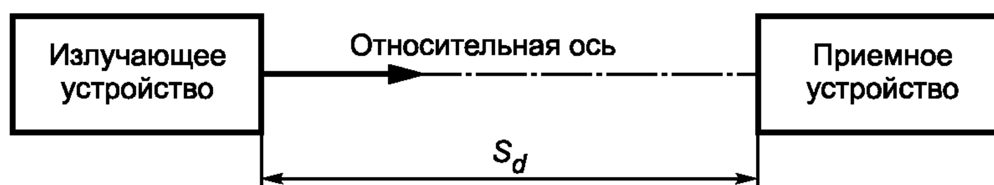
Рисунок 1а — Датчик типа Т. Излучающее устройство и приемное устройство — фотоэлектрический барьер
