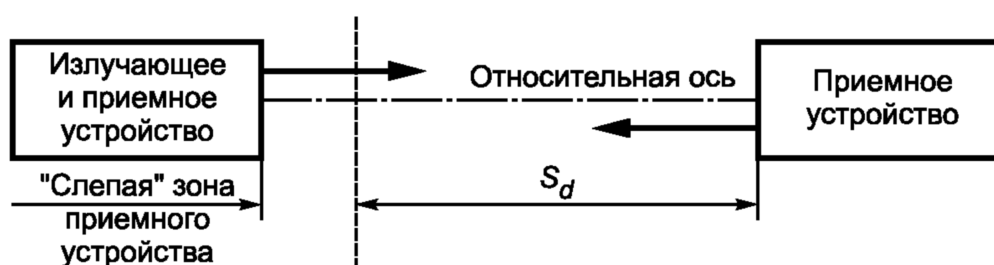
Рисунок 1b — Датчик типа R. Излучающее устройство, приемное устройство и рефлектор — фотоэлектрическое отражение
