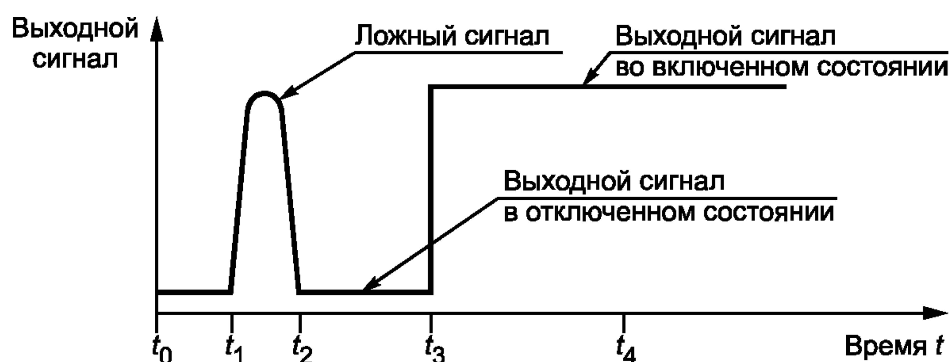
Рисунок 7а — Коммутационный элемент во включенном состоянии
