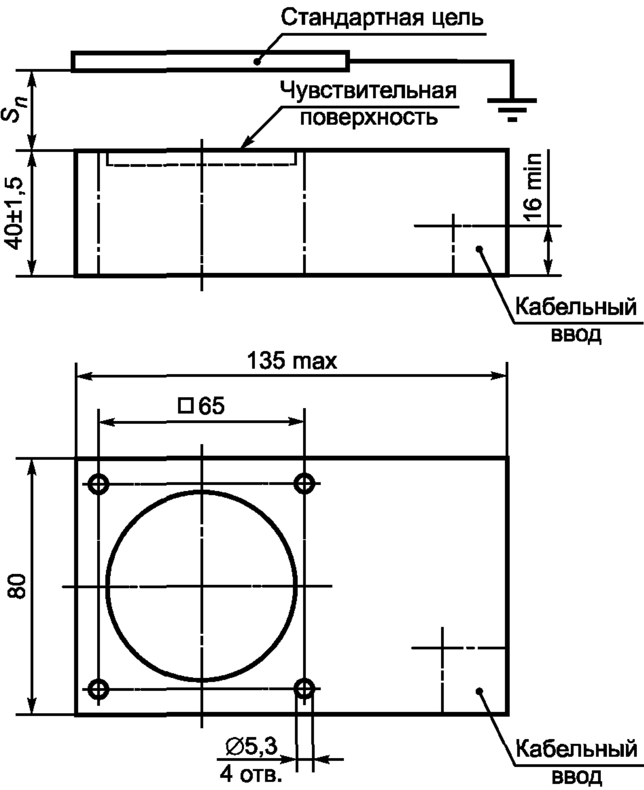
Рисунок А.1 (CD) — Габаритные размеры
