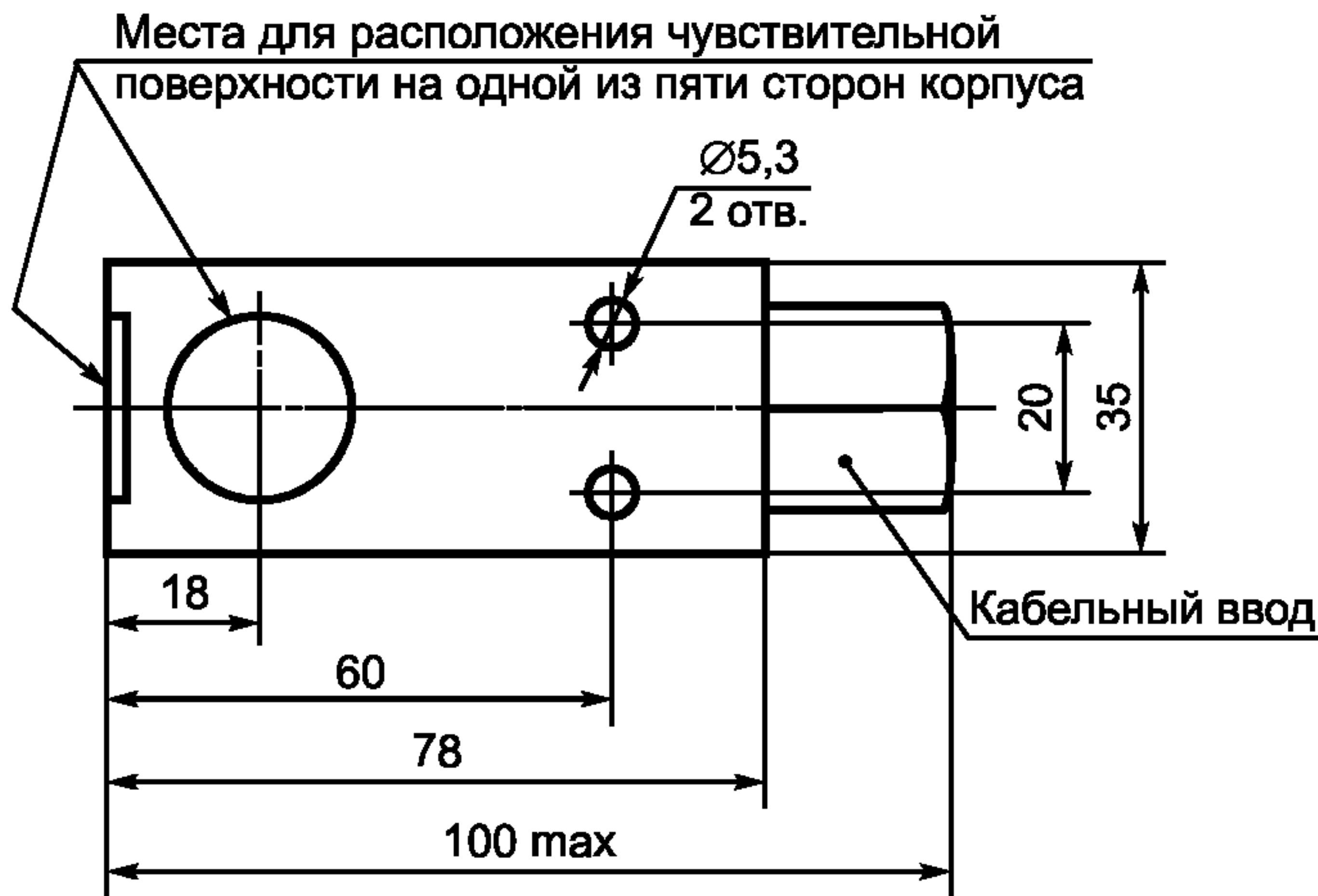
Рисунок А.1.2 (ІС) — Габаритные размеры
