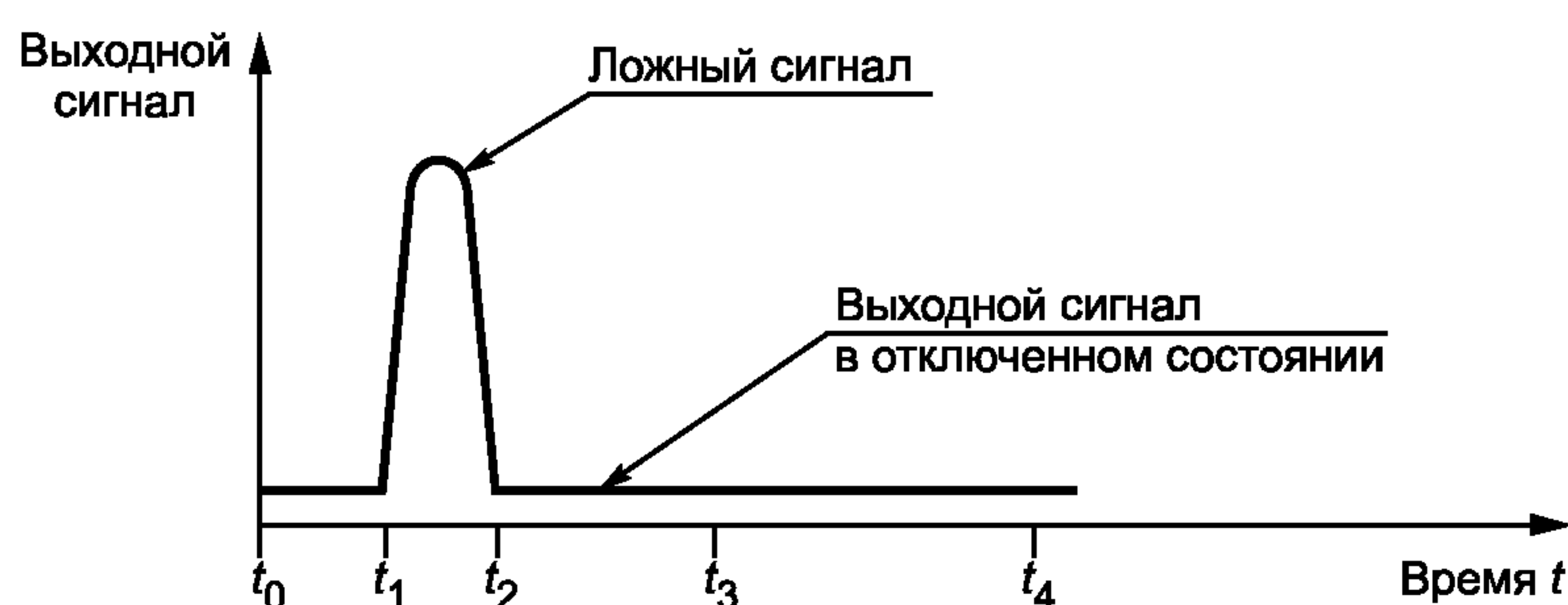
Рисунок 7б — Коммутационный элемент в выключенном состоянии
