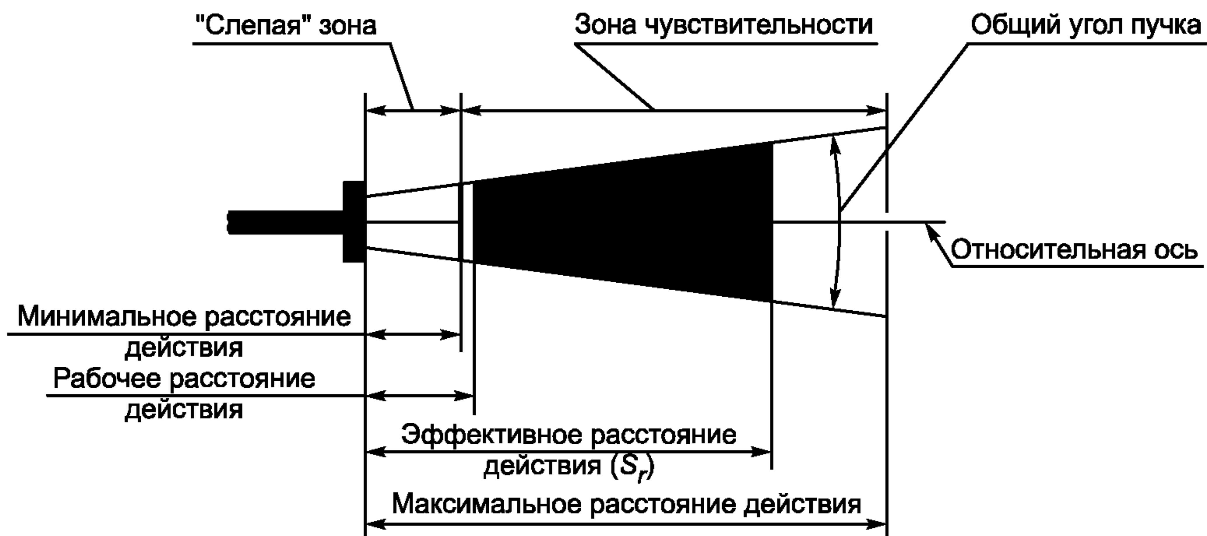
Рисунок 2 — Расстояния дальности действия ультразвукового датчика
