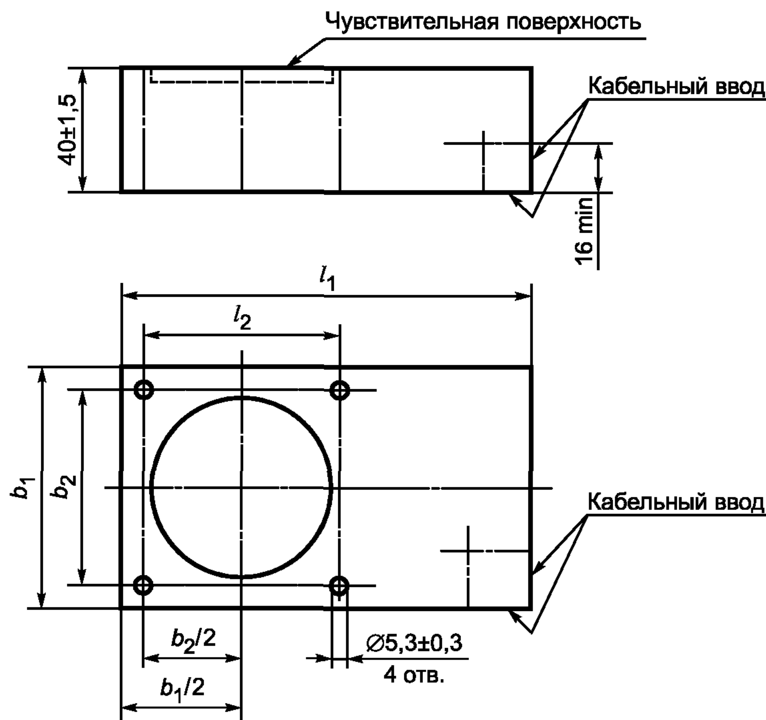
Рисунок А.1 (ID) — Габаритные размеры
