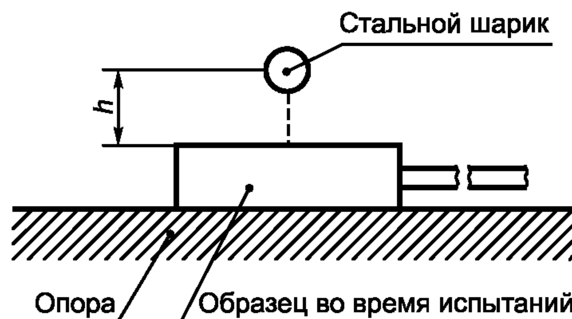
Рисунок В.2 — Испытательное устройство
