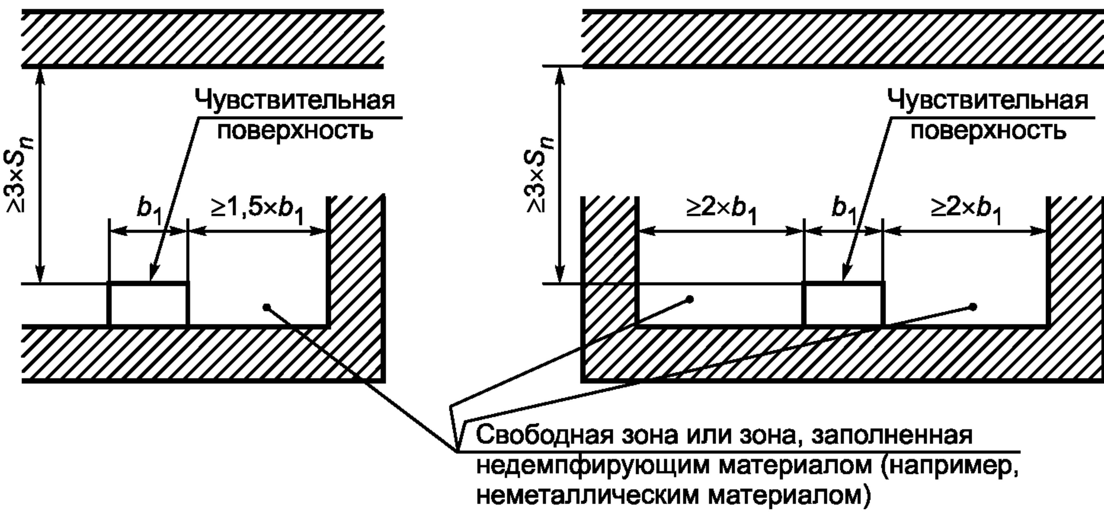
Рисунок А.2 (ID) — Установка датчиков типа I2D в демпфирующий материал
