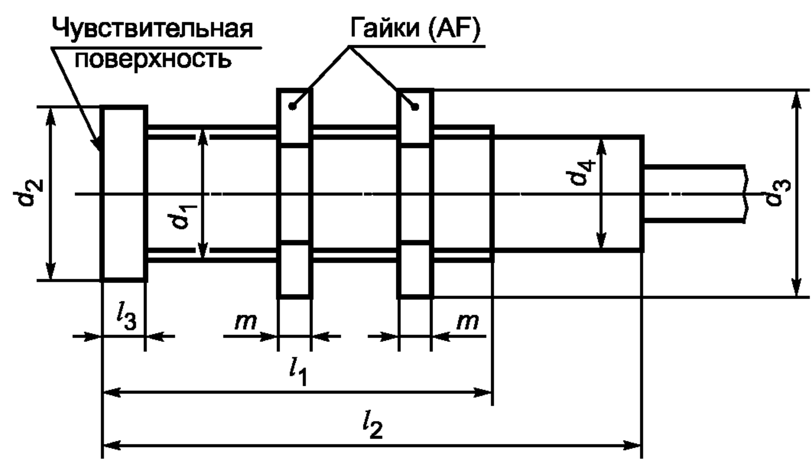
Рисунок A.1 (UA) — Габаритные размеры
