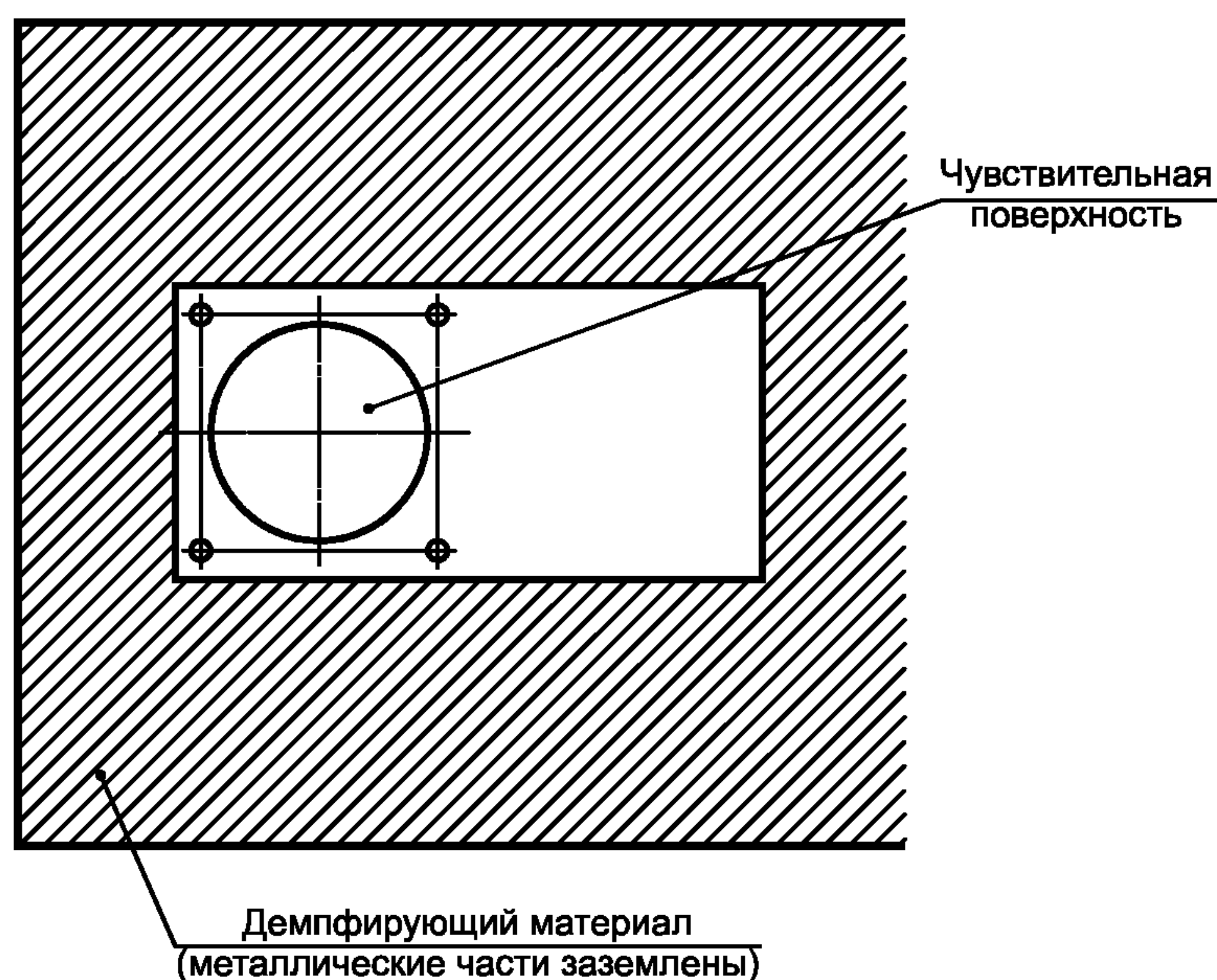
Рисунок A.2 (CD) — Установка (монтаж)
