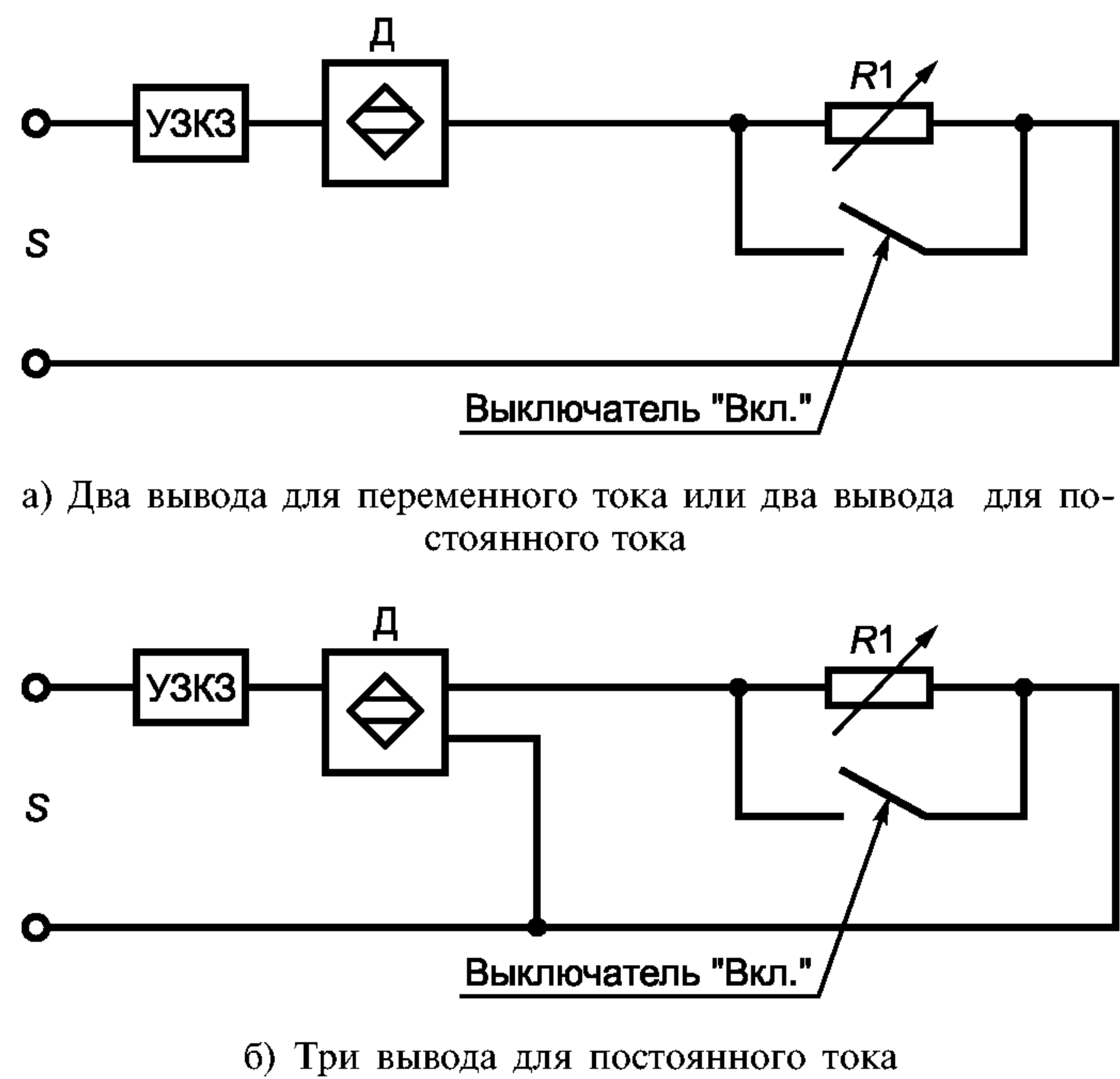
Рисунок 10 — Схема испытаний на короткое замыкание (см. 8.3.4.2)
