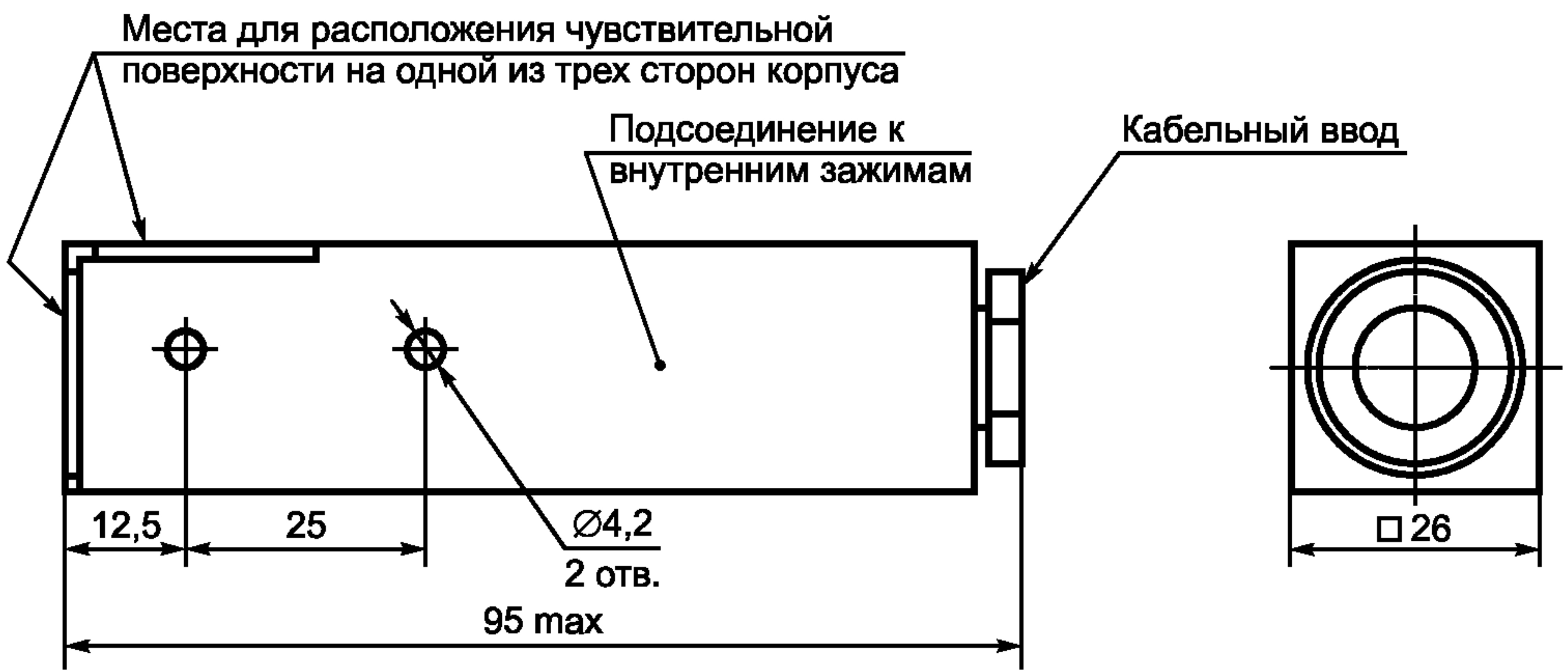
Рисунок А.1 (ІС) — Габаритные размеры
