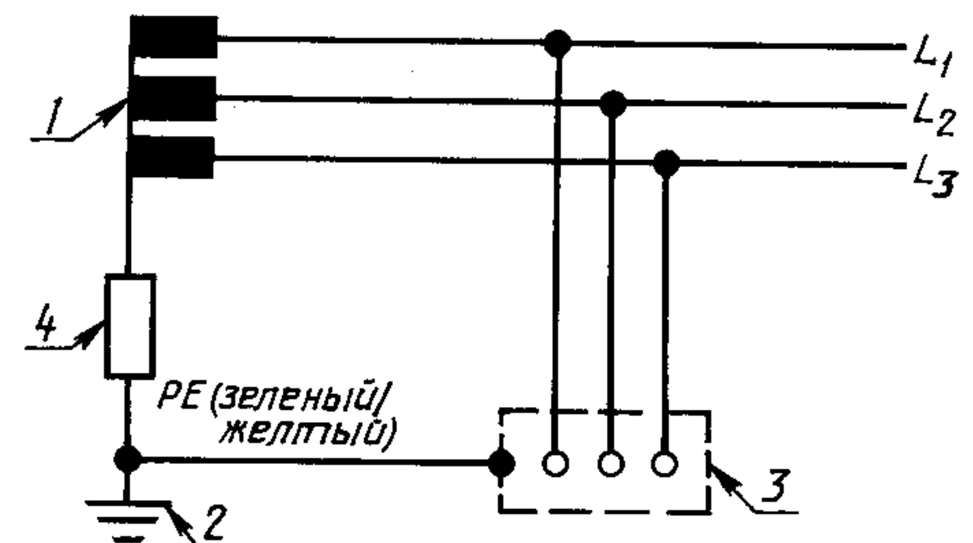
1 — точка заземления энергосистемы; 2 — земля; 3 — открытые проводящие части; 4 — заземляющее сопротивление (резистор или реактор); L_1, L_2, L_3 — фазные проводники энергосистемы; PE — защитный проводник
