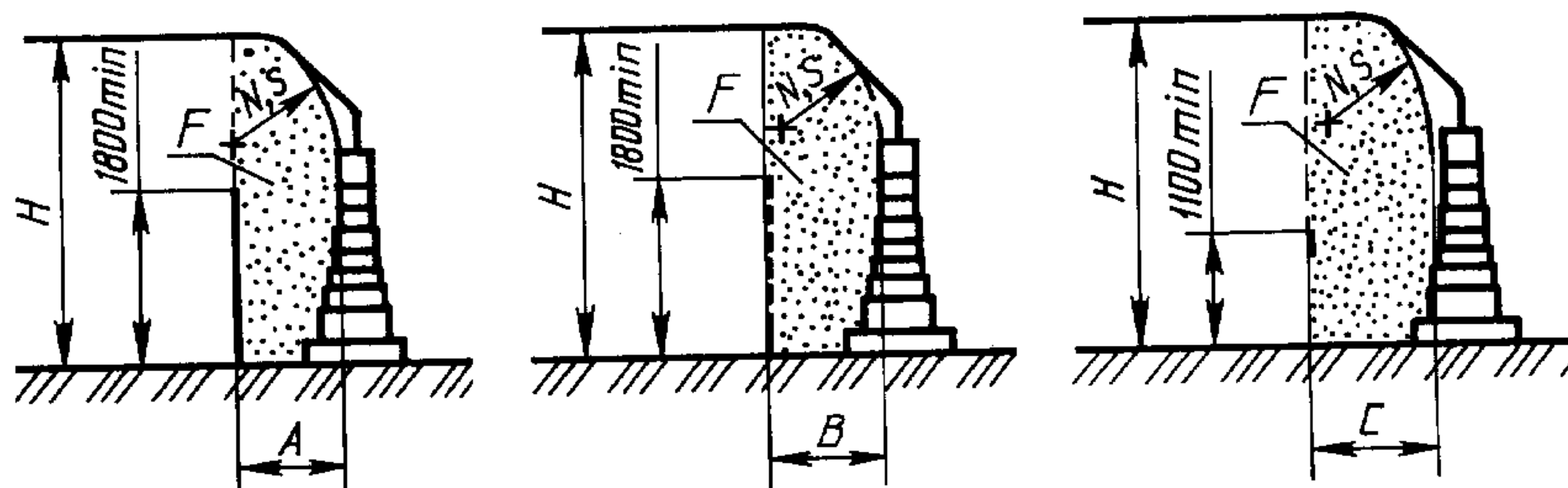
а) жесткое ограждение б) сетка или экран в) ограждение с поручнями, цепями или канатом
