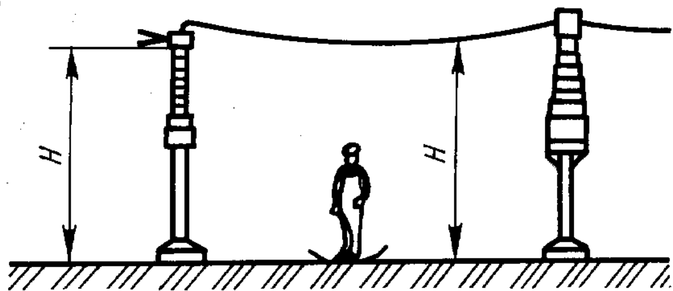
H — минимальное расстояние между частями под напряжением над доступной зоной, указанное в таблице 6. Расстояние может быть увеличено, чтобы учесть условия, указанные в 7.1 и 7.3 Рисунок 2 — Минимальная высота частей под напряжением над доступными поверхностями в наружных установках
