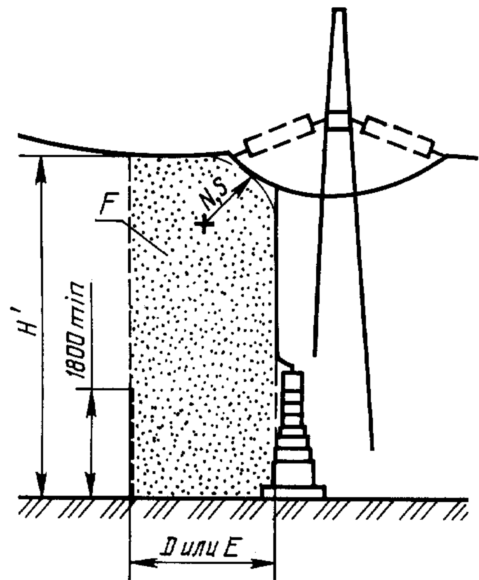
H' — минимальное расстояние для силовых воздушных линий; E — необходимые минимальные расстояния, указанные в таблице 6; N , S — см. таблицу 6; F — зона, в которой не должны находиться части под напряжением Рисунок 1 — Расстояния между частями под напряжением и наружным ограждением
