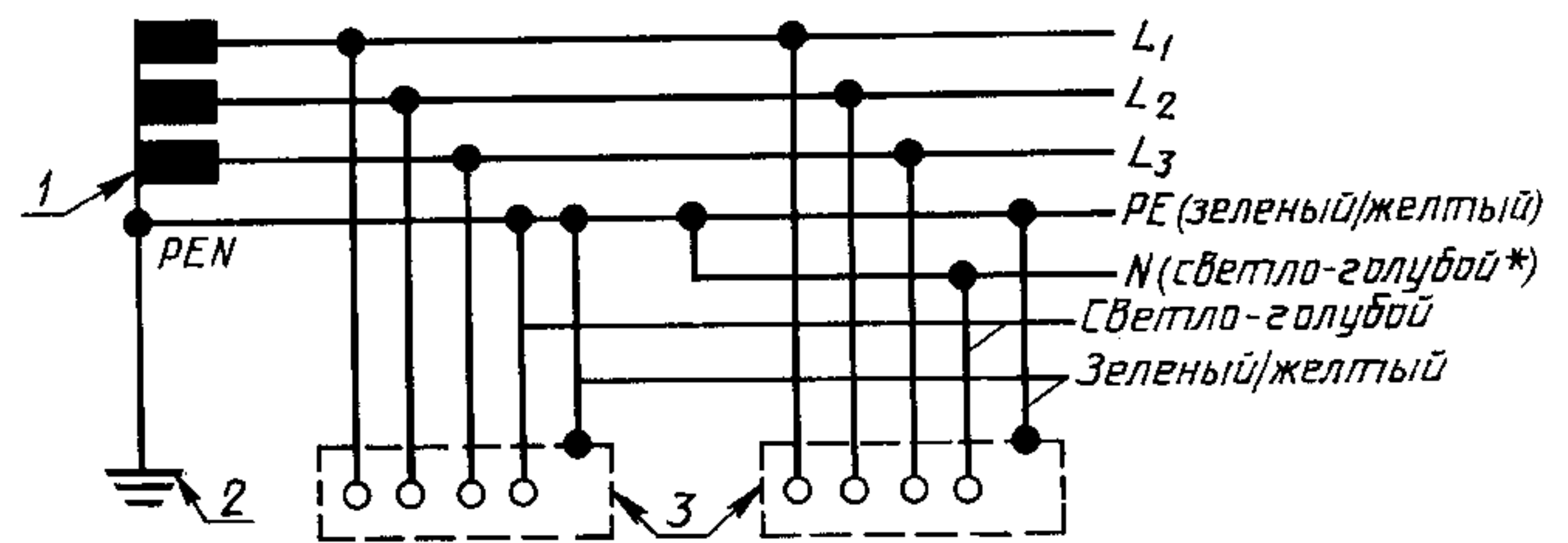
1 — точка заземления энергосистемы; 2 — земля; 3 — открытые проводящие части; L_1, L_2, L_3 — фазные проводники энергосистемы; N — нулевой проводник; PE — защитный проводник
