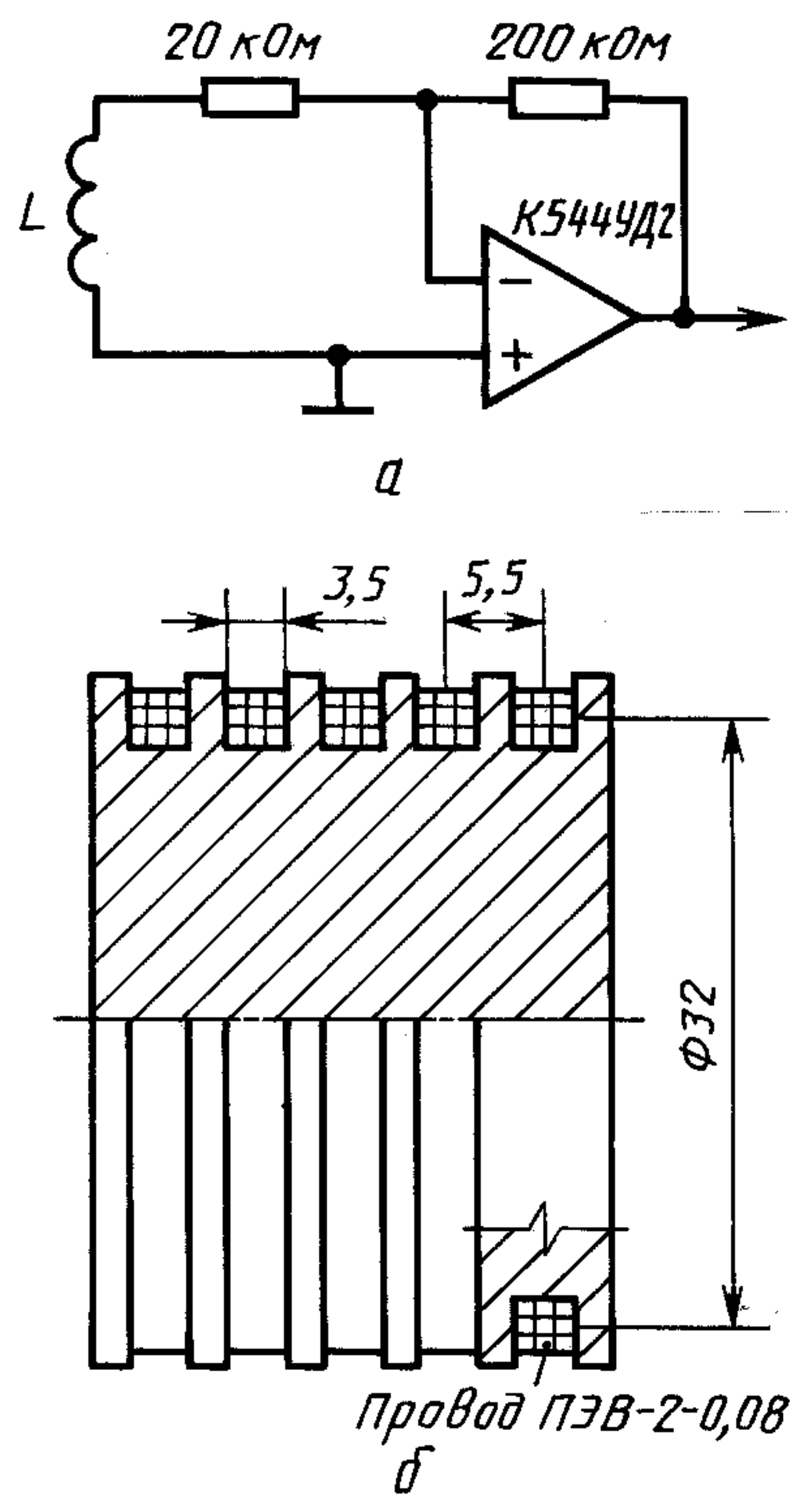
a — принципиальная электрическая схема; b — конструкция Параметры катушки число секций — 5; число витков в секции — 600; индуктивность катушки — 180—190 мГн
