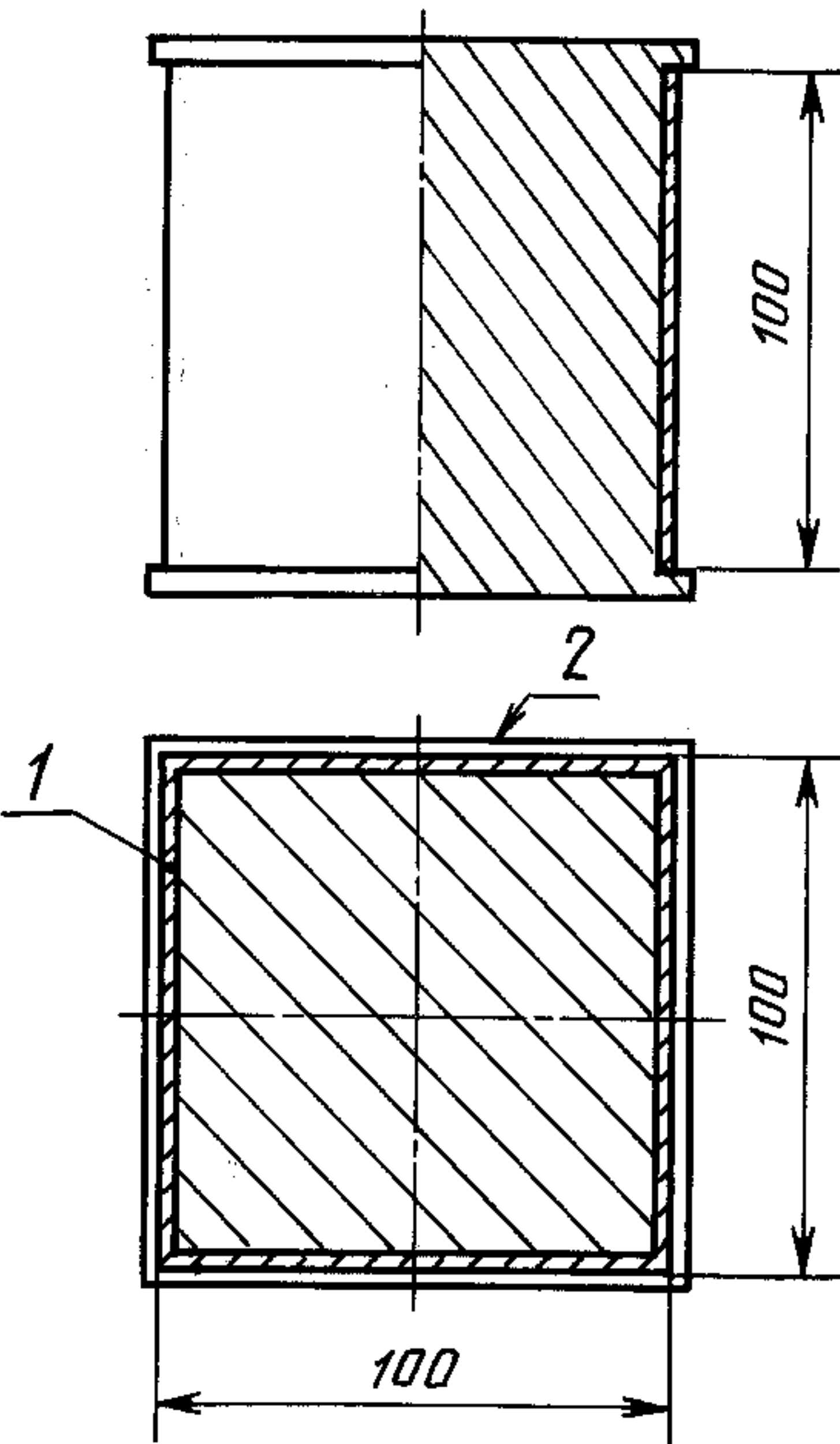
1 — катушка (число витков W=100 ); 2 — каркас
