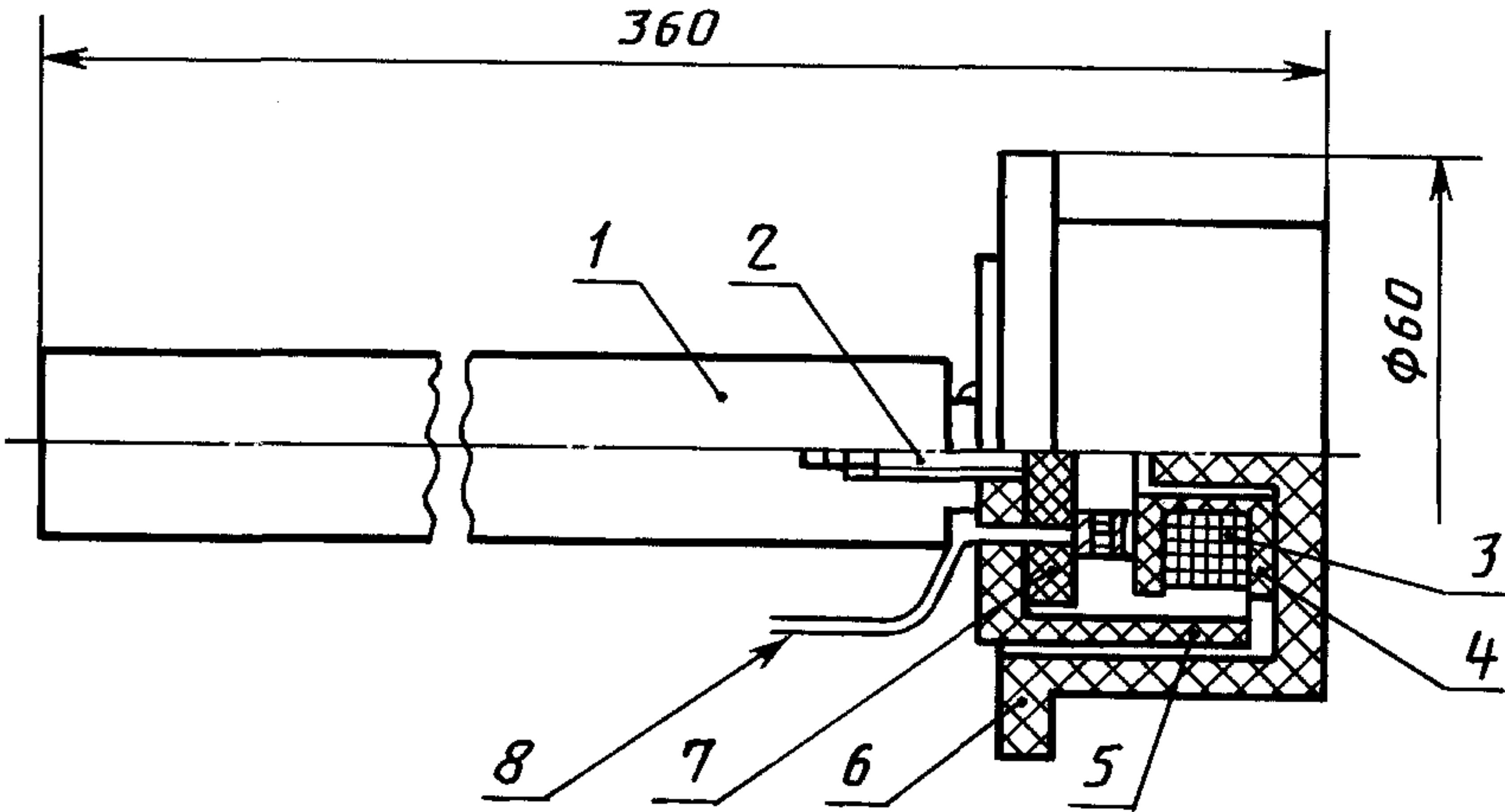
Локальный индукционный преобразователь ИП-1
