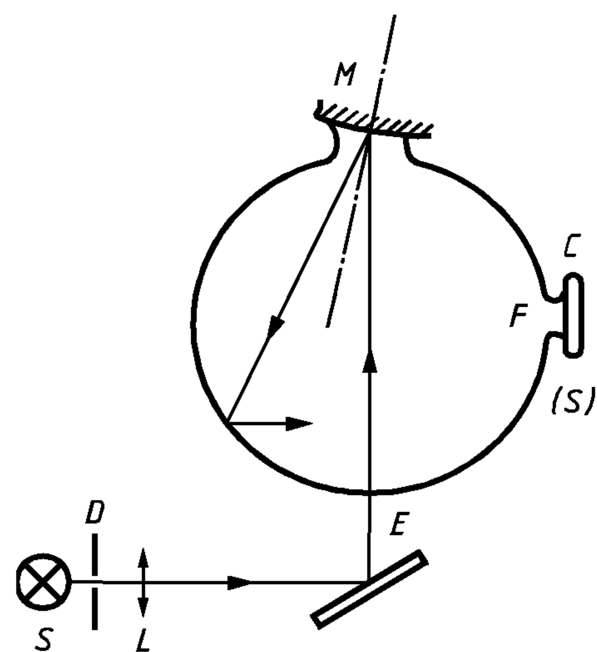
С — приемное устройство; D — диафрагма; E — окно входа; F — окно измерения; L — линза; M — окно для образца; S — источник света; (S) — светомерный шар
