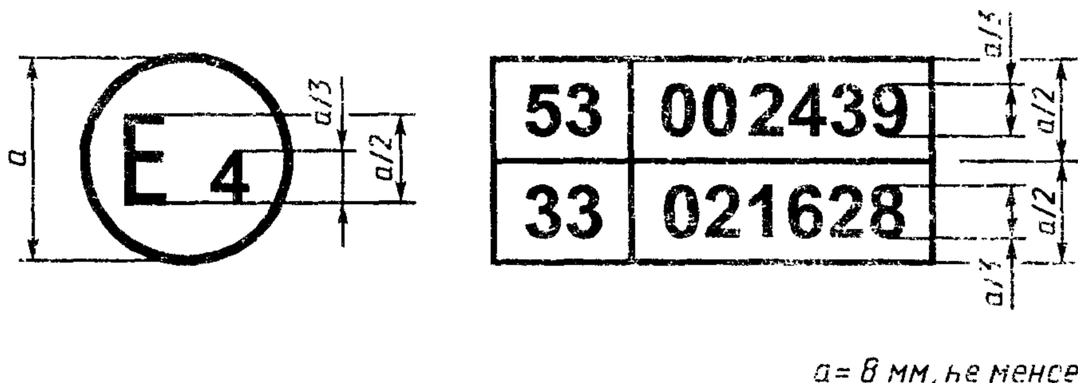
Образец В (см. 4.5 настоящих Правил)
