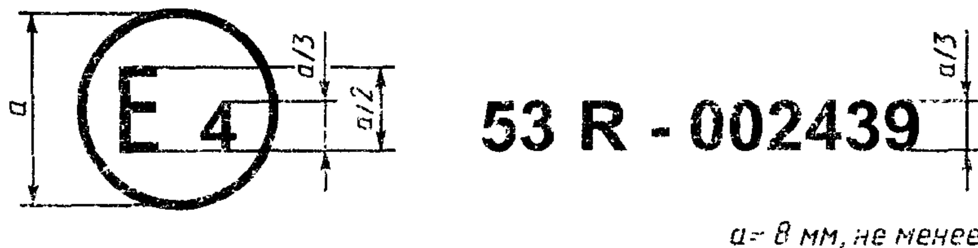
Образец А (см. 4.4 настоящих Правил)
