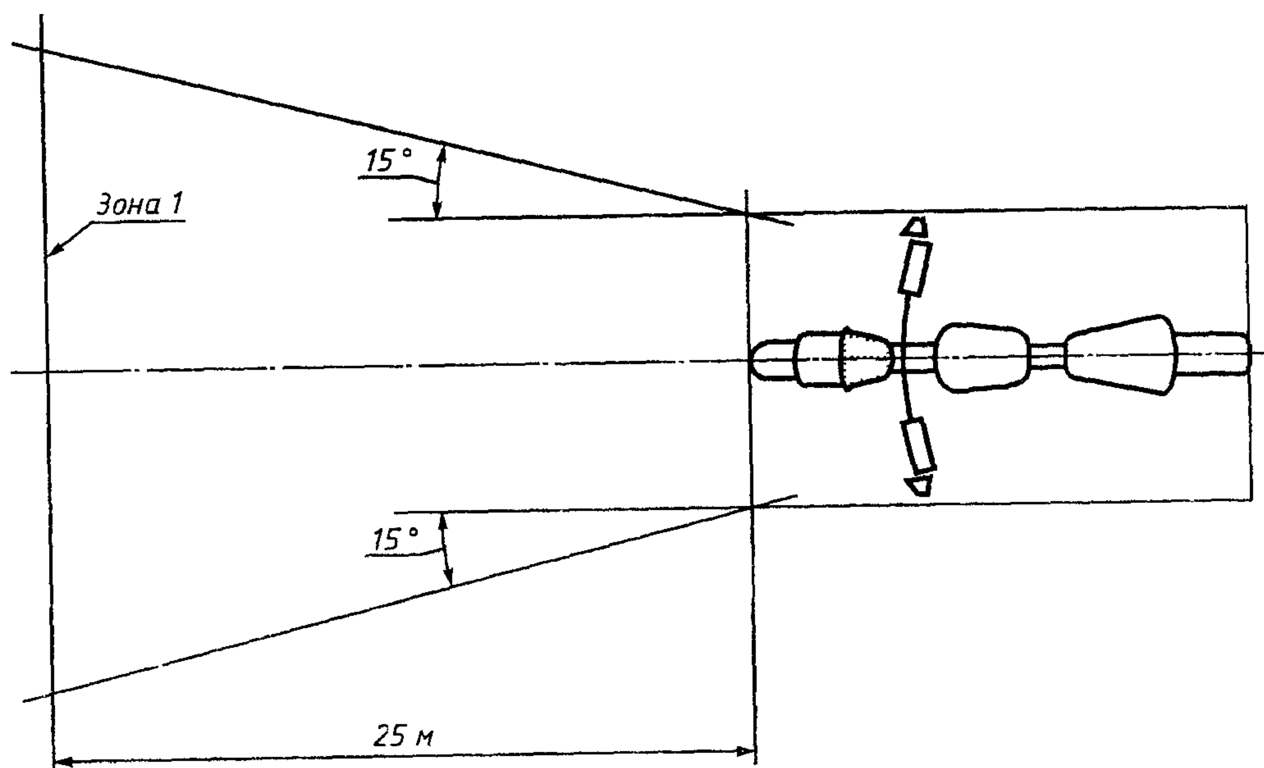
Рисунок 1 — Видимость красного огня спереди
