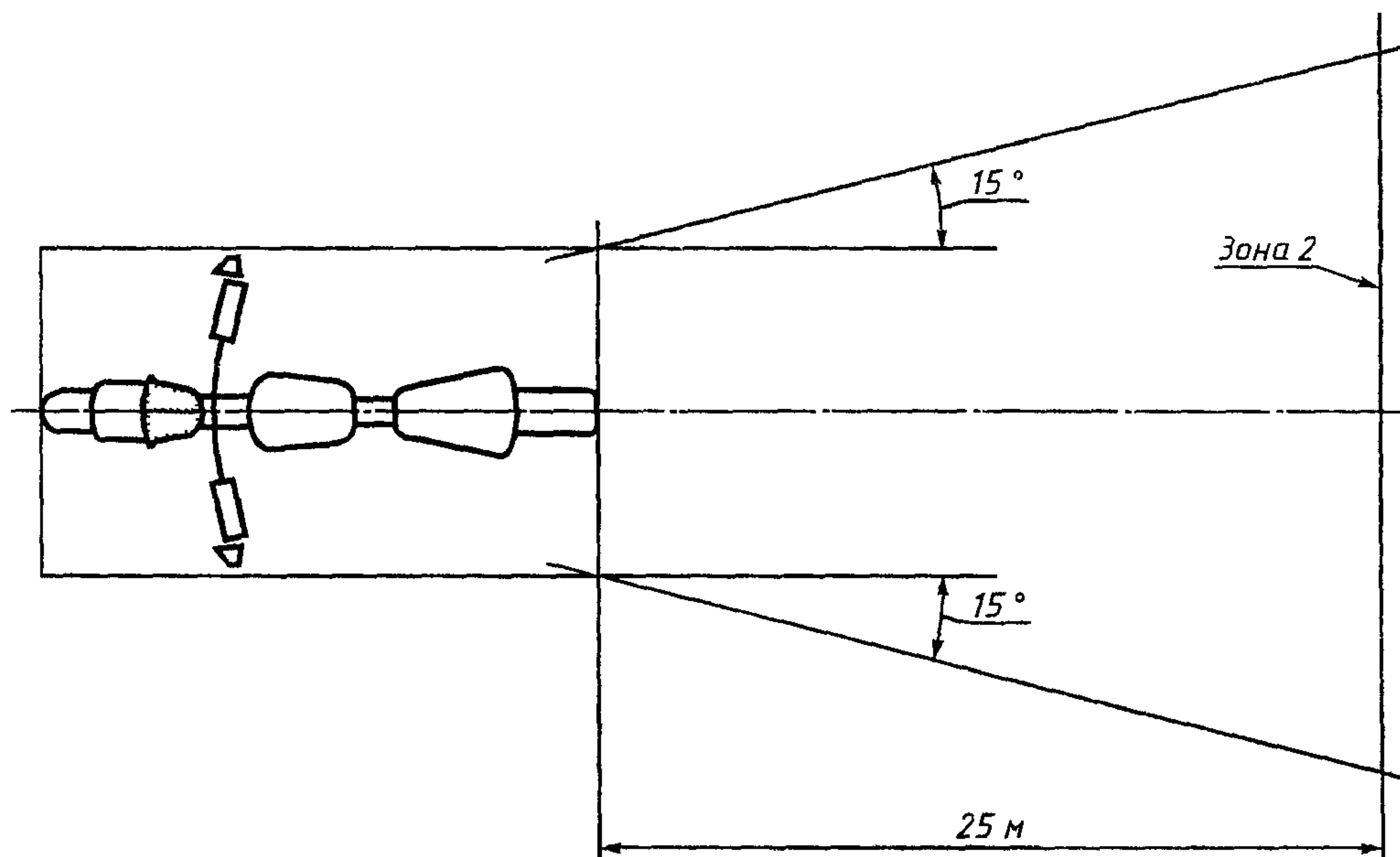
Рисунок 2 — Видимость белого огня сзади
