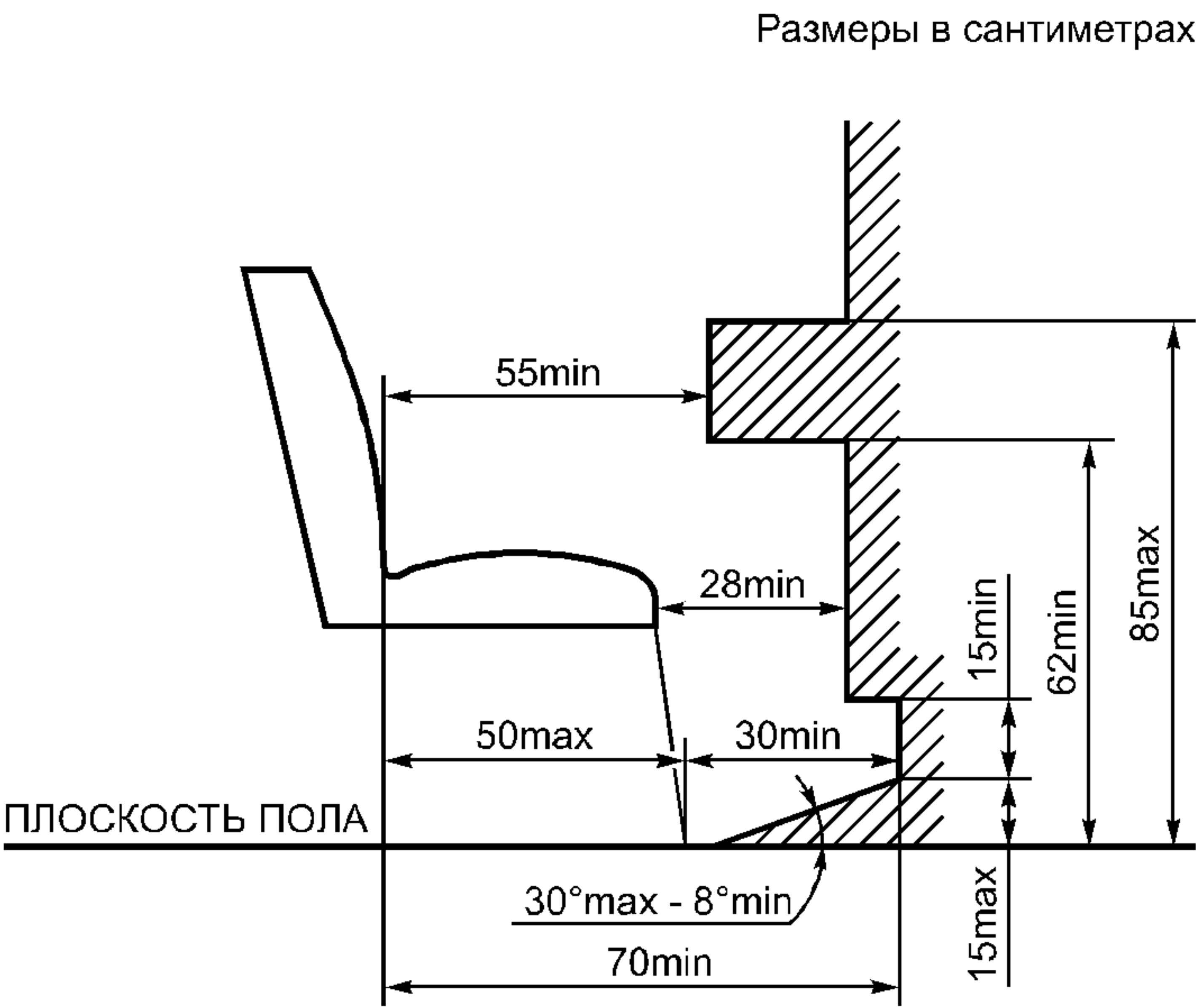
Рисунок 3.8 — Пространство для сидящих пассажиров (см. 5.7.8.5)
