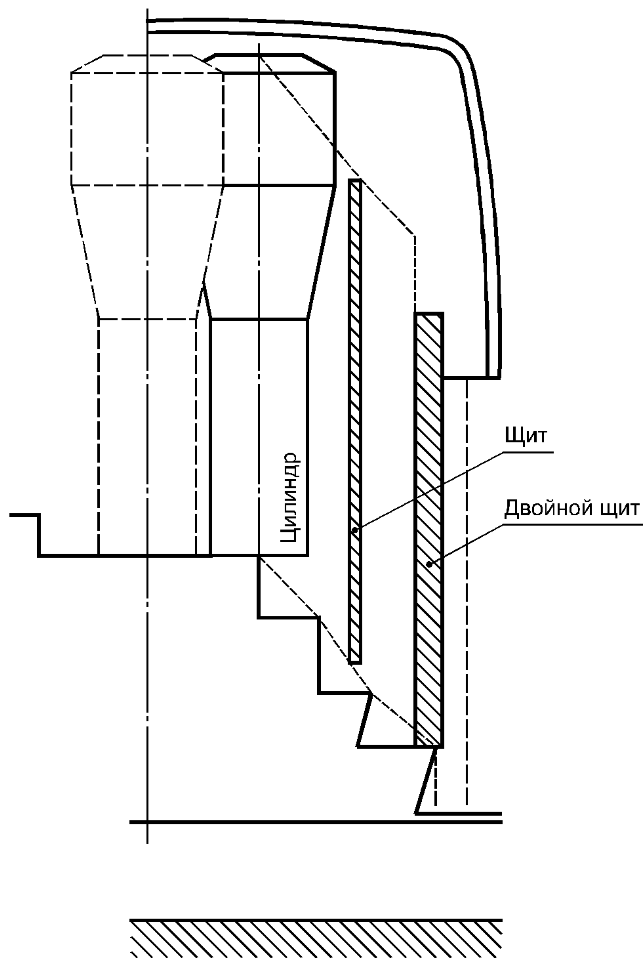
Рисунок 3.9 — Доступ к служебным дверям (см. 5.7.1)
