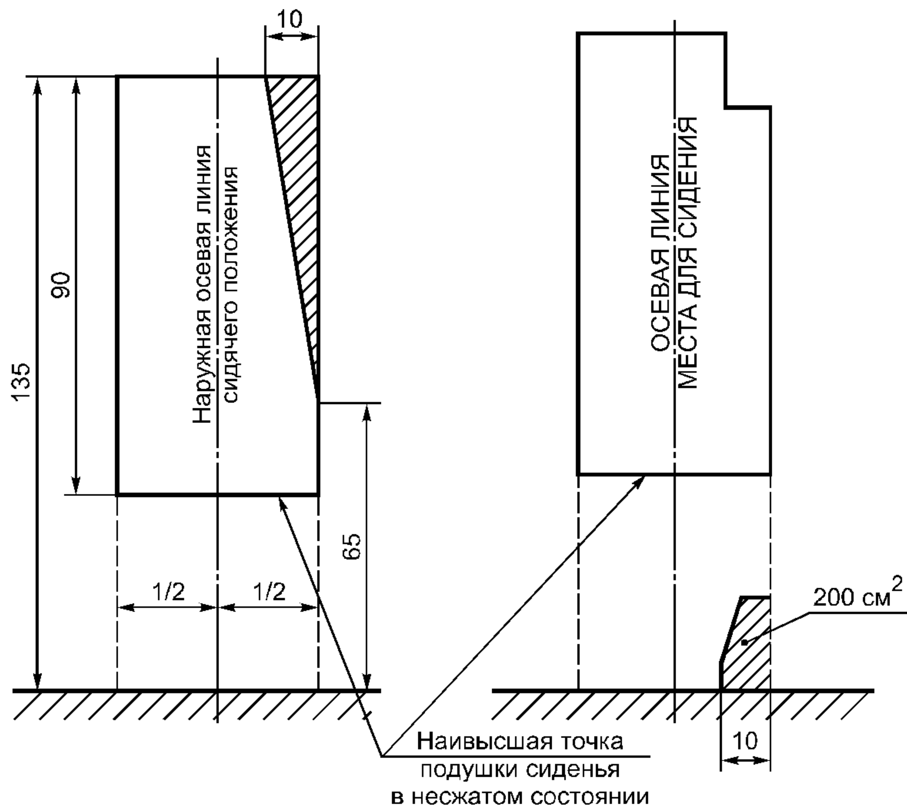
Рисунок 3.10 — Допустимый выступ элемента конструкции (см. 5.7.8.6.2.2)
