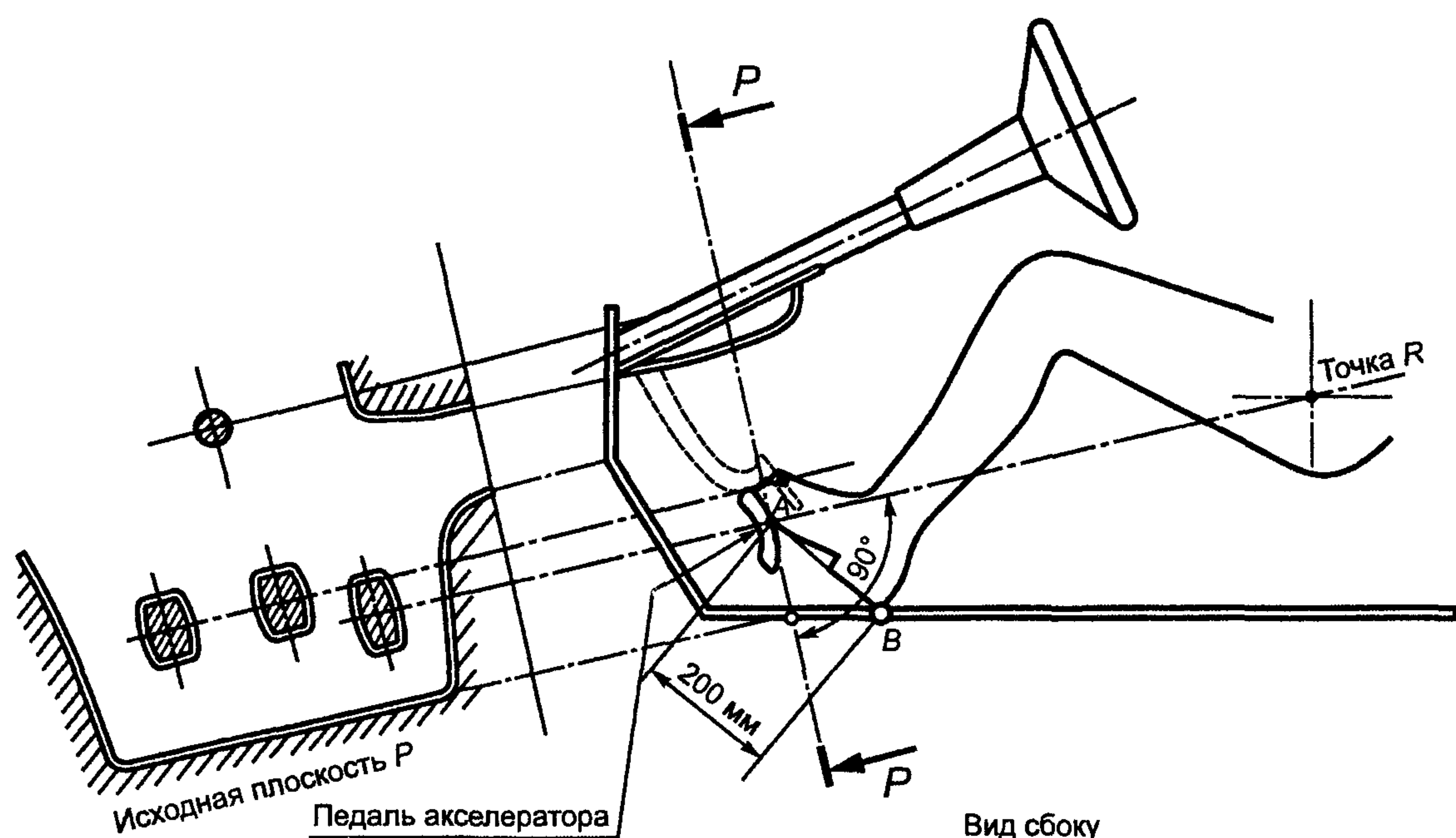
Рисунок 1 — Размещение педалей управления
