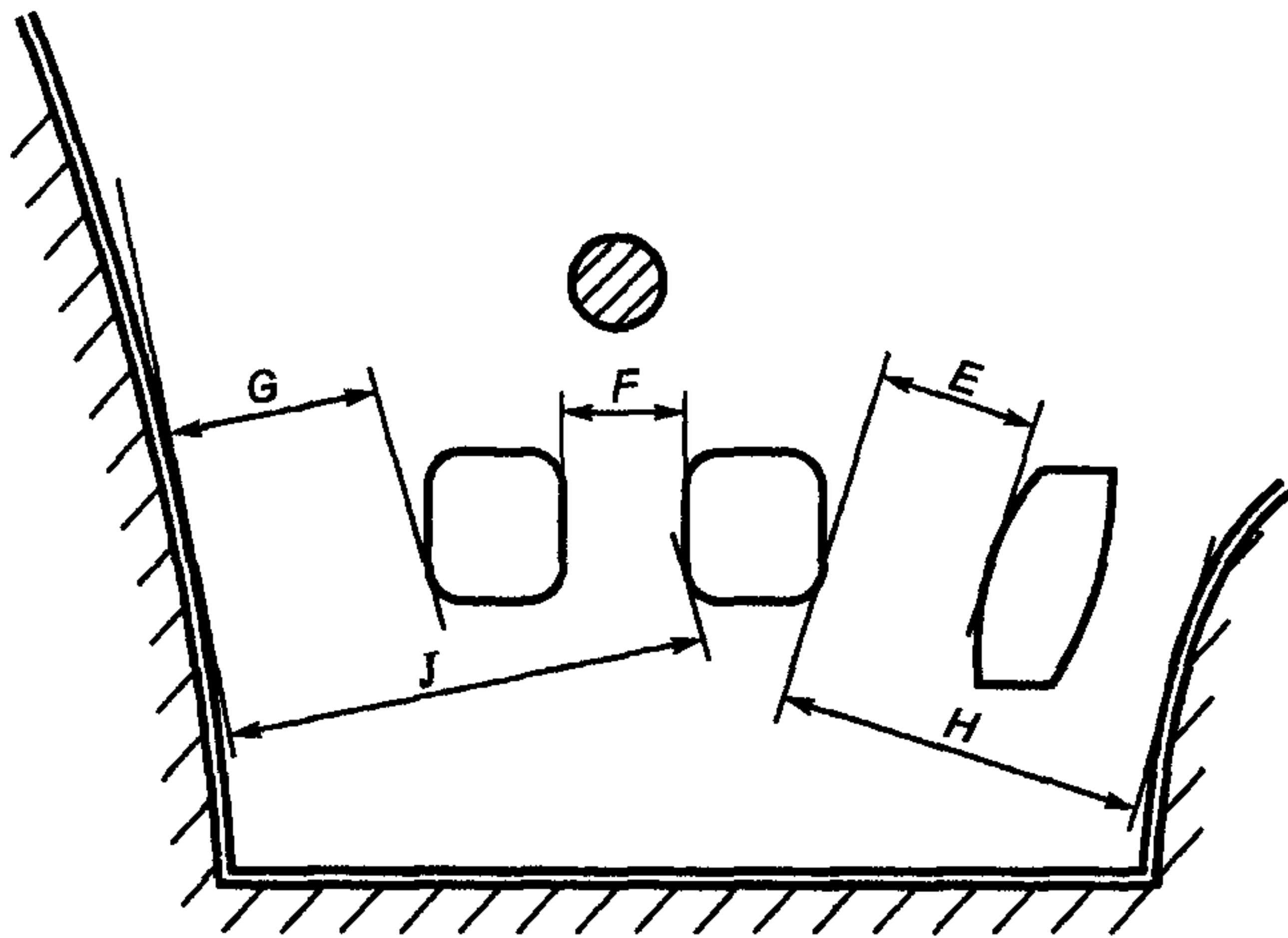
Рисунок 2 — Три педали — трансмиссия обычного типа
