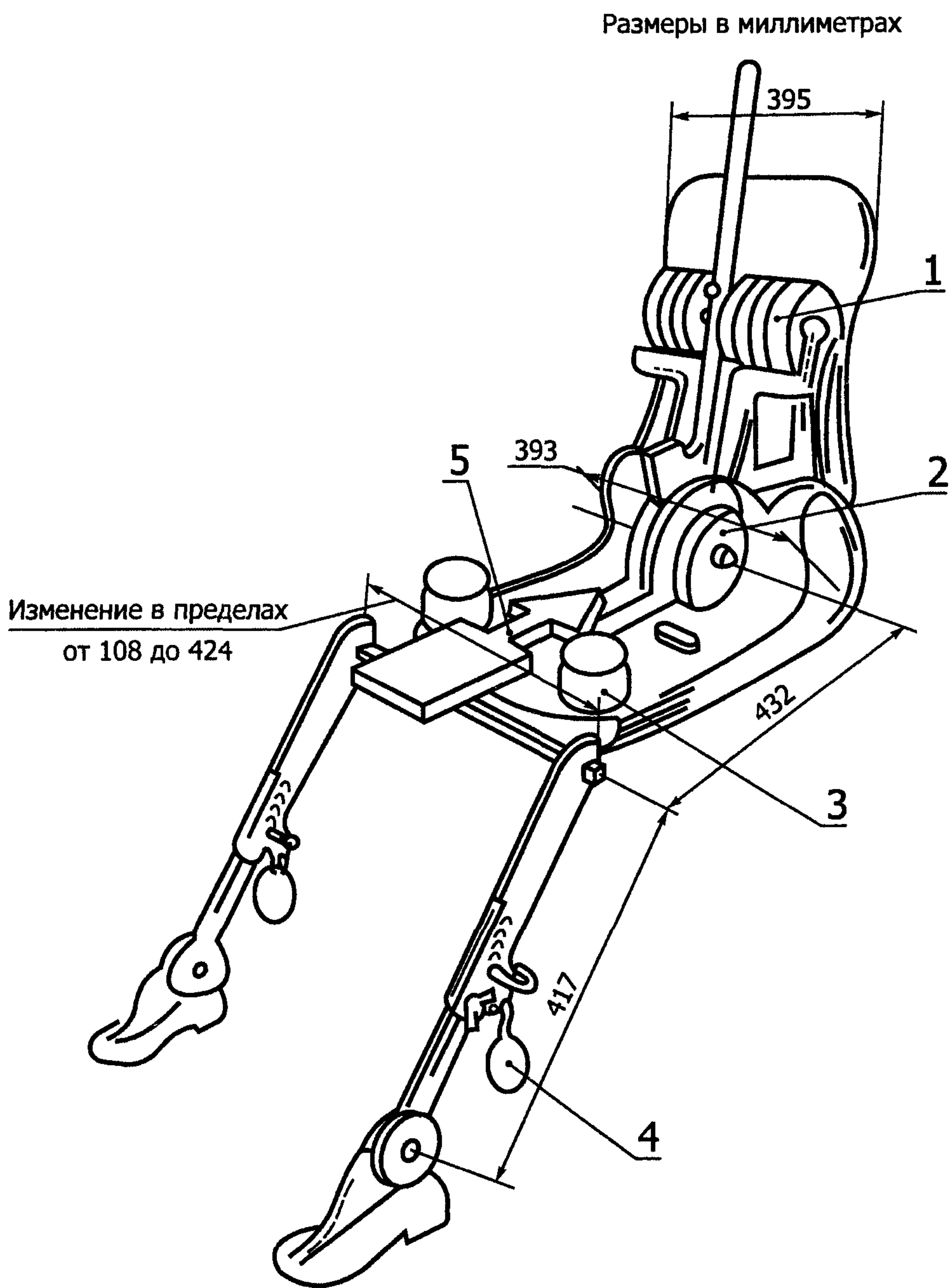
1 — спинные грузы; 2 — седалищные грузы; 3 — набедренные грузы; 4 — ножные грузы; 5 — направление и точка приложения нагрузки
