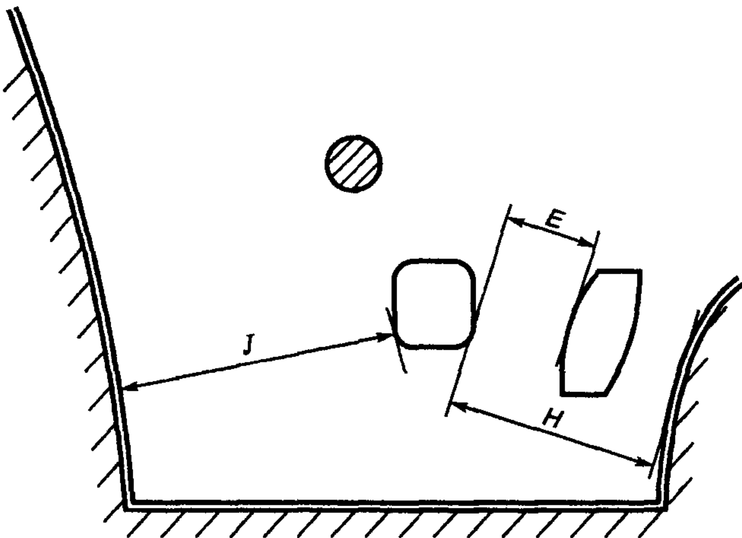
Рисунок 1 — Две педали — автоматическая трансмиссия
