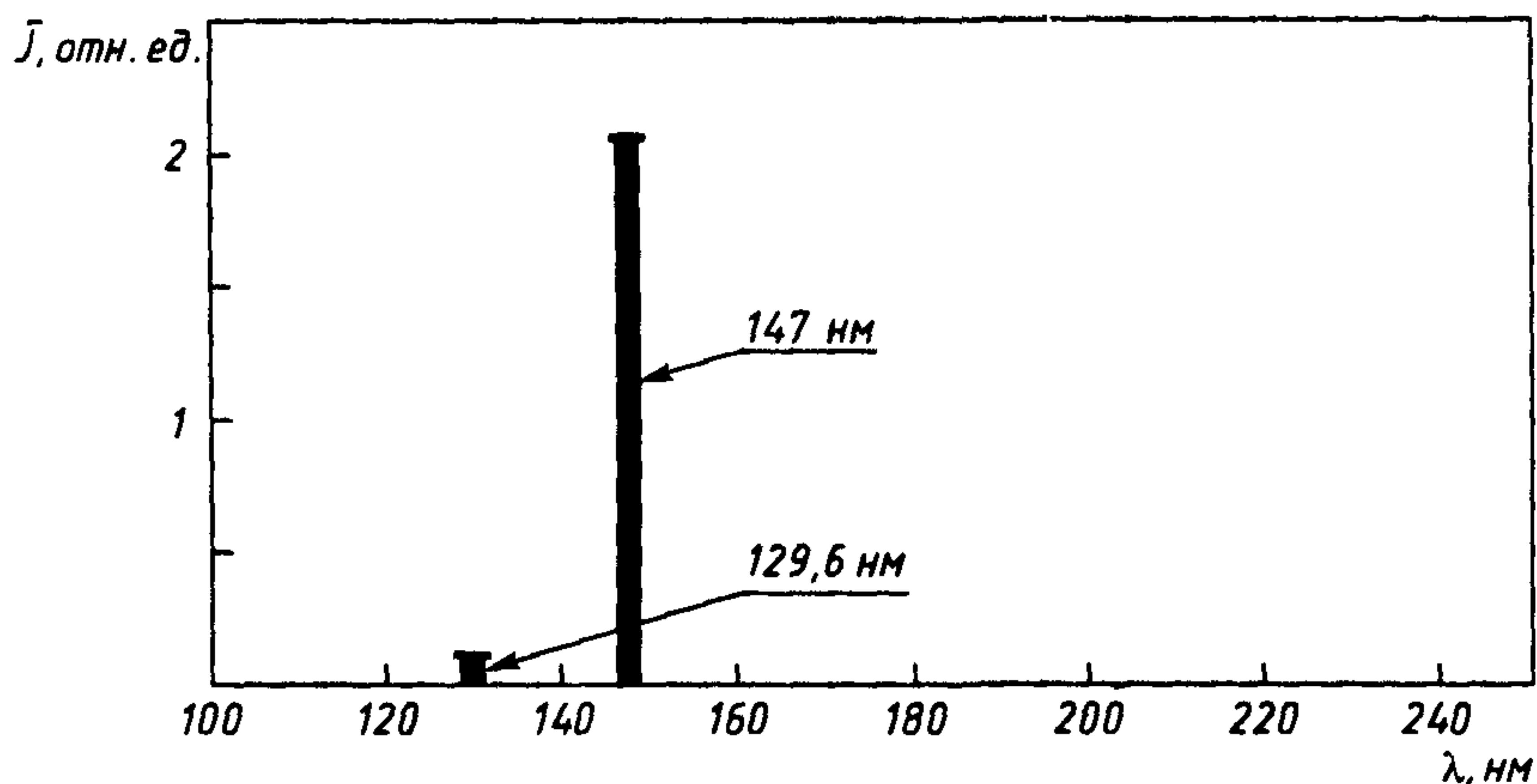
Рисунок 3 — Спектральное распределение излучения ксеноновой лампы
