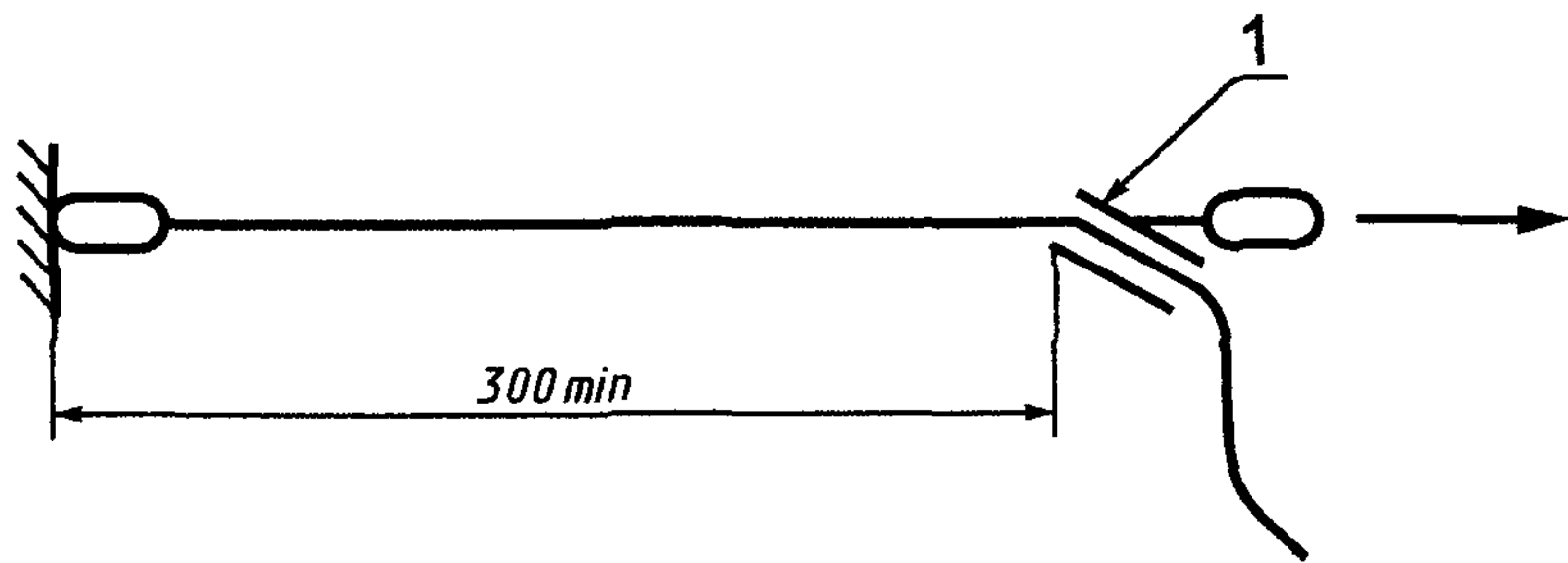
1 — устройство для регулирования длины
