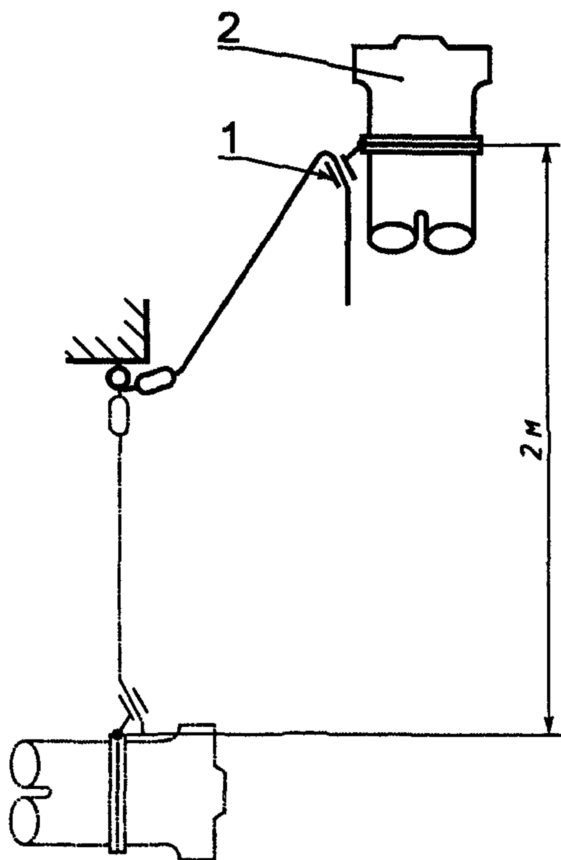
1 — устройство для регулирования длины; 2 — испытательный манекен
