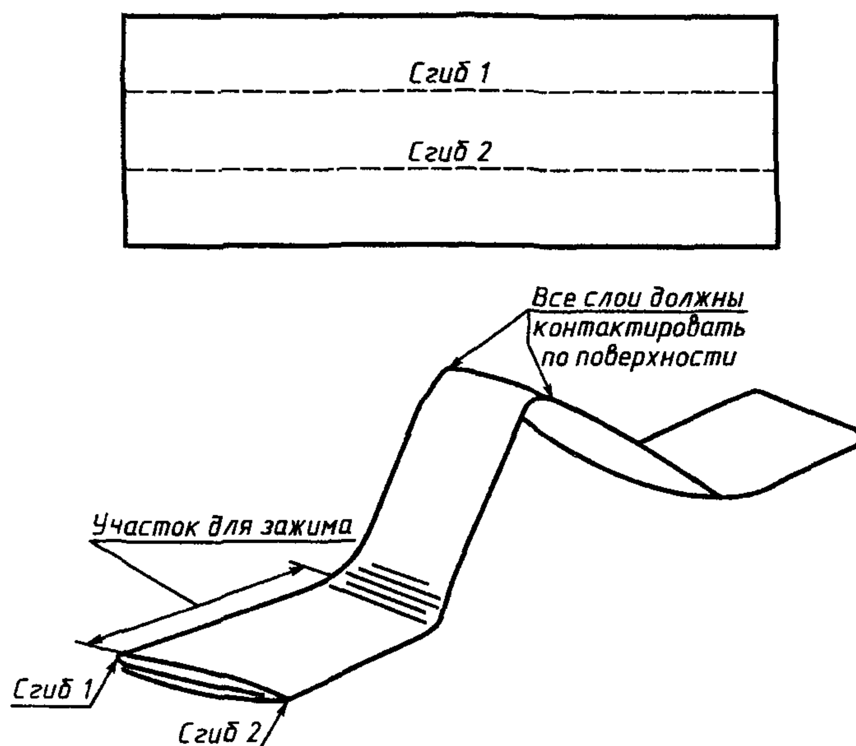
Рисунок 1 — Подготовка элементарной пробы к испытанию методом Де Метта
