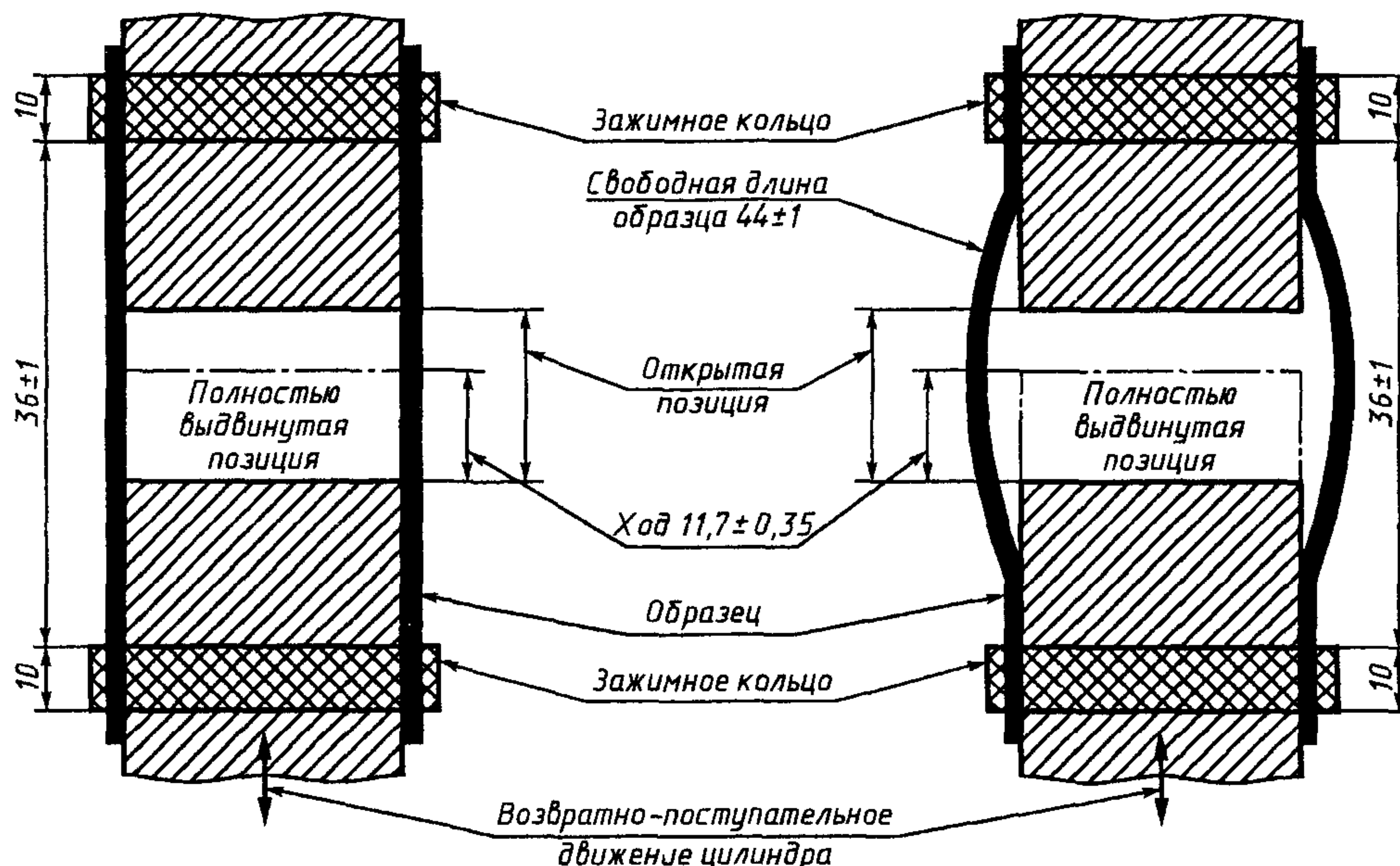
Рисунок 3 — Схема испытания методом определения при изгибе цилиндрического образца (метод Б)
