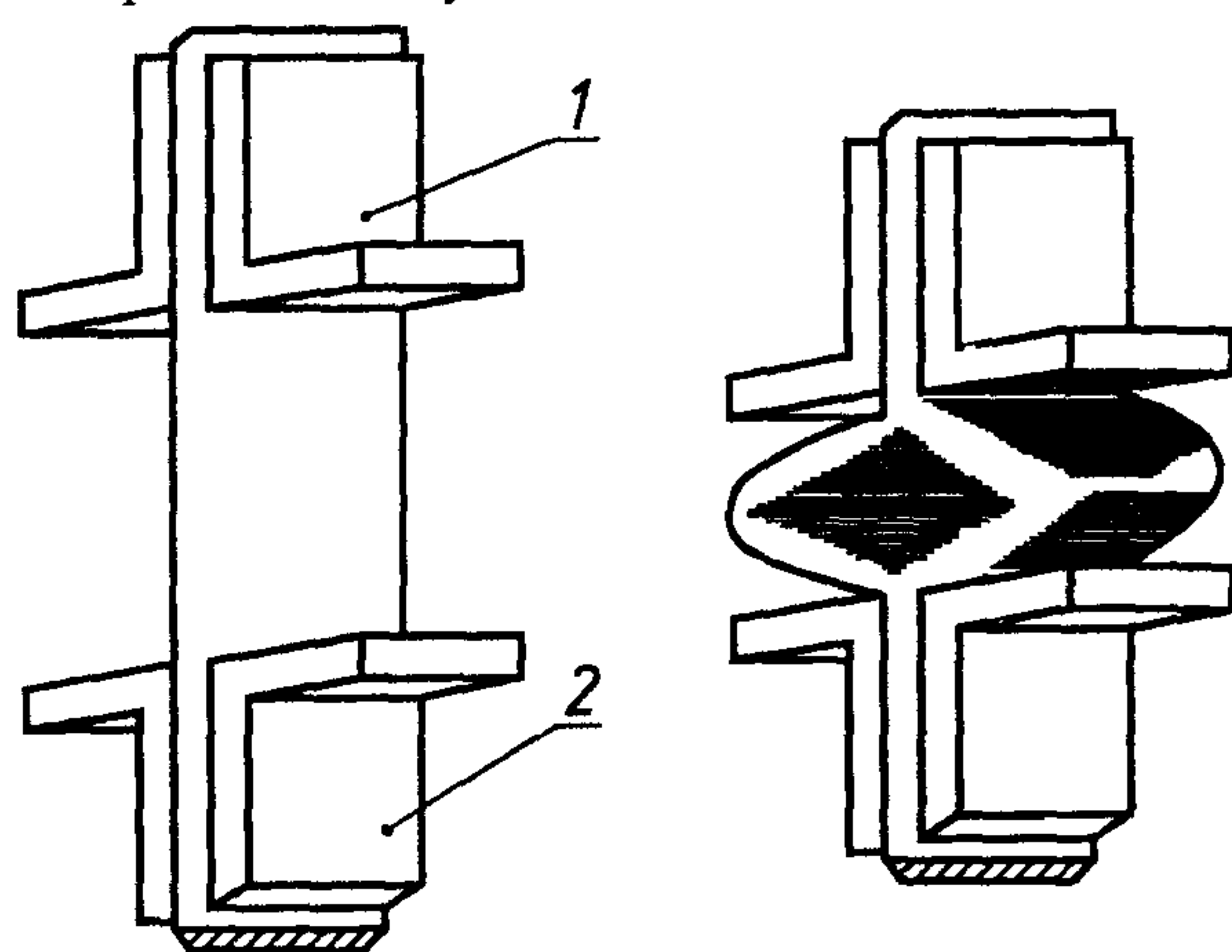
1 — неподвижный зажим; 2 — подвижный зажим
