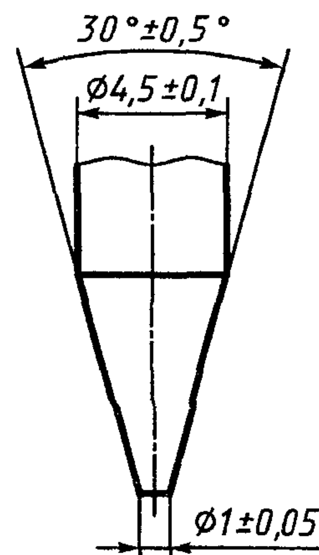
Рисунок 2 — Форма рабочей части прокалывающей иглы
