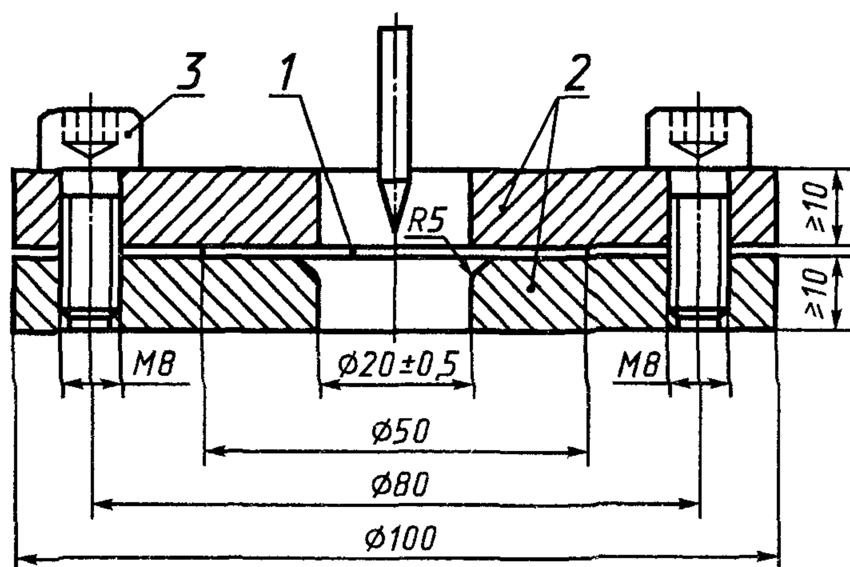
1 — элементарная проба; 2 — пластины; 3 — зажимные болты
