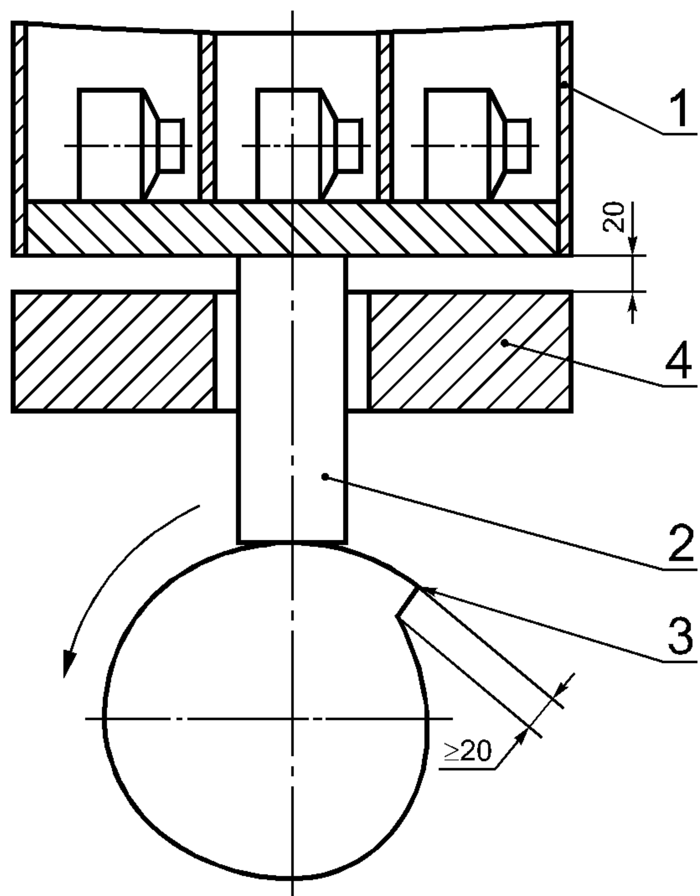
1 — стальная коробка; 2 — поршень; 3 — кулачок; 4 — стальная пластина
