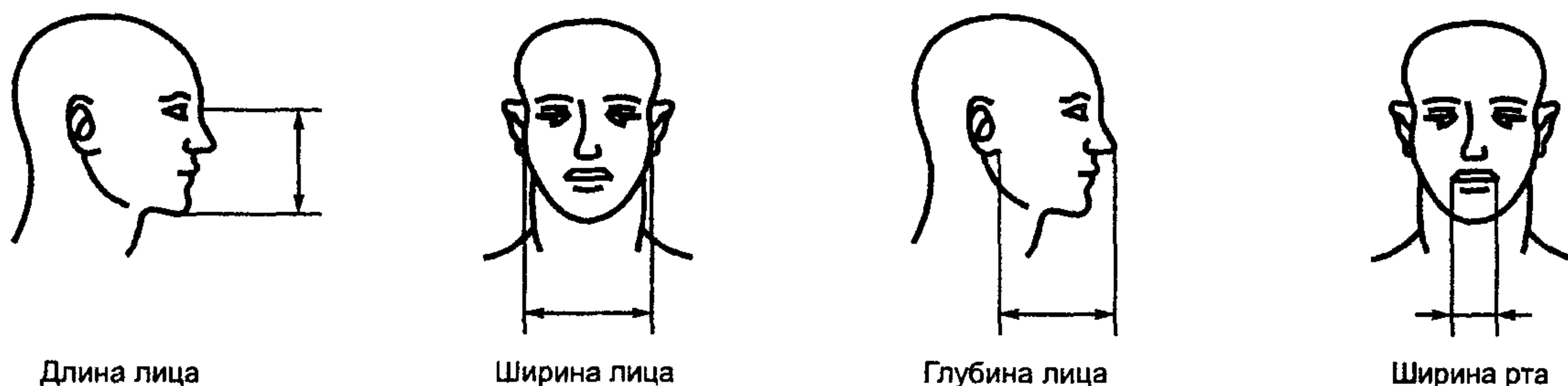
Рисунок 6 — Параметры лица
