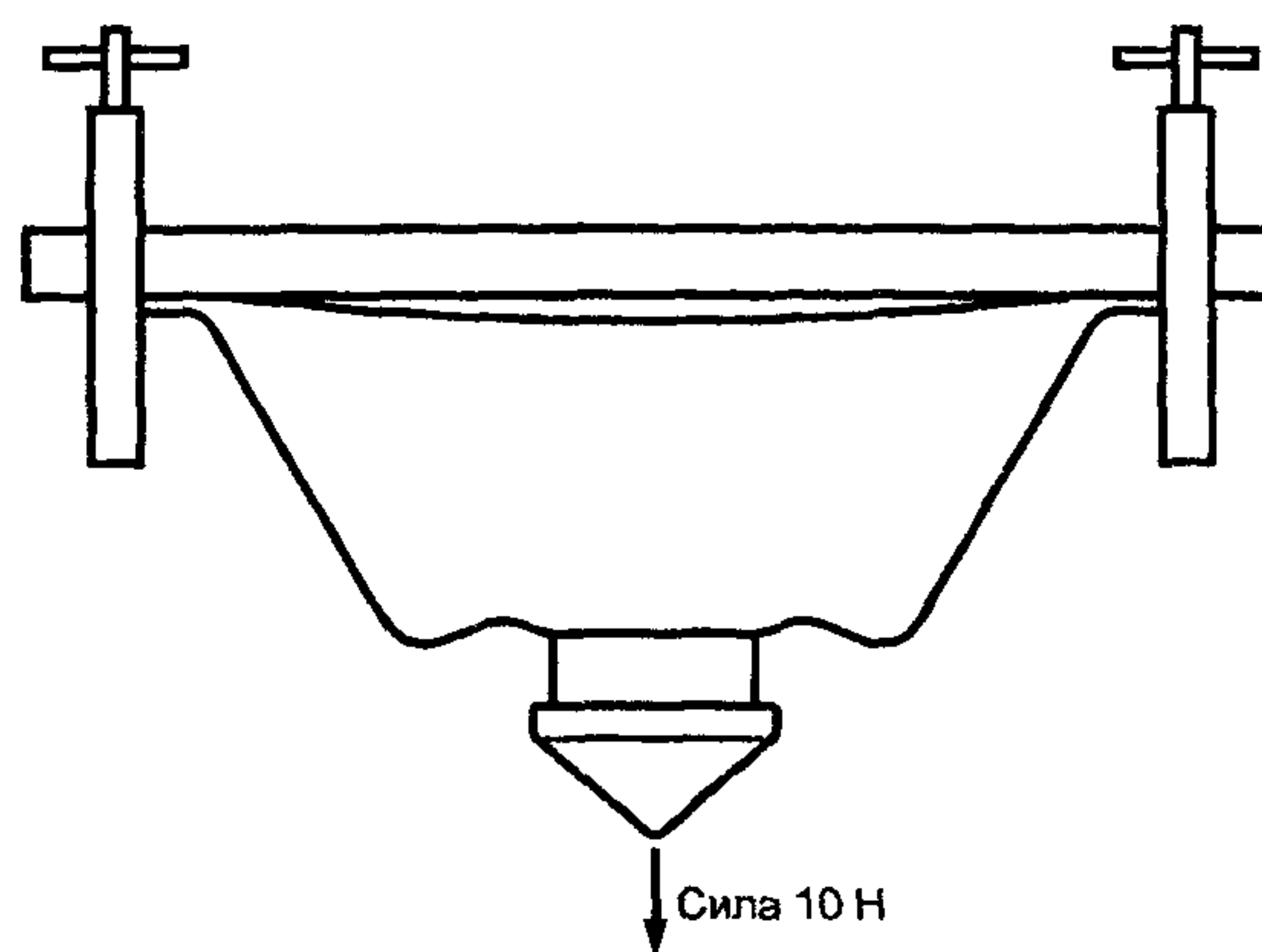
Рисунок 10 — Зажимное устройство для лицевой части
