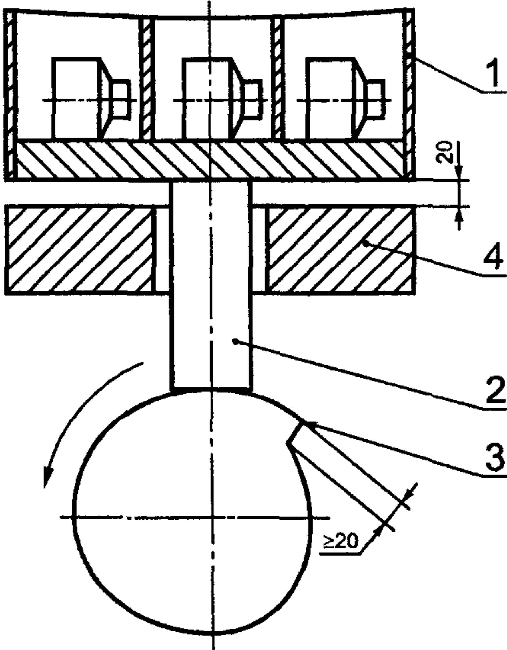
1 — стальная коробка; 2 — поршень; 3 — кулачок; 4 — стальная пластина Рисунок 1 — Установка для механического воздействия
