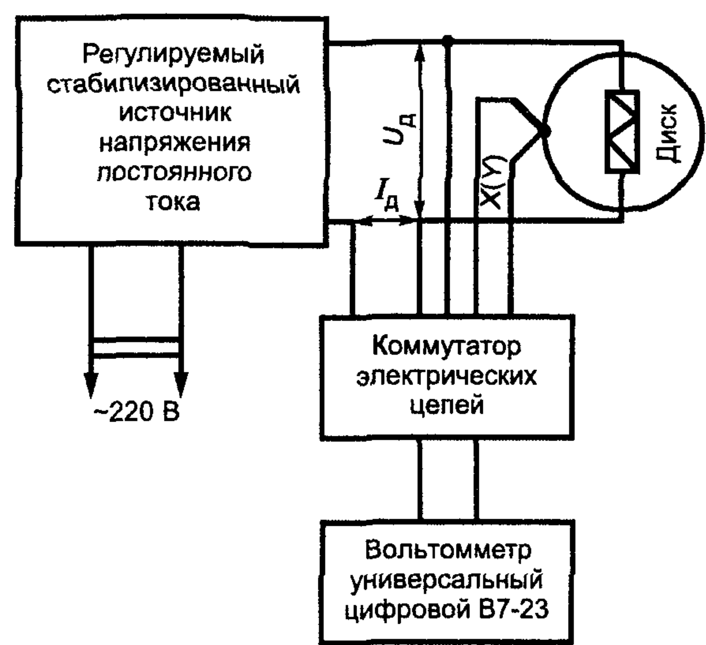
Рисунок Б.2 — Электрическая схема градуировочного стенда
