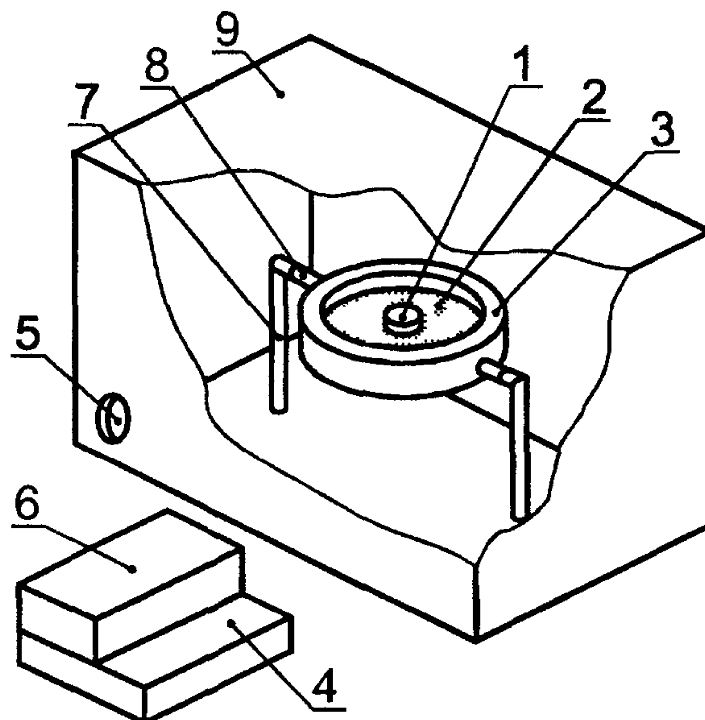
1 — датчик, закрепленный на диске; 2 — диск, 3 — охранный кольцо из пенополиуретана, 4 — средство измерения; 5 — отверстие шлюза для проводов; 6 — регулируемый источник стабилизированного напряжения для питания диска; 7 — неподвижная стойка, 8 — цилиндрический шарнир (для поворота диска); 9 — камера с относительно неподвижным воздухом объемом \approx 2 м 3
