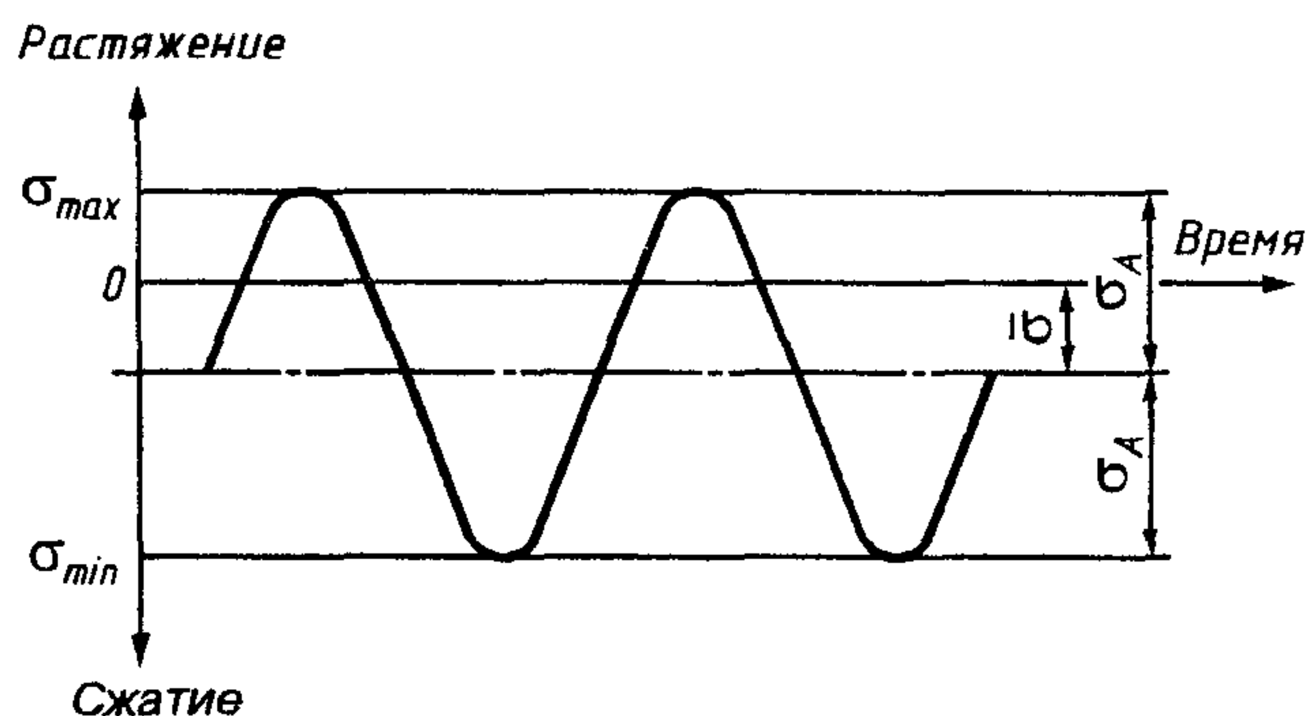
Рисунок А.2 — Синусоидальная кривая напряжений
