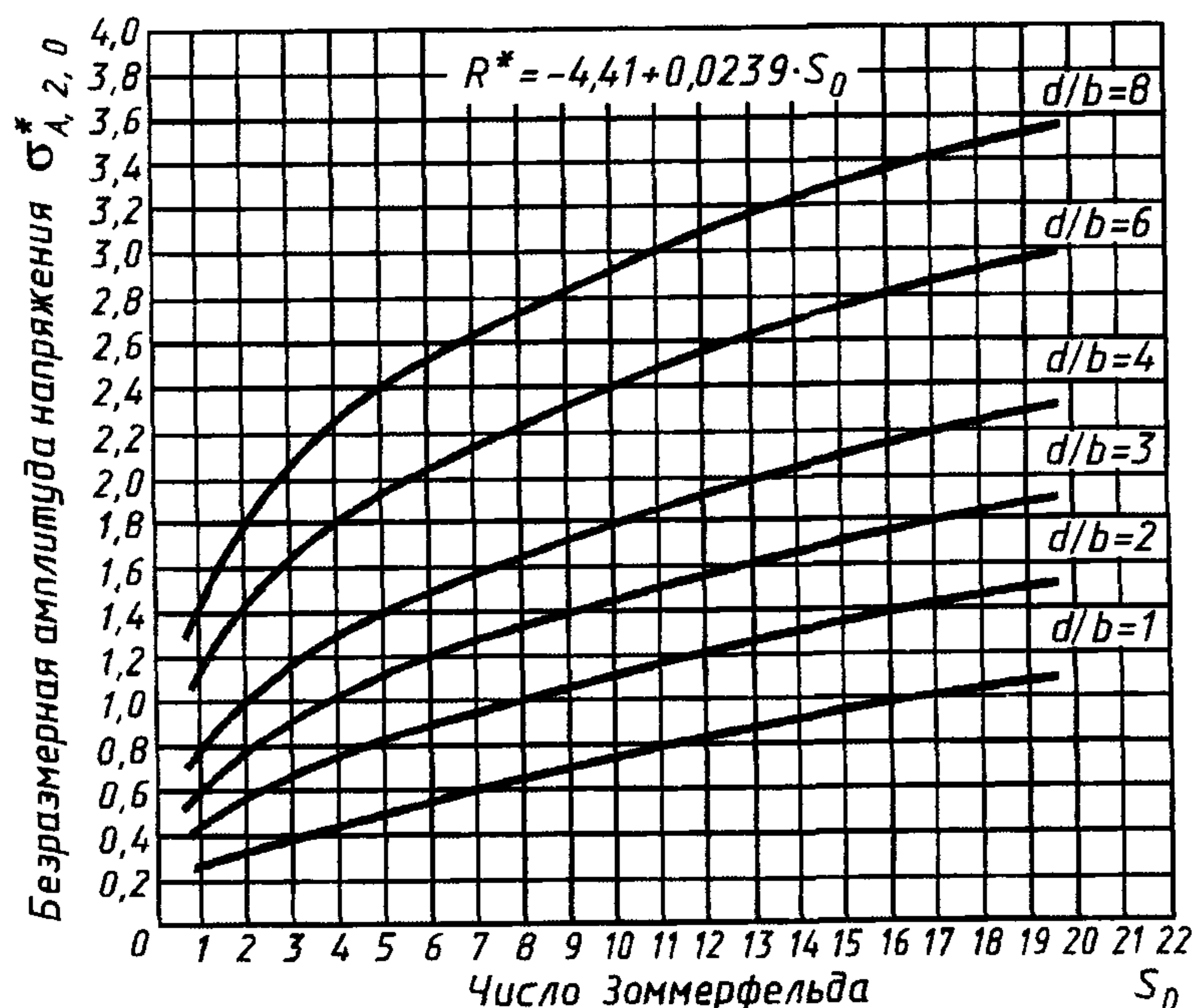
Рисунок А.3 — Антифрикционный слой/промежуточный слой:
