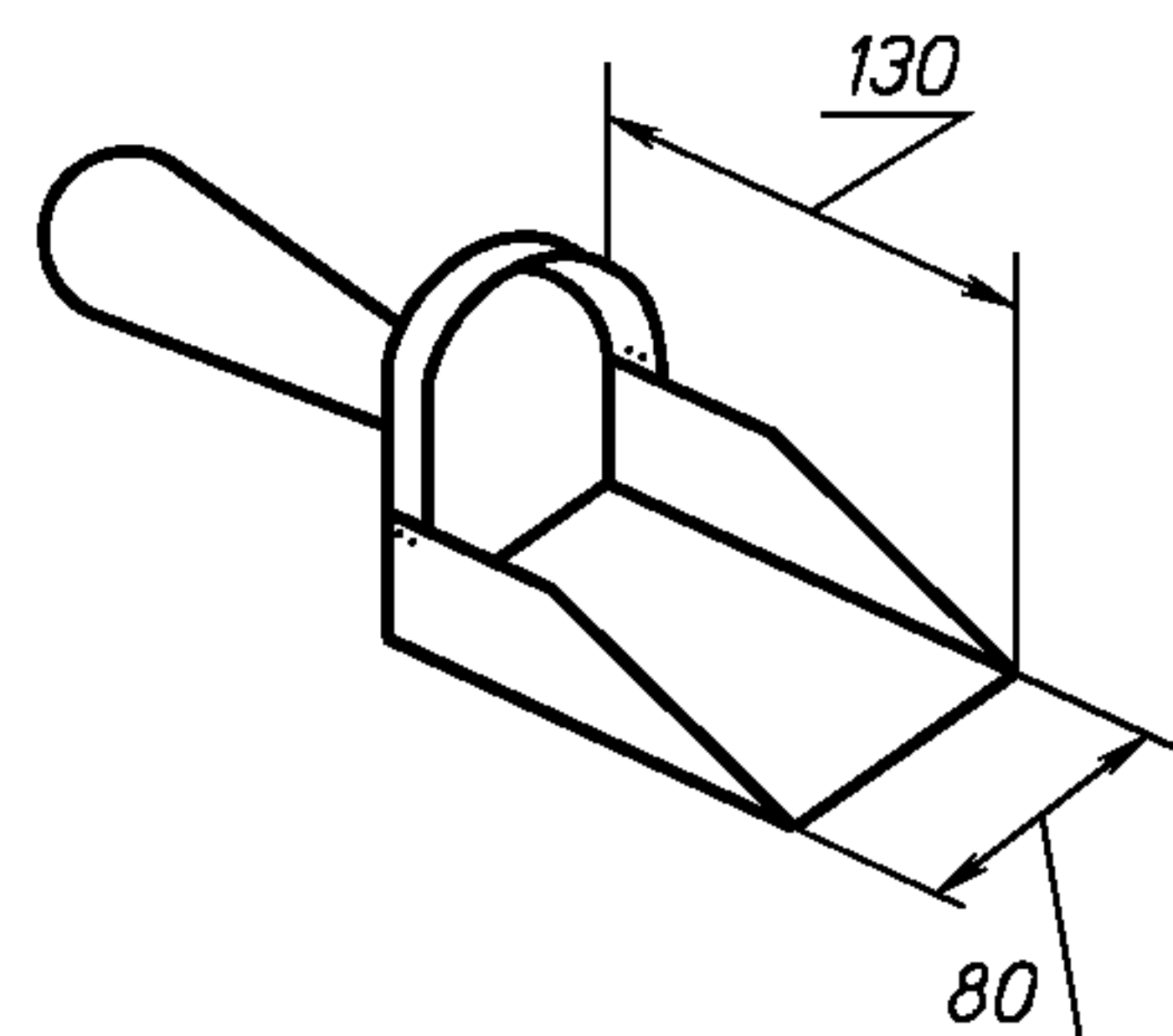
Рисунок 2 — Совок
