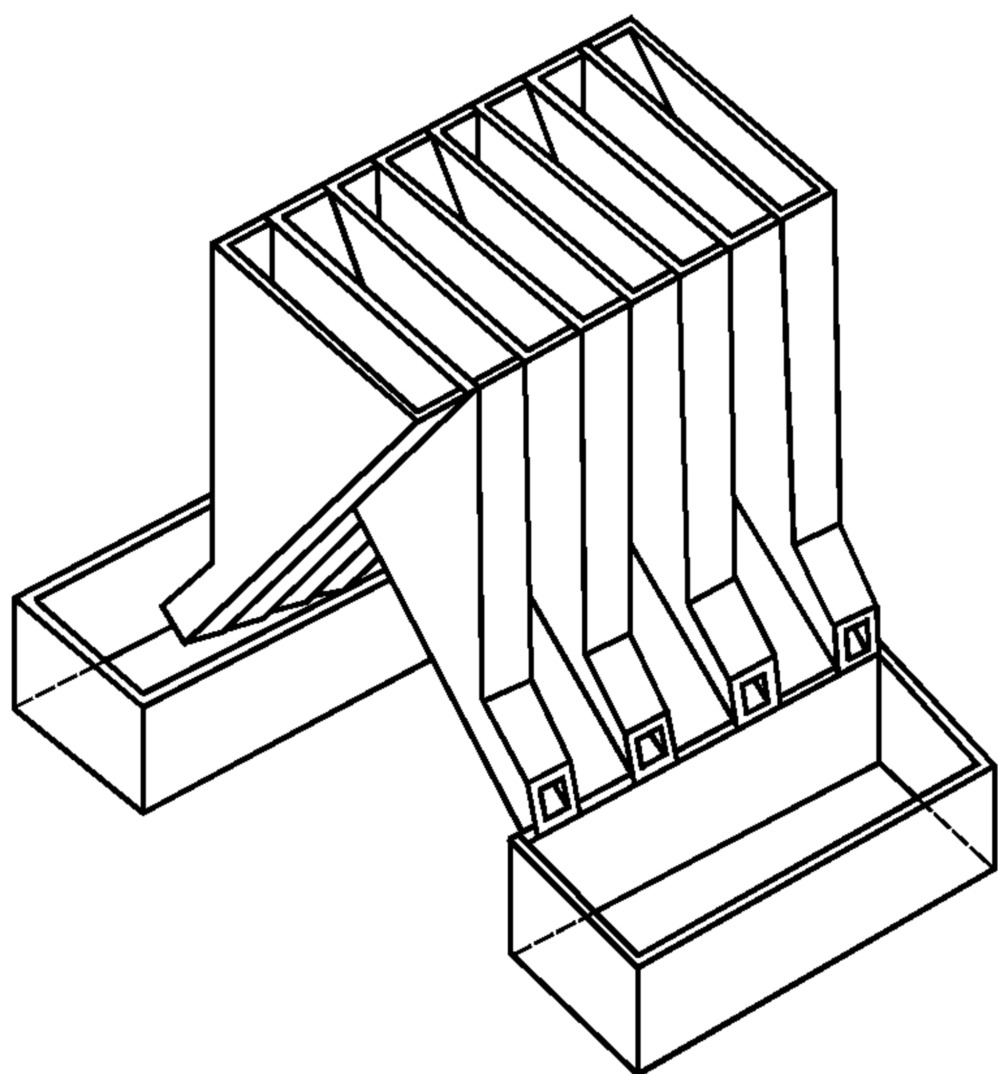
Рисунок 8 — Конический делитель
