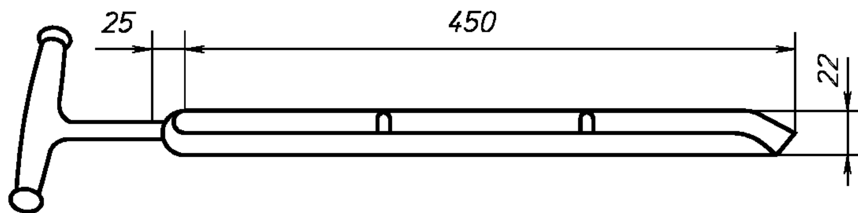
Рисунок 3 — Секционный щуп открытого типа
