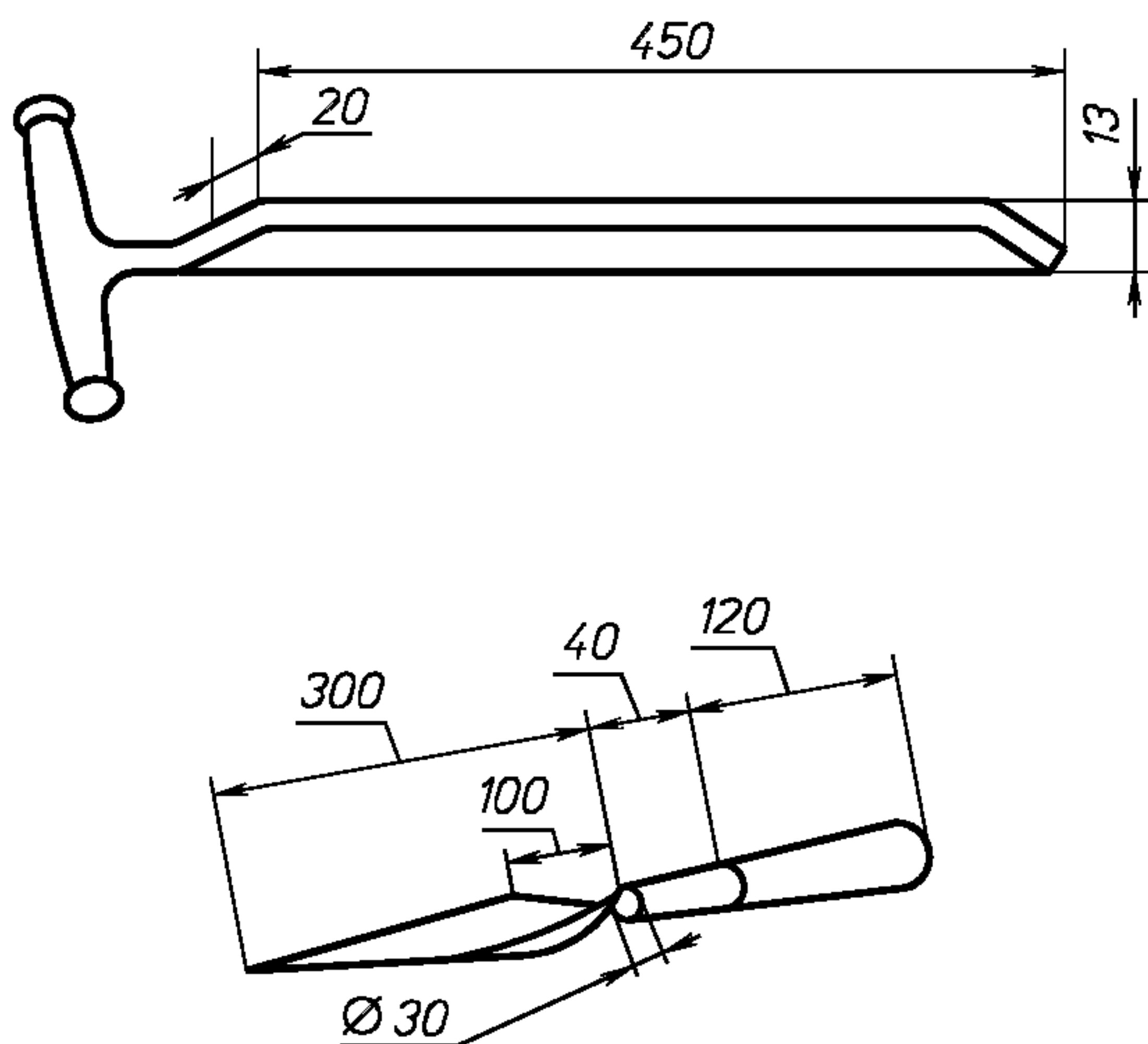
Рисунок 1 — Щуп открытого типа
