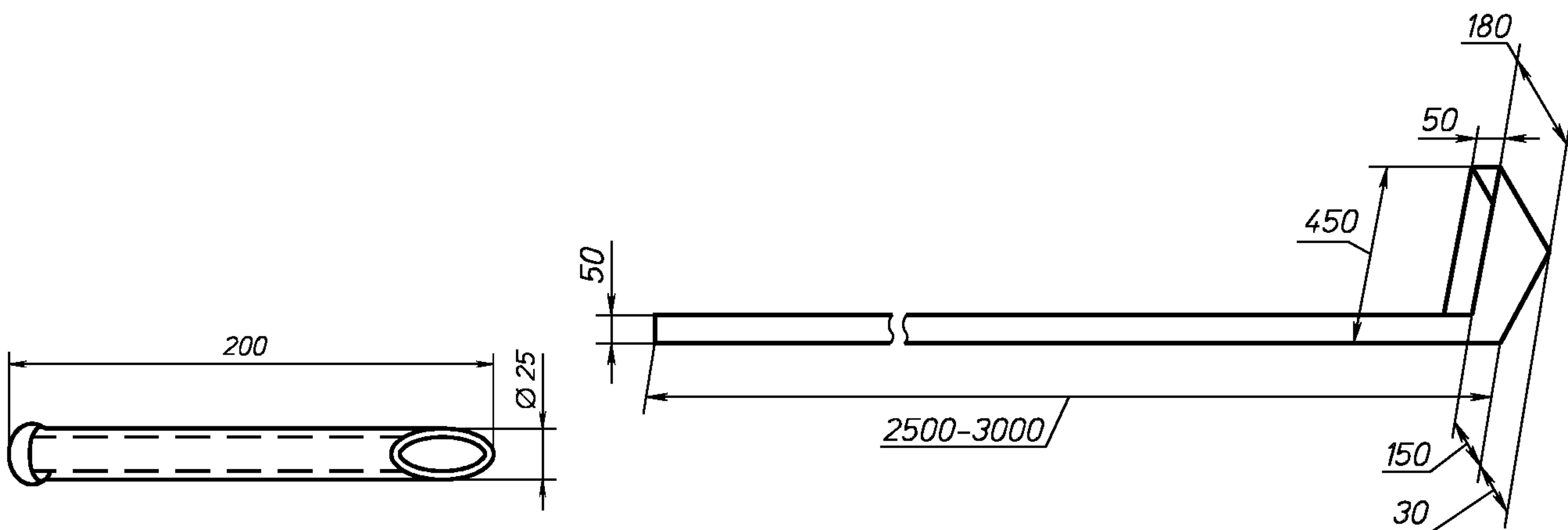
Рисунок 5 — Пробоотборник для отбора проб из мешков (мешочный щуп)
