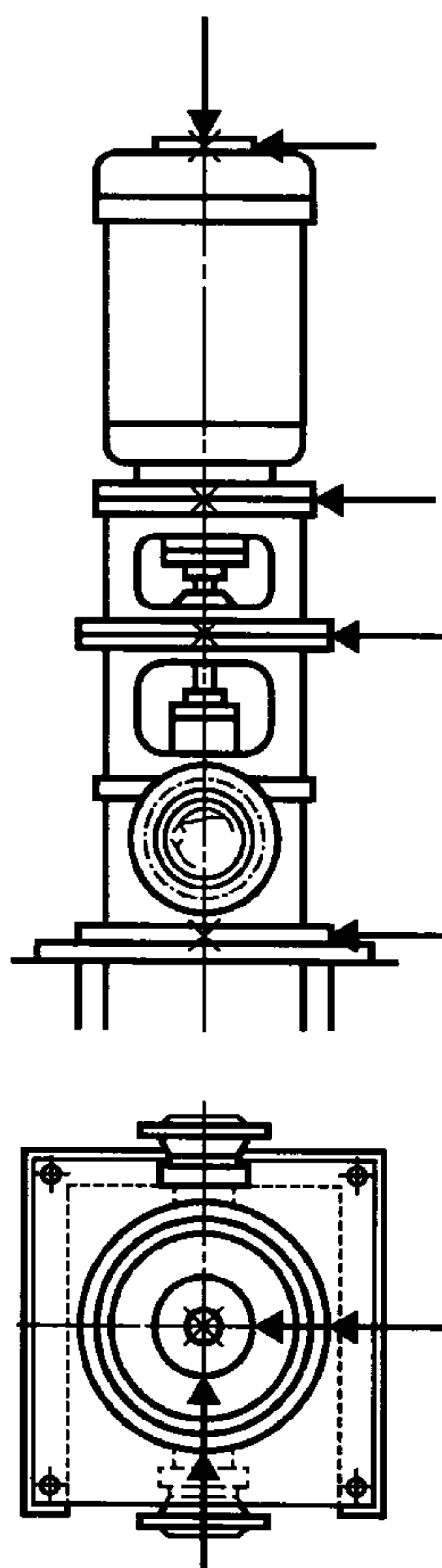
Рисунок 1д — Точки измерения на вертикально установленной машине
