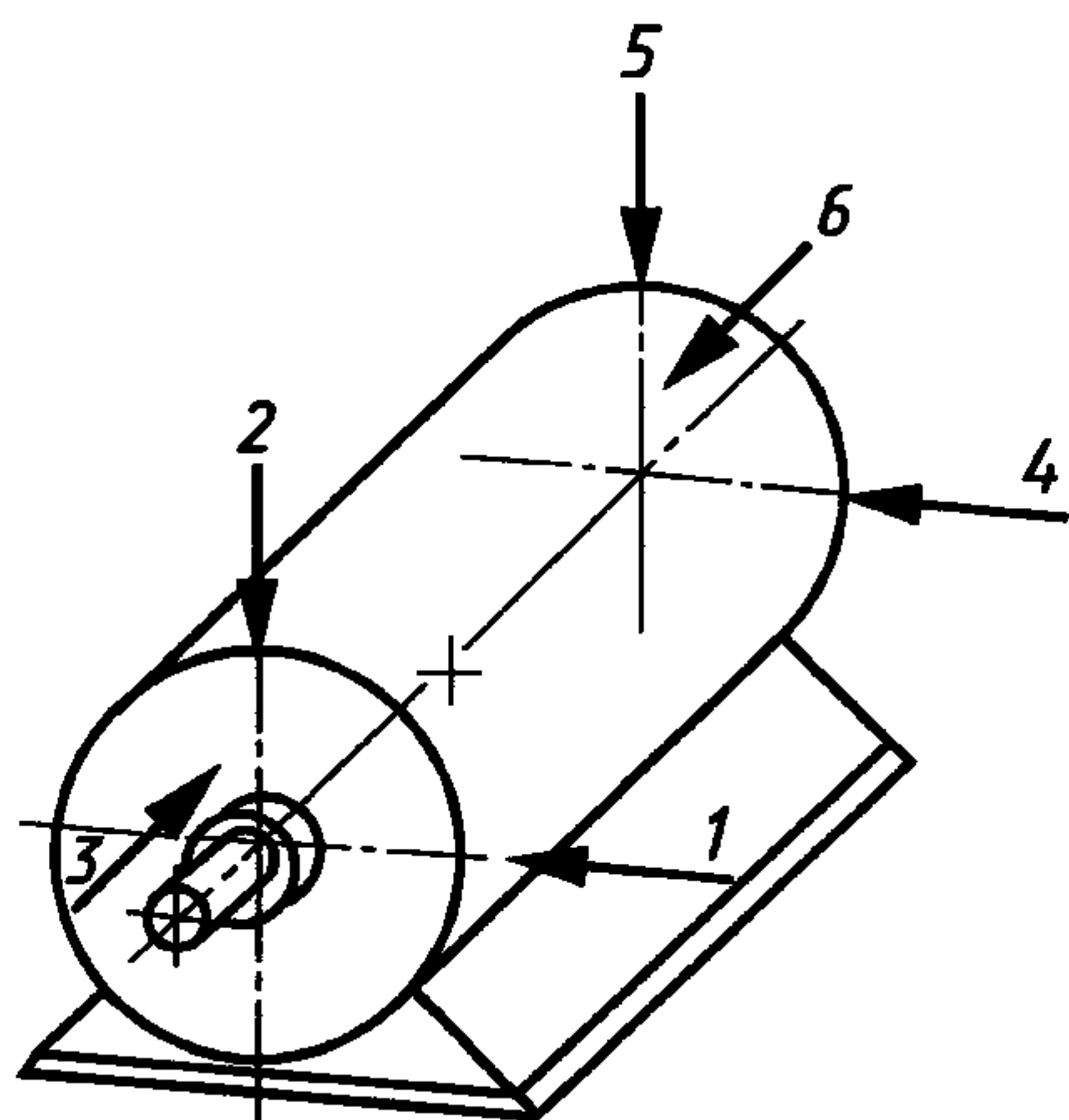
Рисунок 1в — Точки измерения на малых электрических машинах
