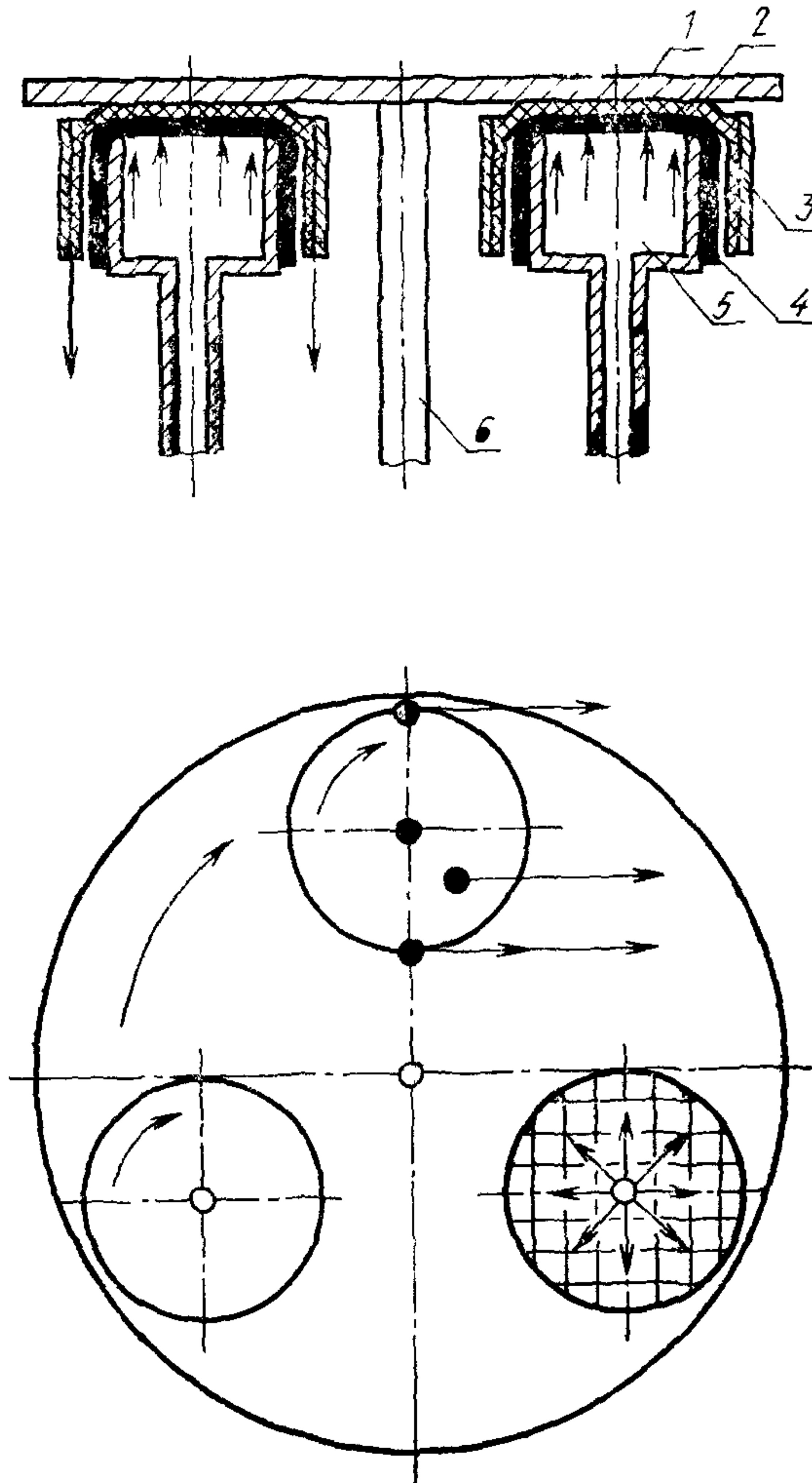
1 — истирающий диск; 2 — проба; 3 — обойма; 4 — мембрана; 5 — головка; 6 — ось
