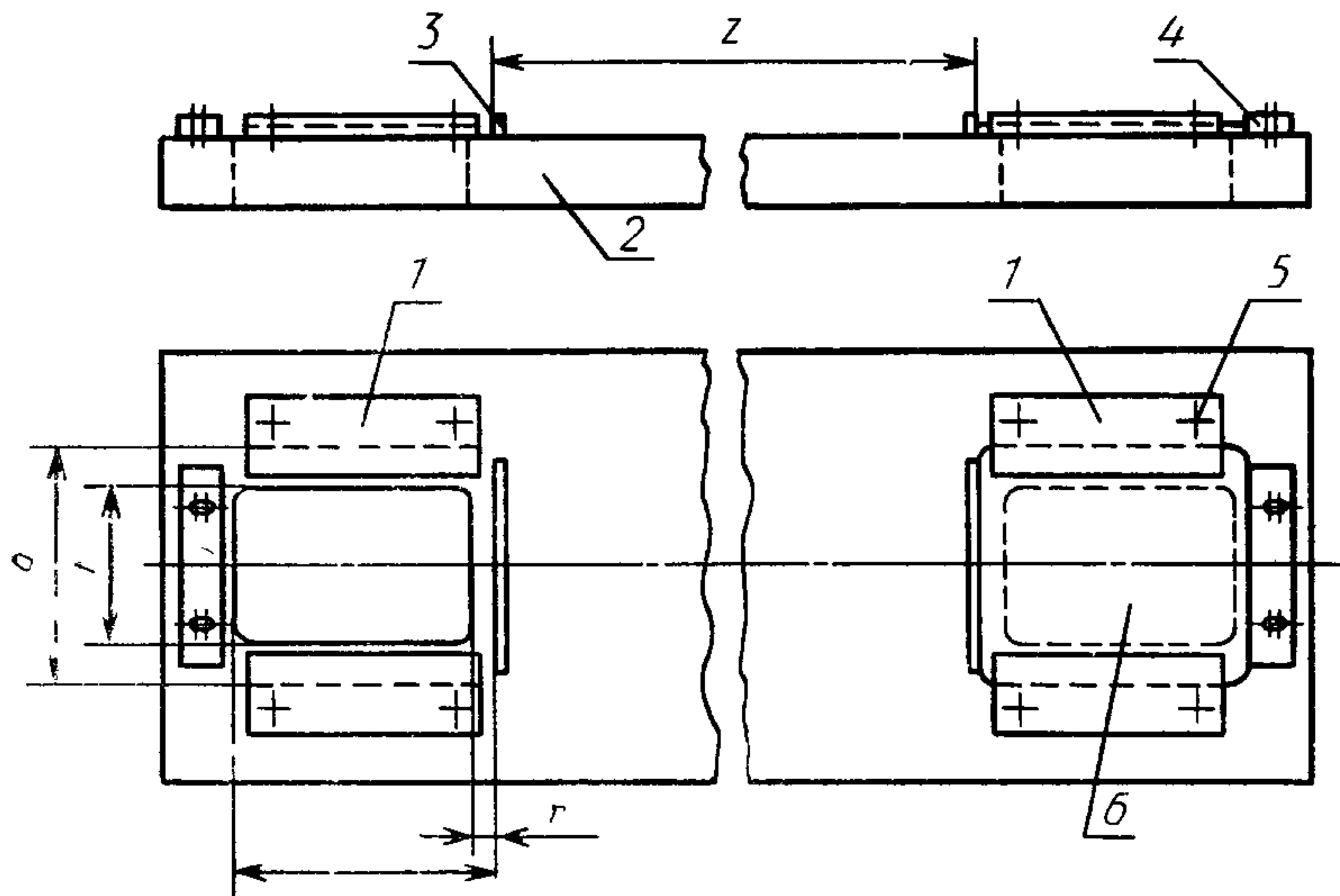
1 — зажимная скоба * (перекрытие монтажной пластины — 10 мм); 2 — опора; 3 — упор; 4 — планка для прижима монтажной пластины к упору; 5 — винты креп- ления зажимной скобы; 6 — монтажная пластина (см. черт. 2)
