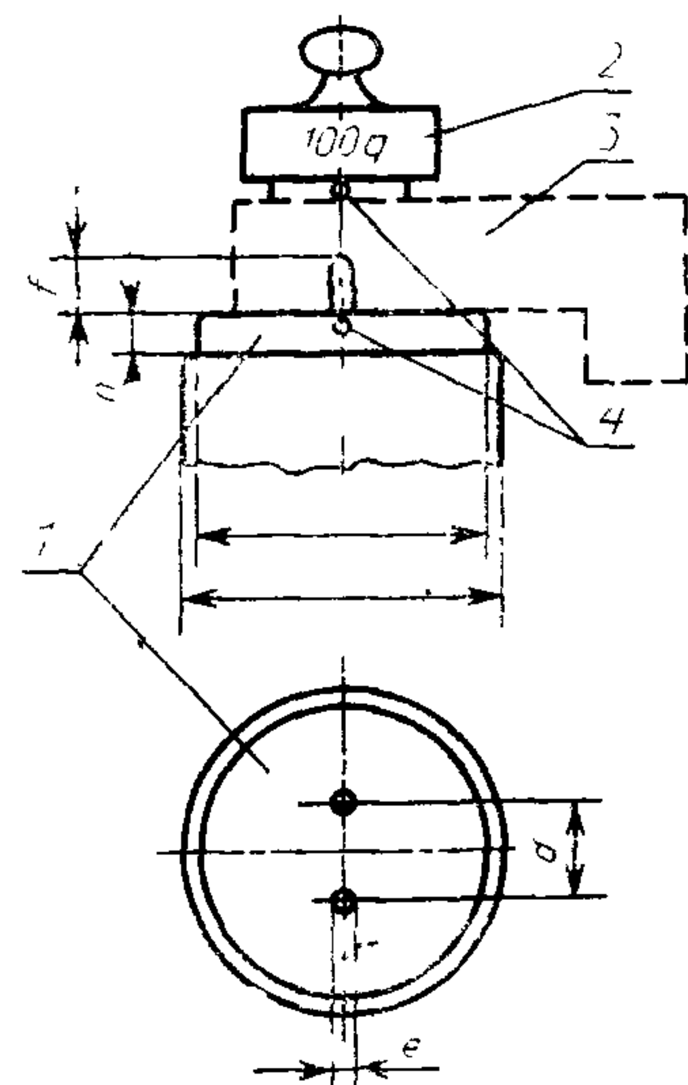
1 — испытательный цоколь; 2 — груз; 3 — патрон для ламп; 4 — термоэлектрические преобразователи
