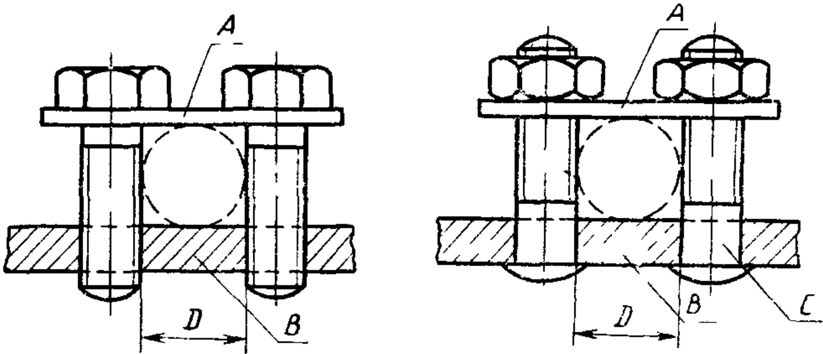
A — прижимная пластина, B — опорная деталь, C — шпилька; D — место расположения жилы провода
