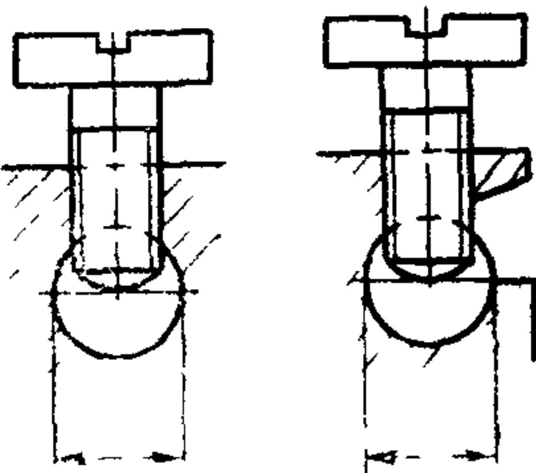
D — место расположения жилы провода
