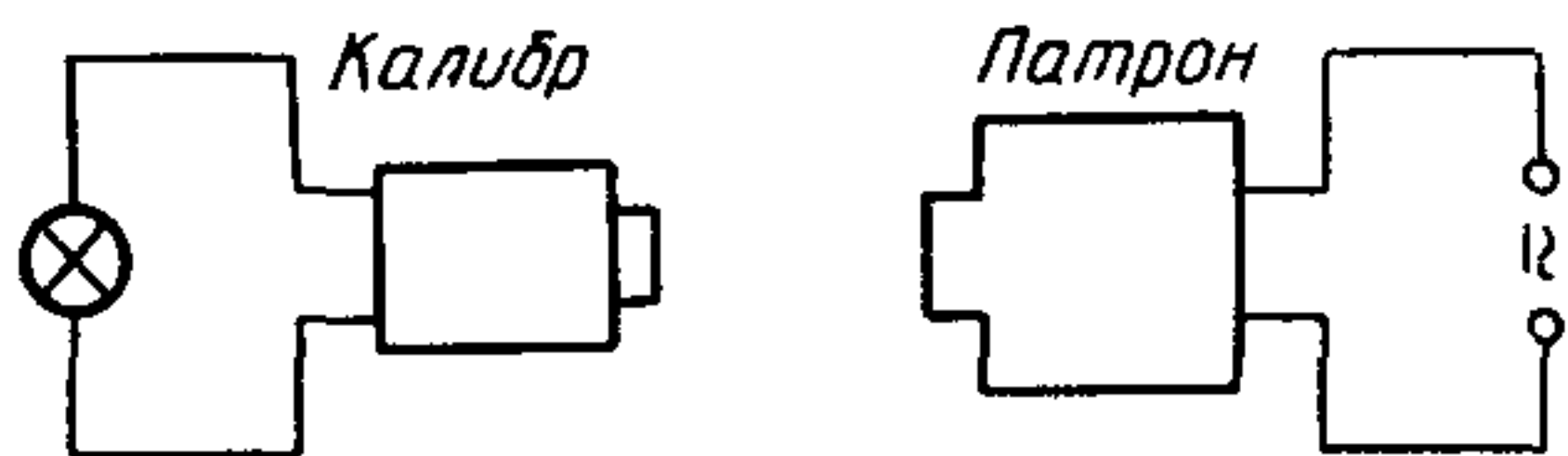
Принципиальная электрическая схема испытания
