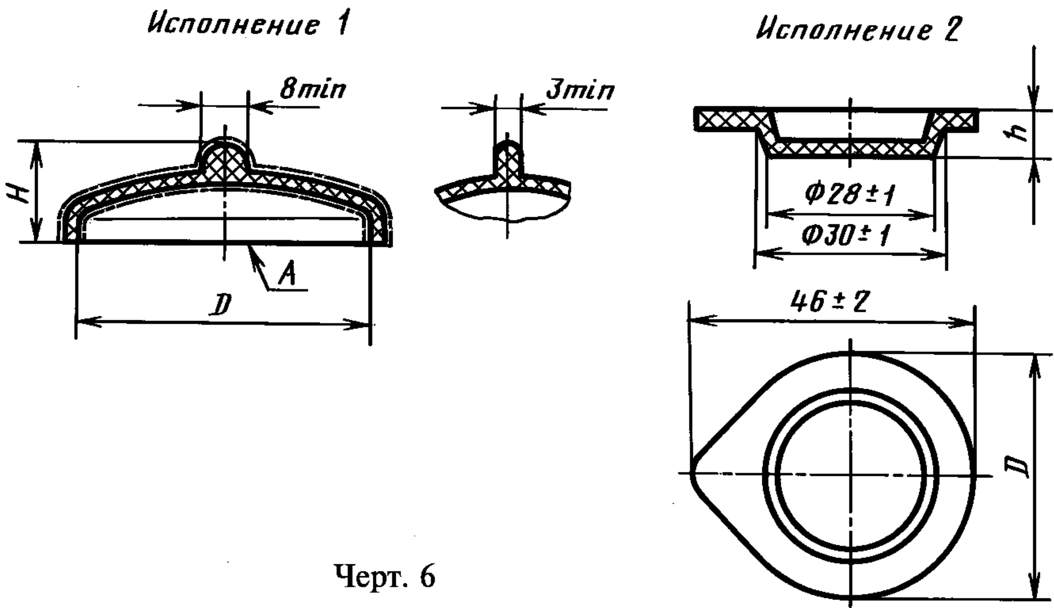
Крышки к тиглям
