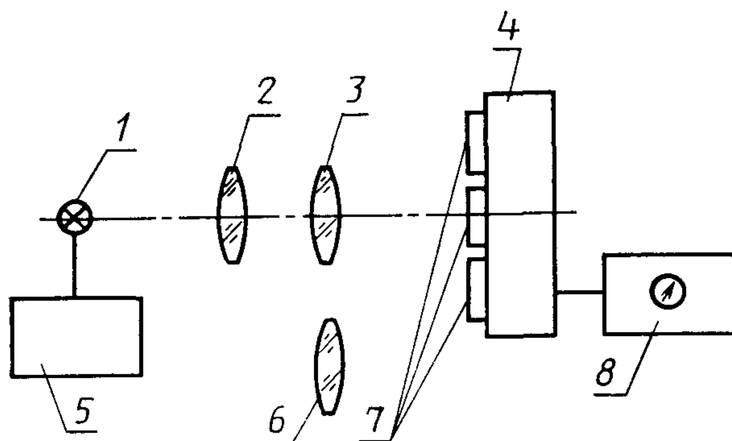
1 — источник света; 2 — коллиматор; 3 — эталонная насадка; 4 — фотоэлектрический колориметр; 5 — стабилизатор напряжения; 6 — испытуемая насадка; 7 — сменные светофильтры; 8 — измерительный прибор
