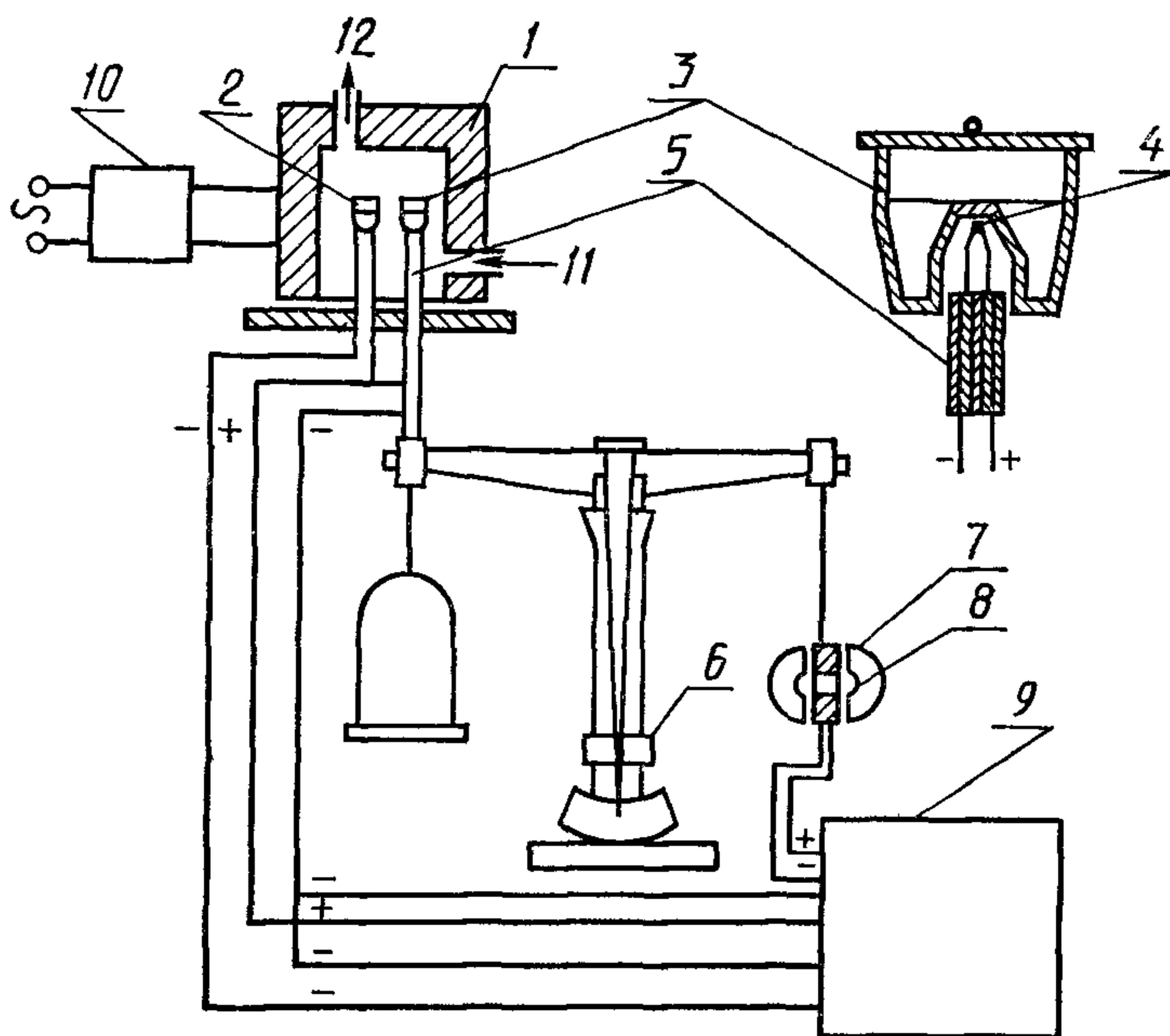
1 — термокамера; 2 — тигель с инертным веществом; 3 — тигель с пробой; 4 — термопара; 5 — керамическая трубка; 6 — весы; 7 — катушка; 8 — магнит; 9 — регистрирующий блок с пишущим устройством; 10 — блок питания и управления нагревом печи; 11 — ввод газа (или вакуумирования); 12 — отвод газообразных продуктов
