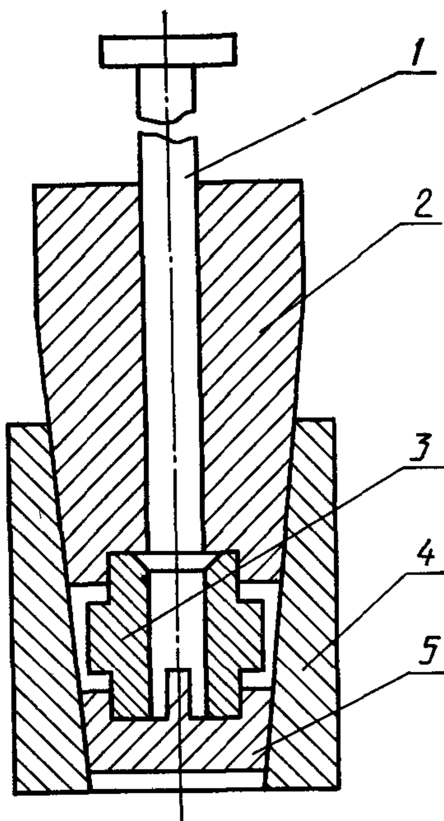
1 — пуансон; 2 — бункер; 3 — гнездо для тигля; 4 — обруч; 5 — пята
