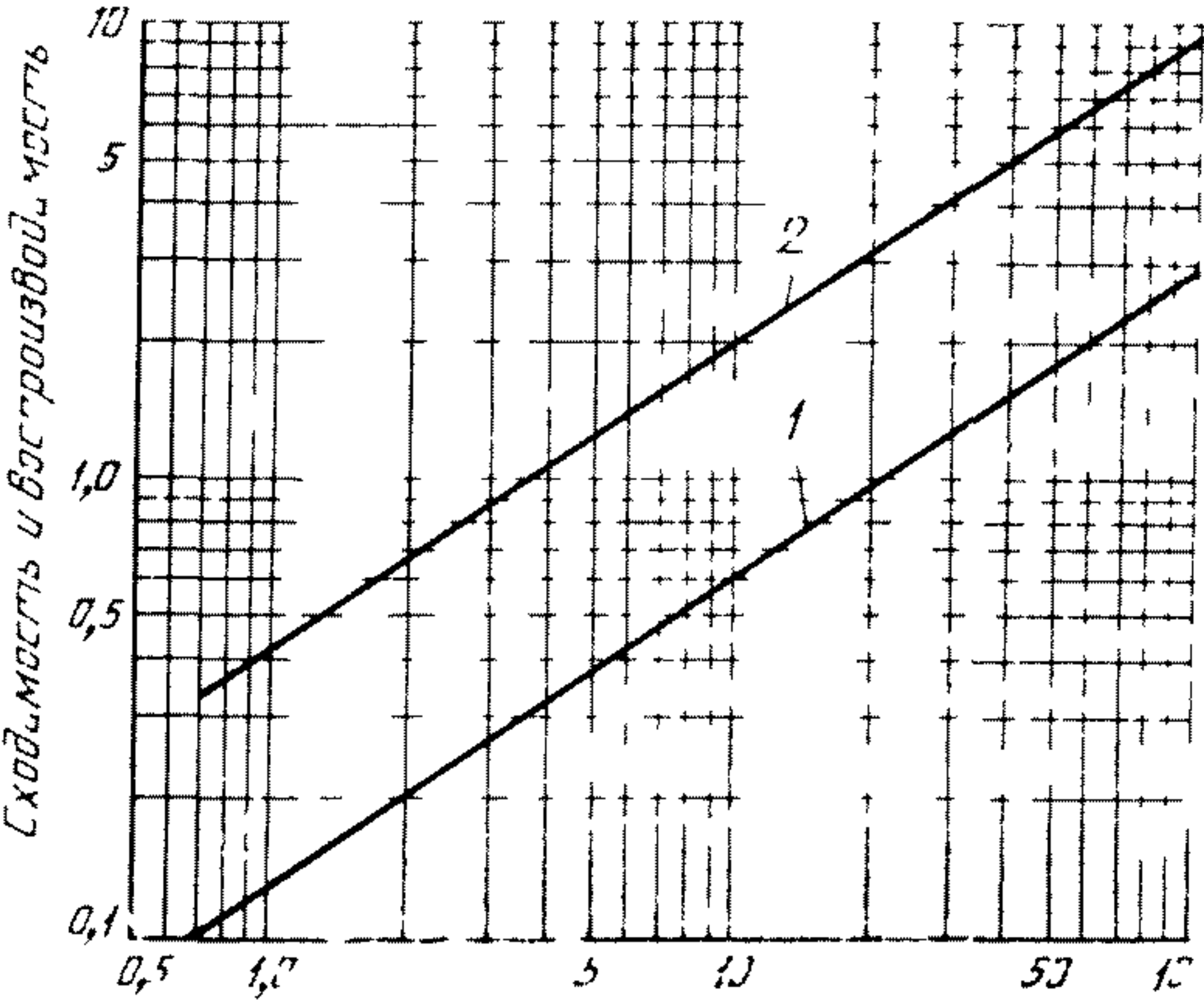
ТОЧНОСТНЫЕ ХАРАКТЕРИСТИКИ РЕЗУЛЬТАТОВ ОПРЕДЕЛЕНИЙ ДЛЯ НЕФТЕПРОДУКТОВ, 90% КОТОРЫХ ВЫКИПАЕТ ДО 205°С
