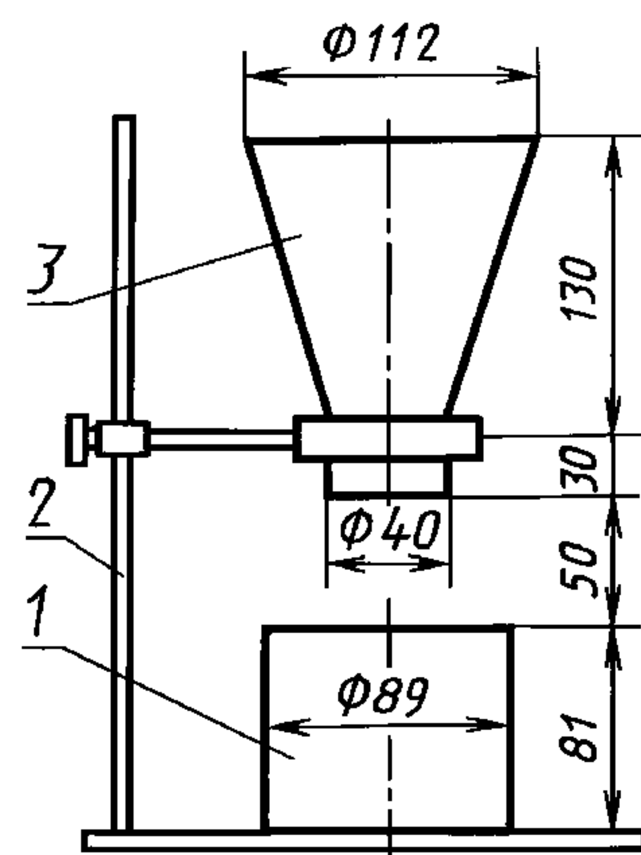
1 — измерительный цилиндр вместимостью 500 см 3 ; 2 — штатив; 3 — воронка
