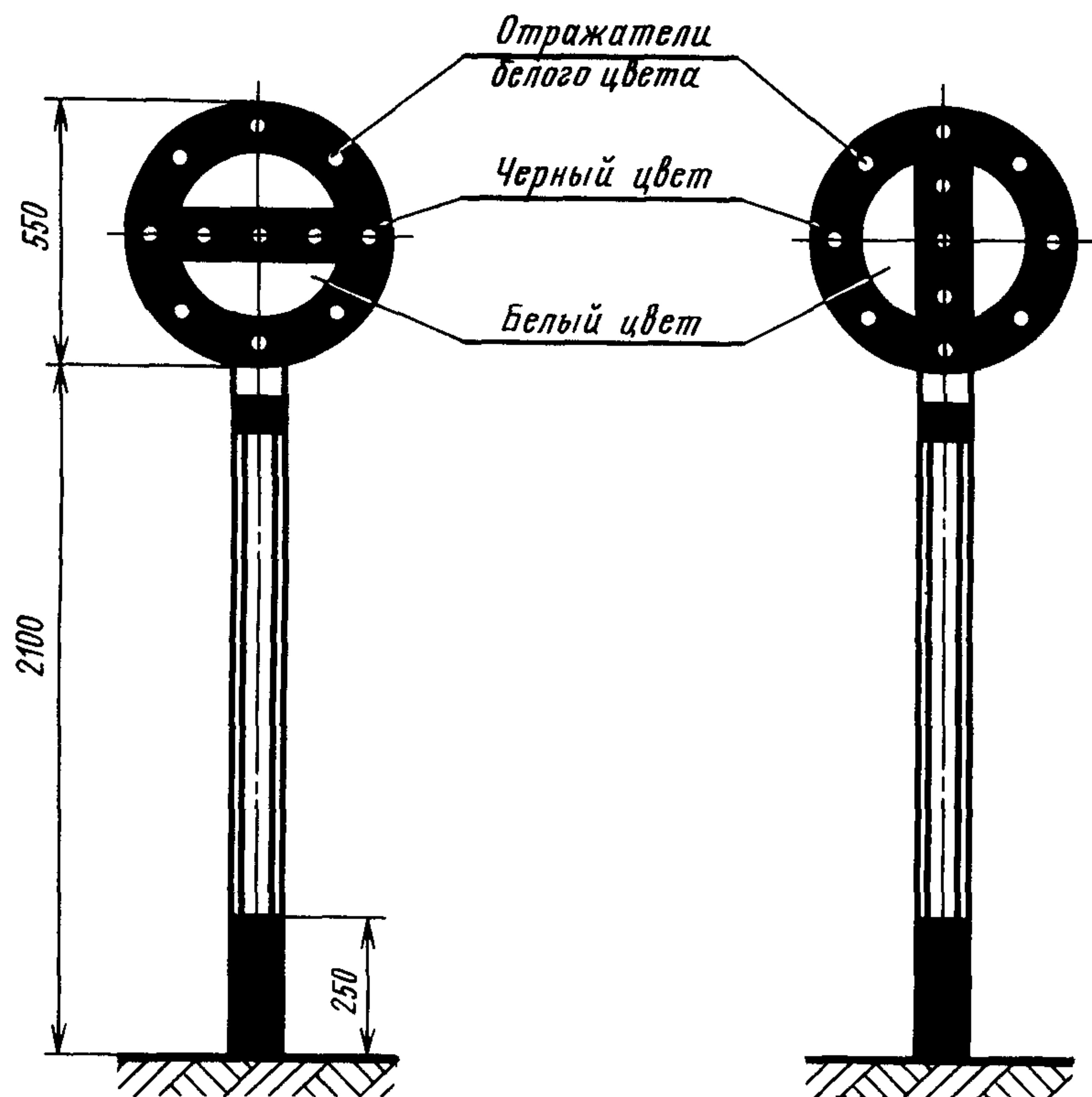
Размещение отражателей
