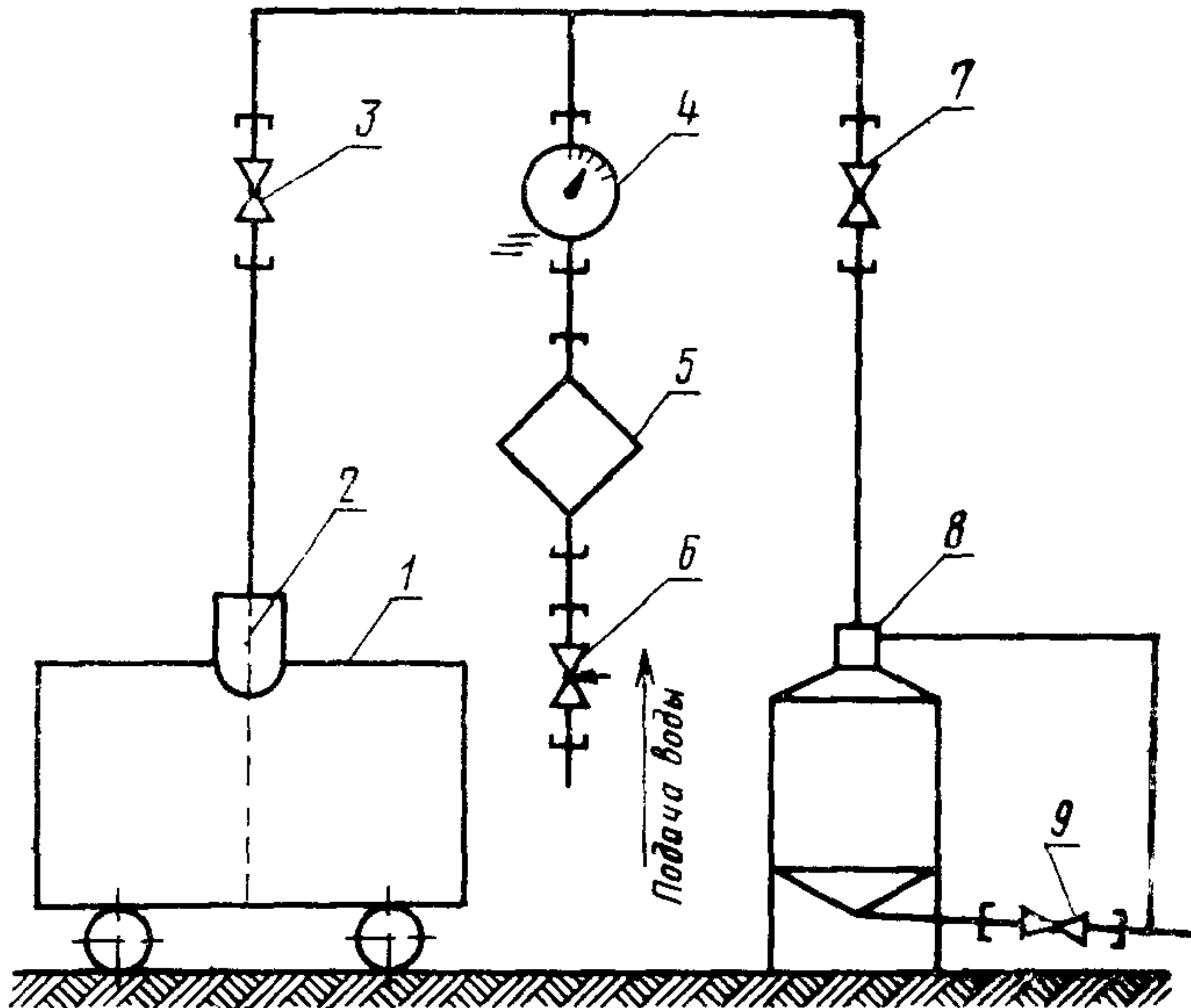
1—цистерна, 2—шланг, 3 6, 7, 9—краны, 4—счетчик жидкости, 5—фильтр; 8—мерник
