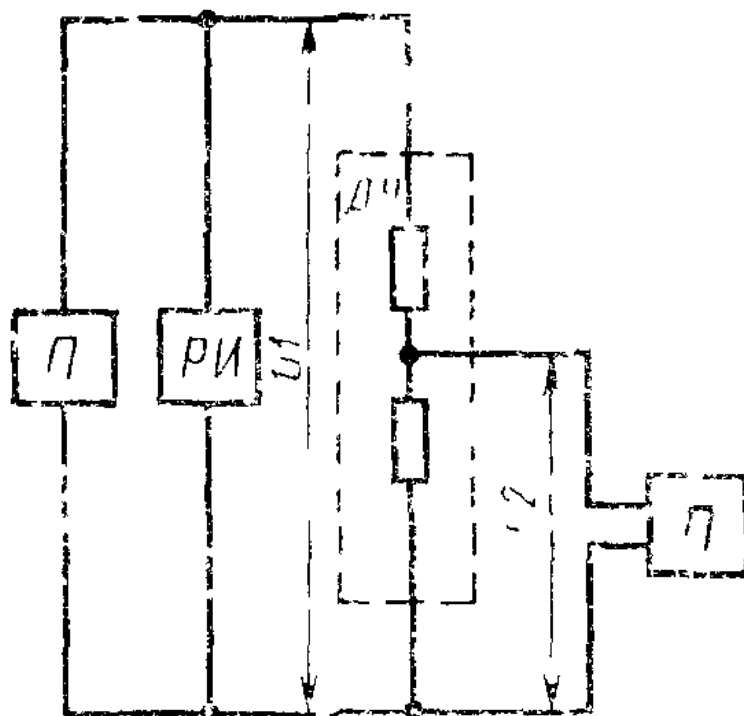
Схема измерения регулируемым источником постоянного напряжения
