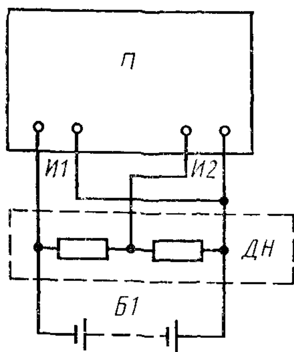
ДН—делитель напряжения Черт. 3
