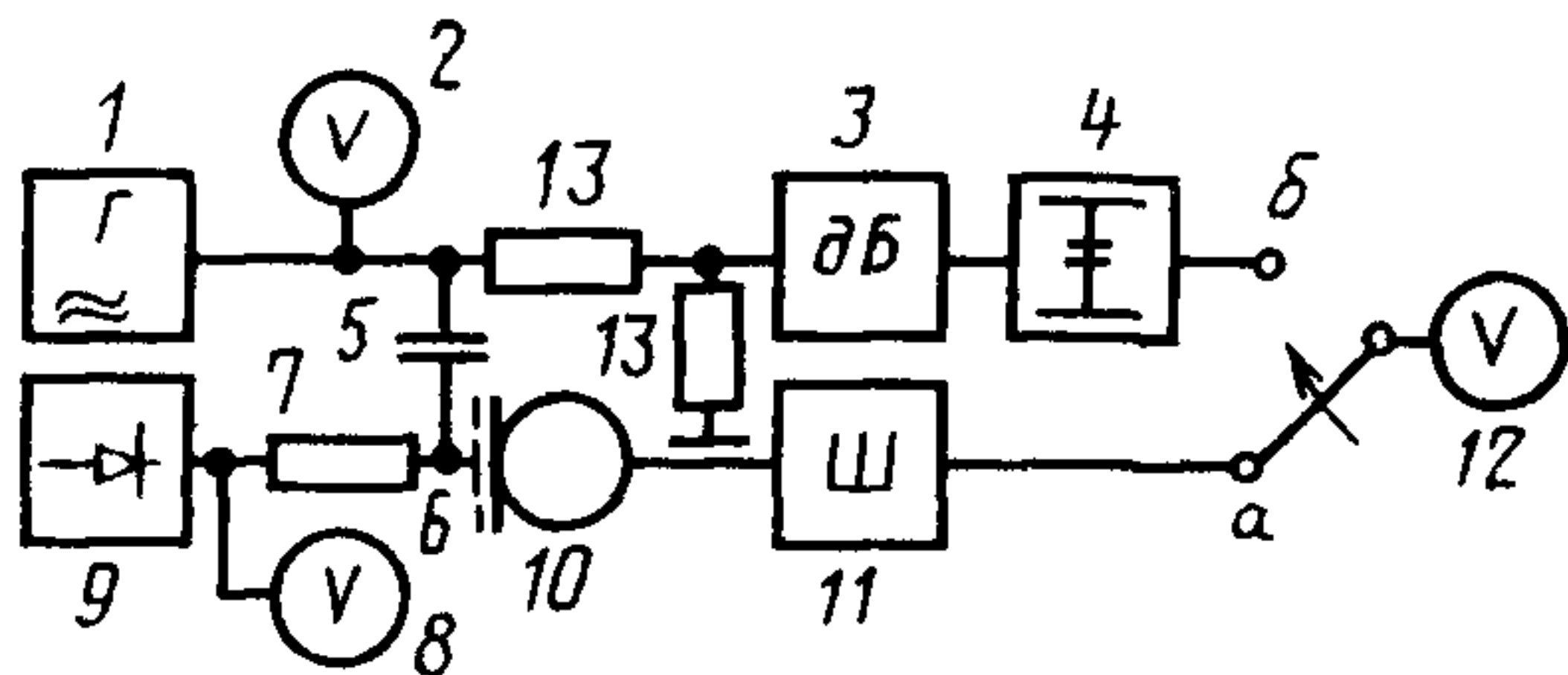
1—генератор; 2, 8—вольтметры; 3—магазин затуханий; 4—согласующее звено; 5—разделительный конденсатор; 6—электростатический возбудитель; 7—резистор; 9—источник поляризующего напряжения; 10—микрофон шумомера; 11—электрическая часть шумомера; 12—вольтметр или самописец; 13—делитель напряжения
