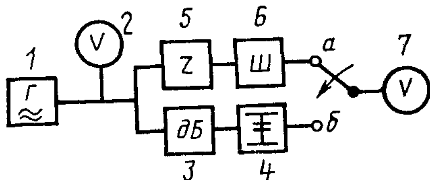
1—генератор; 2—вольтметр; 3—магазин затуханий; 4—согласующее звено; 5—эквивалент микрофона; 6—электрическая часть шумомера; 7—вольтметр или самописец
