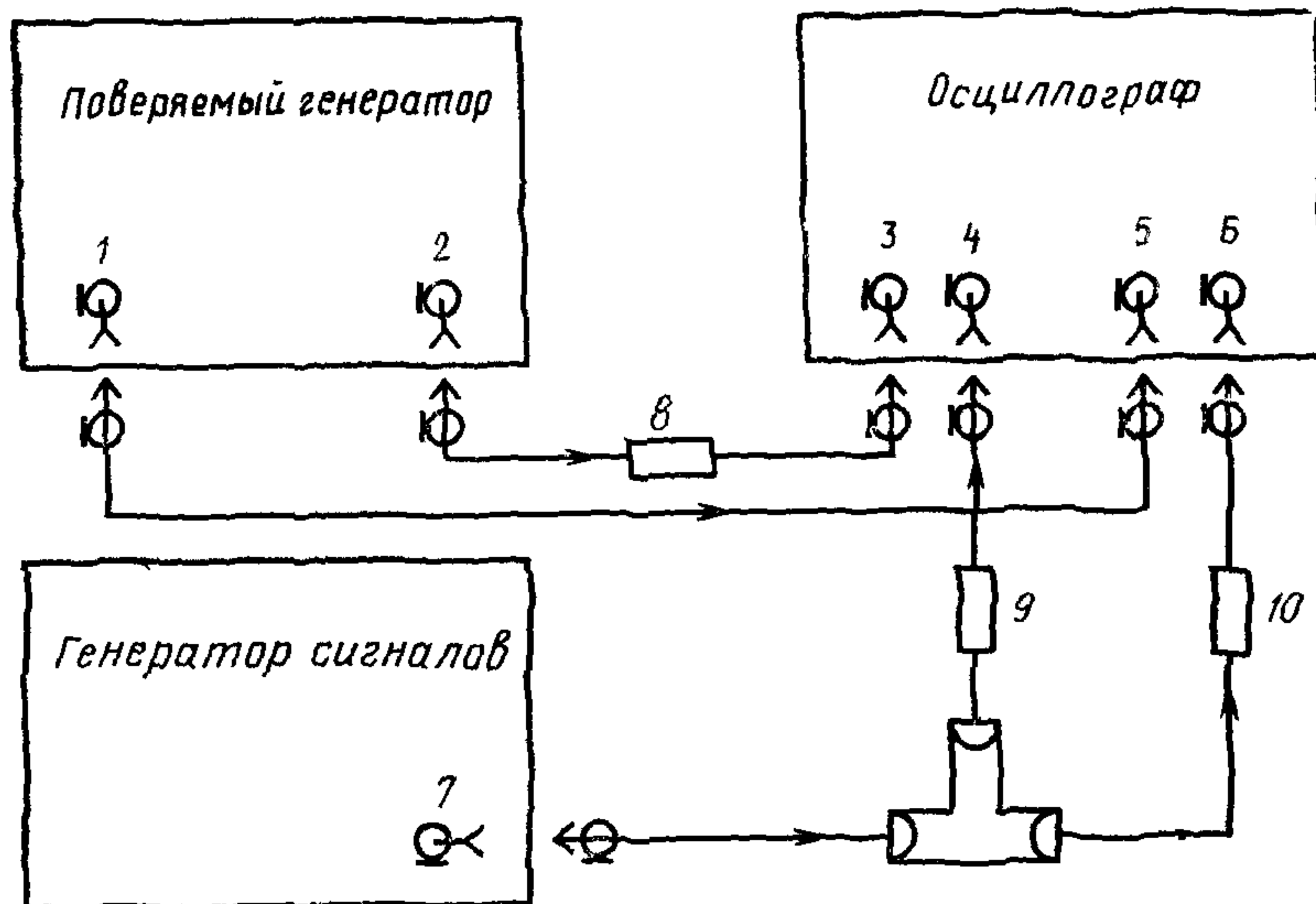
1—выход синхронизирующих импульсов, 2—выход основных импульсов, 3—вход I канала Y, 4—вход II канала Y, 5—вход низкочастотной синхронизации, 6—вход высокочастотной синхронизации, 7—выход сигнала, 8, 9, 10—аттенюаторы
