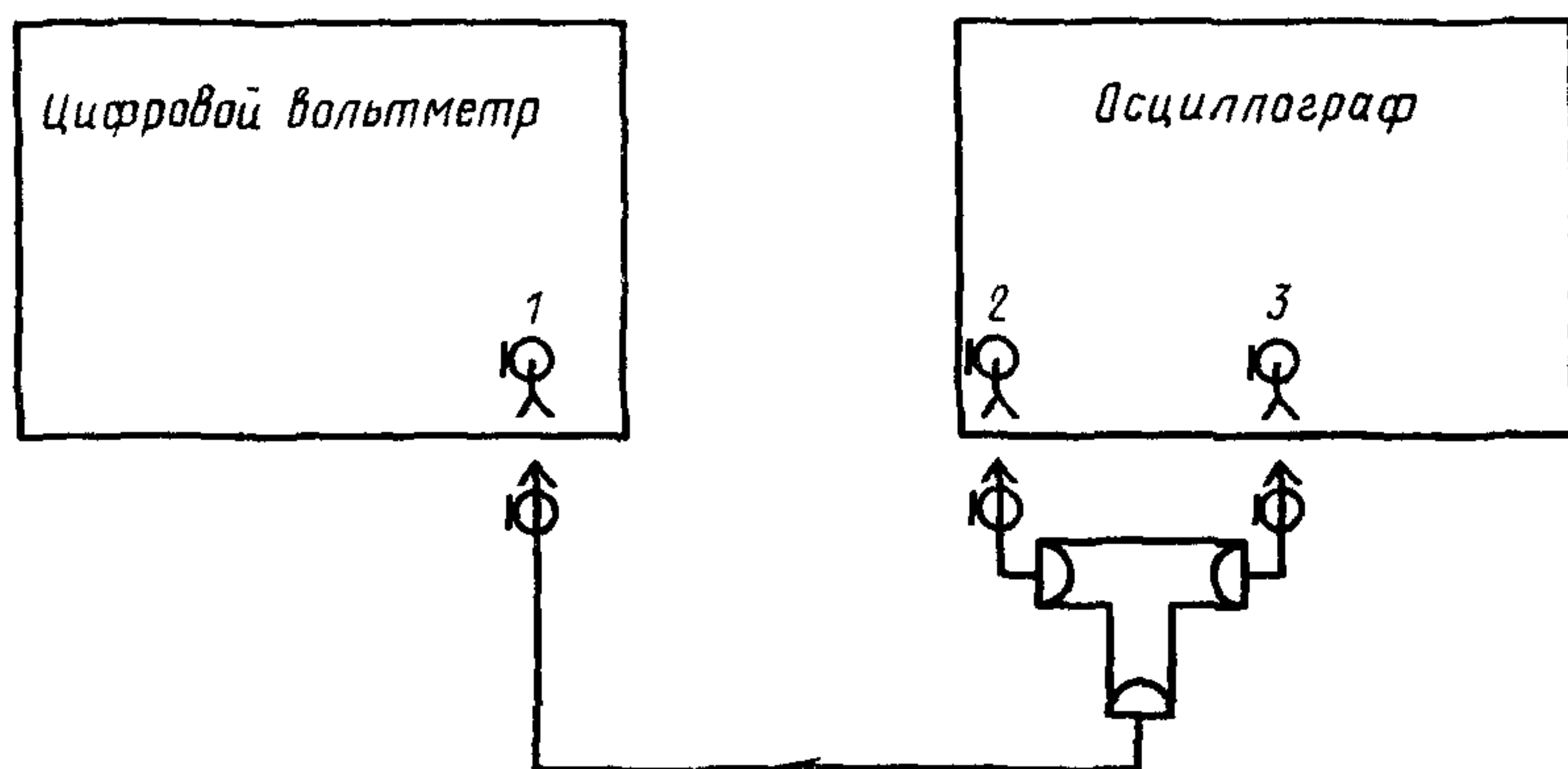
1—вход сигнала; 2—выход калибратора напряжения, 3—вход канала Y
