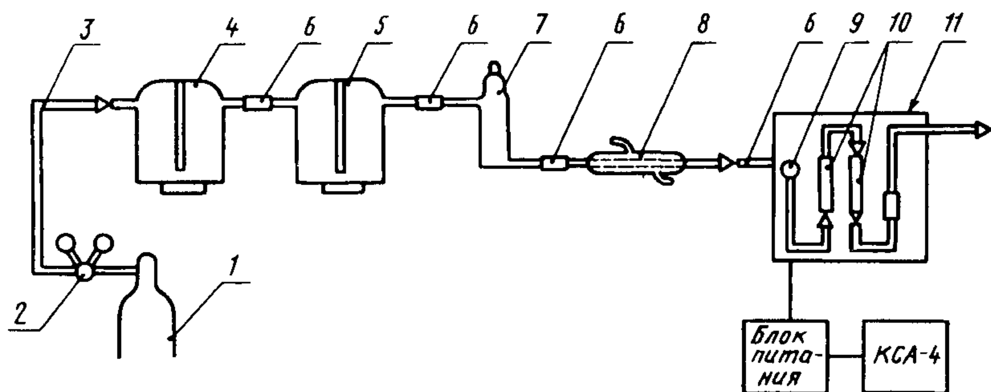
Установка для определения воды
